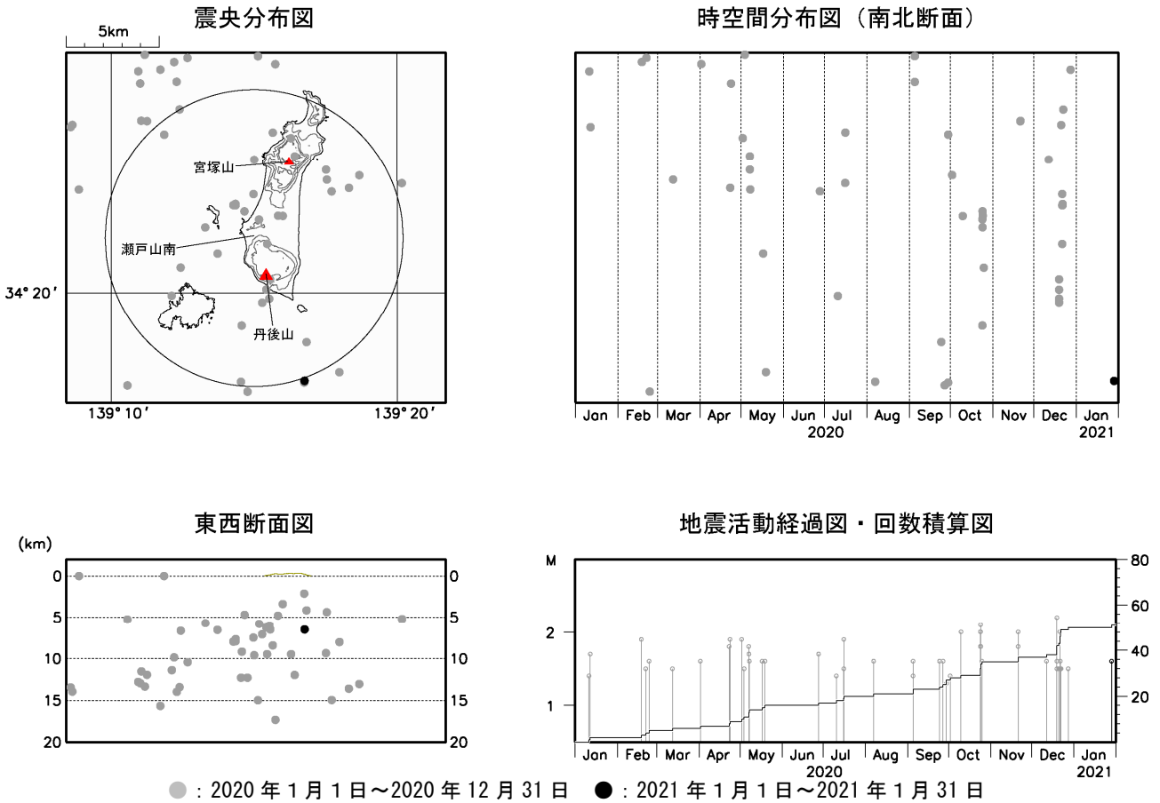
図3 新島 広域地震観測網による山体・周辺の地震活動（2020年1月1日～2021年1月31日）
