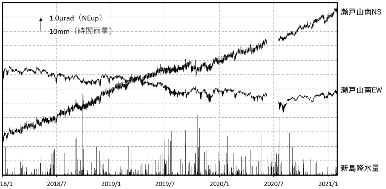
図5 新島 瀬戸山南観測点の傾斜変動（2018年1月1日～2021年1月31日） 図中の空白部分は欠測を示します。
