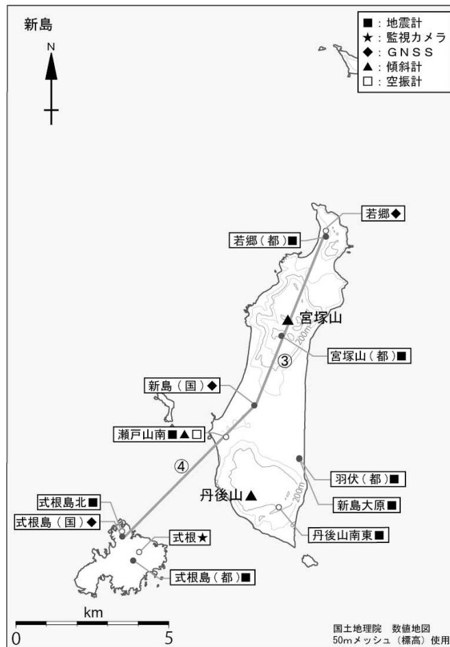
図6 新島 観測点配置図
