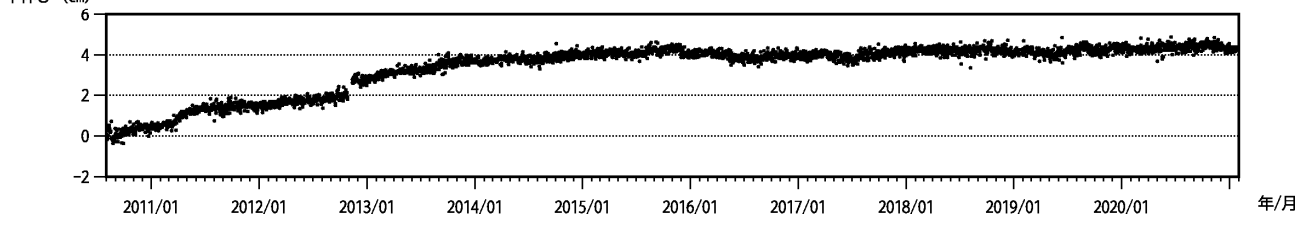
図2 新島 火山活動経過図(2010年8月2日～2021年1月31日)
