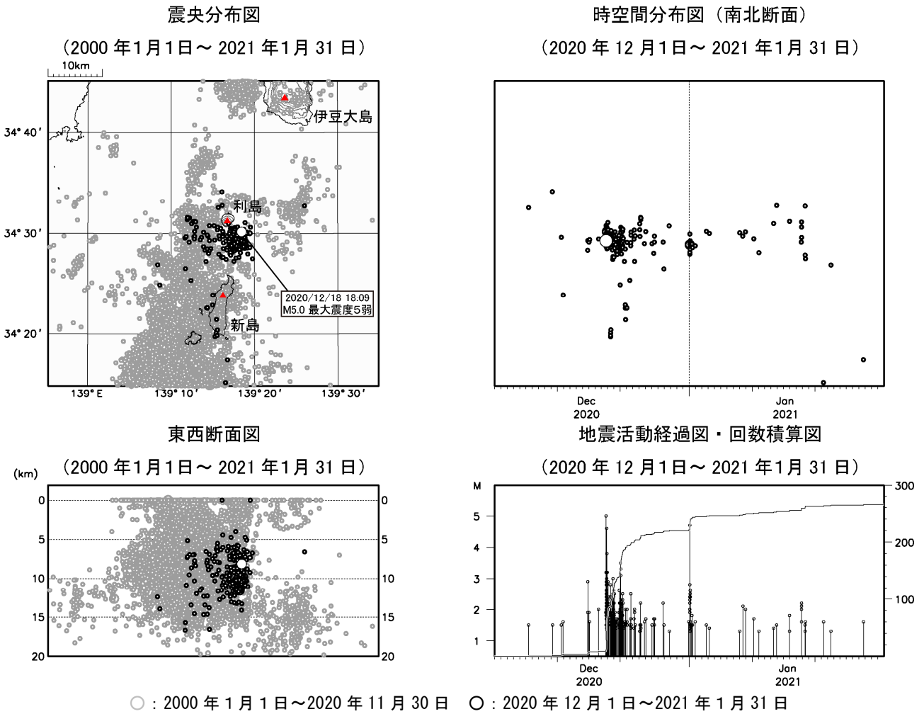
図4 新島 広域地震観測網による新島・利島周辺の地震活動 (2000年1月1日～2021年1月31日)
