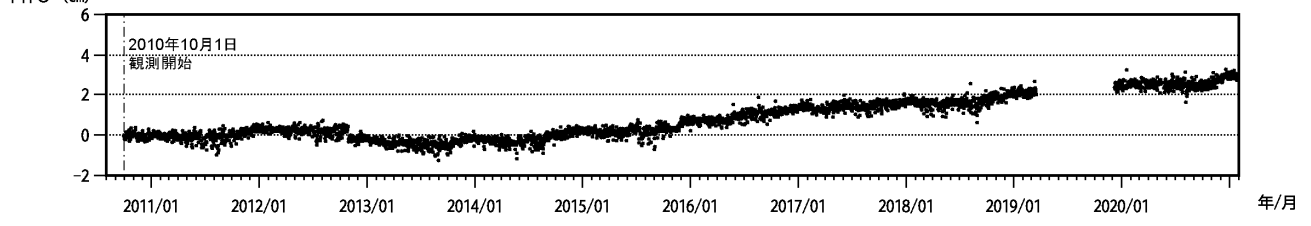
④ GNSS観測 式根島(国)-新島(国) (基線長 6092m)
