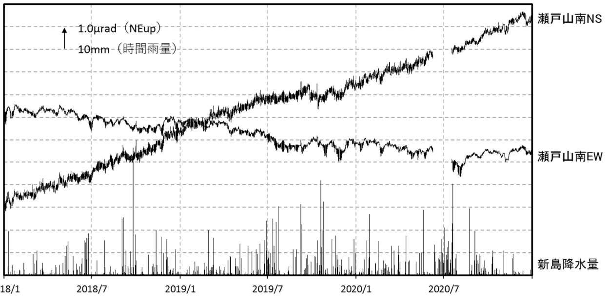
図5 新島 瀬戸山南観測点の傾斜変動（2018年1月1日～2020年12月31日） 図中の空白部分は欠測を示します。
