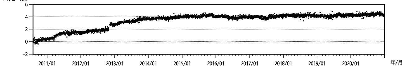
図2 新島 火山活動経過図(2010年8月2日～2020年12月31日)
