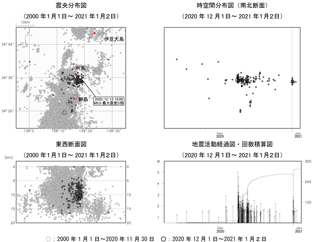
図4 新島 広域地震観測網による新島・利島周辺の地震活動 (2000年1月1日～2021年1月2日)
