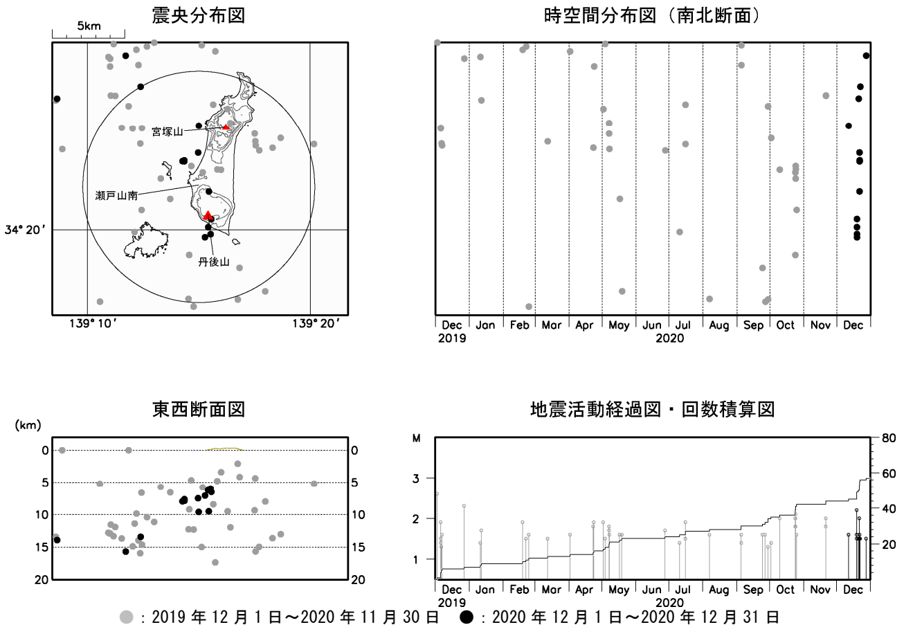
図3 新島 広域地震観測網による山体・周辺の地震活動（2019年12月1日～2020年12月31日） 広域地震観測網により震源決定したもので、深さは全て海面以下として決定しています。 M（マグニチュード）は地震の規模を表し、M1.3以上の地震を示しています。 図中の震源要素は一部暫定値が含まれており、後日変更することがあります。 計数対象（瀬戸山南から半径約8km、深さ約20km以内）以外の地震が含まれるため、図2-①の日別A型地震回数とは異なります。 震央分布図中の円は火山性地震の回数の計数対象（瀬戸山南から半径8km、深さ20km以内）の範囲を示しています。 この図では、関係機関の地震波形を一元的に処理し、地震観測点の標高を考慮する等した新手法で得られた震源を用いています（ただし、2020年8月以前の地震については火山活動評価のための参考震源です）。 2021年1月12日現在、2020年4月18日から10月23日までの地震について、暫定的に震源精査の基準を変更しているため、その前後の期間と比較して微小な地震での震源決定数の変化（増減）が見られます。
