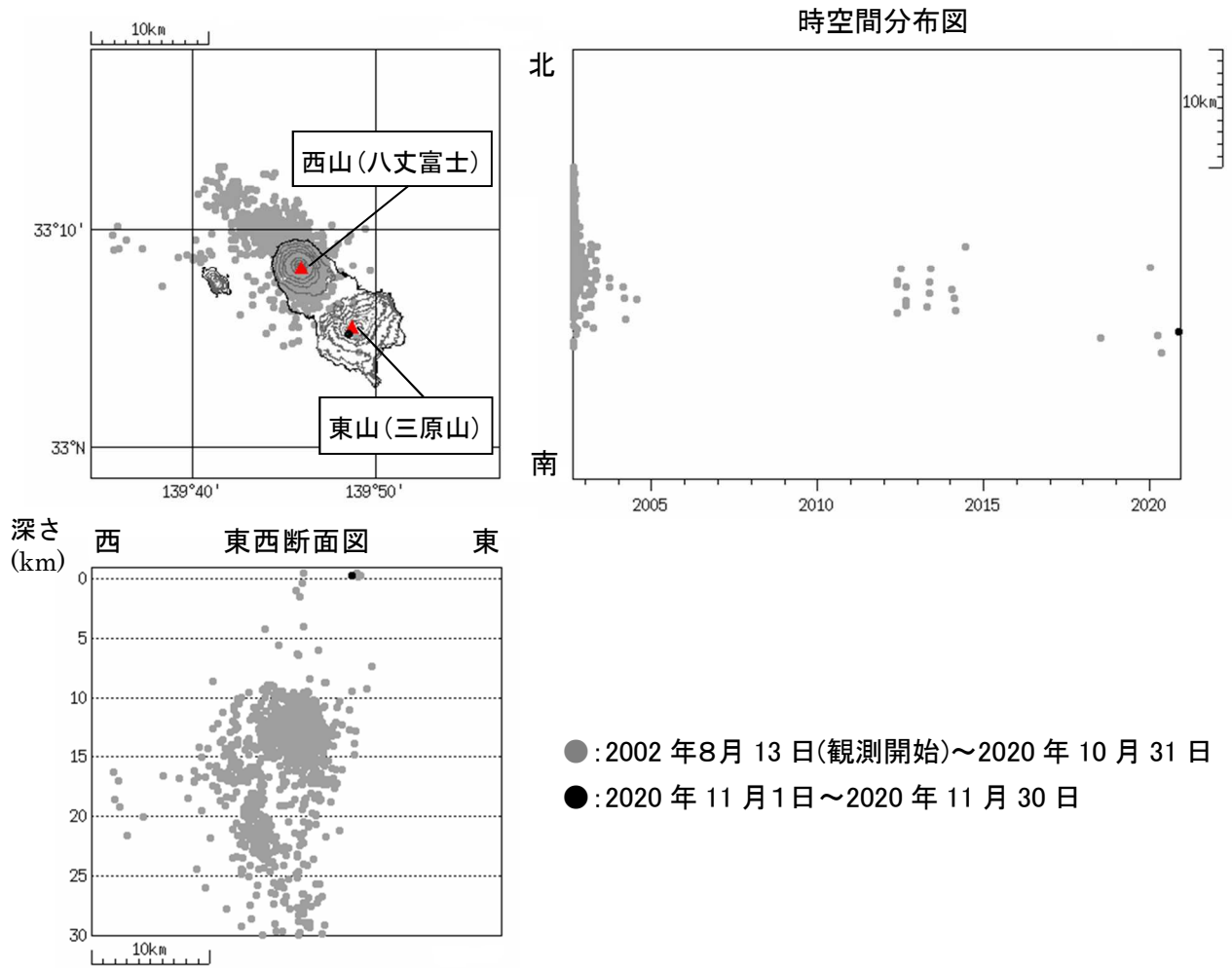
図3 八丈島 震源分布図 (2002年8月13日~2020年11月30日) 今期間発生した火山性地震の震源は、東山(三原山)直下の海拔0km付近に求まりました。
