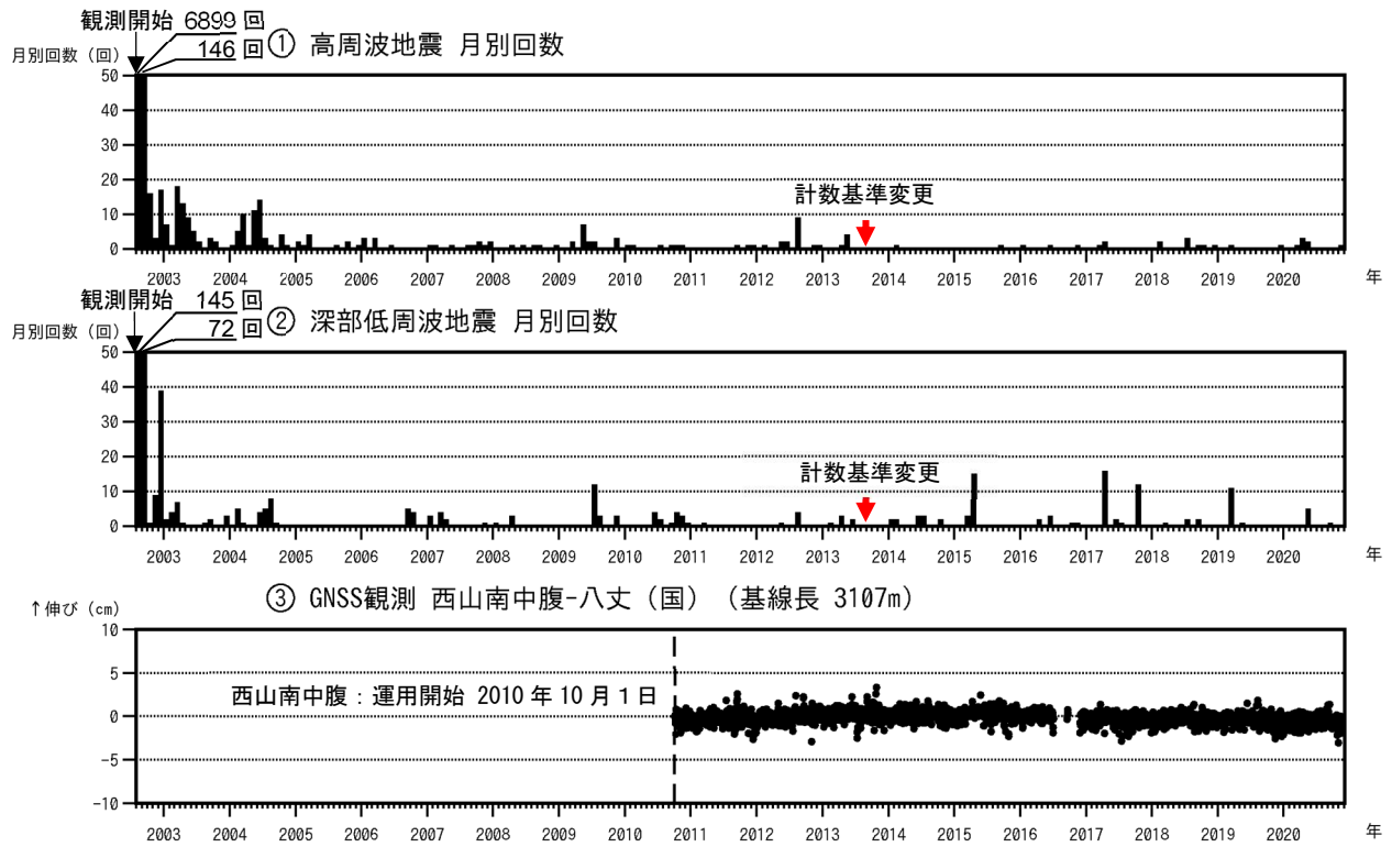
図2 八丈島 火山活動経過図（2002年8月13日～2020年11月30日）
