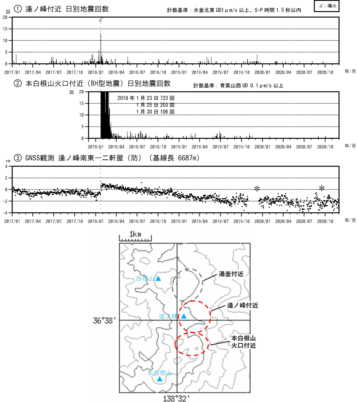
図 13 草津白根山（本白根山） 火山活動経過図（2017年1月1日～2020年11月30日）
