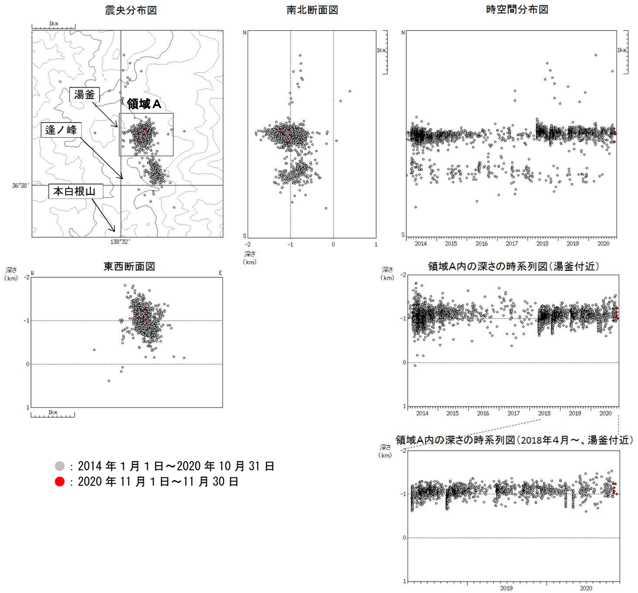
図5 草津白根山 震源分布図（2014年1月1日～2020年11月30日）
