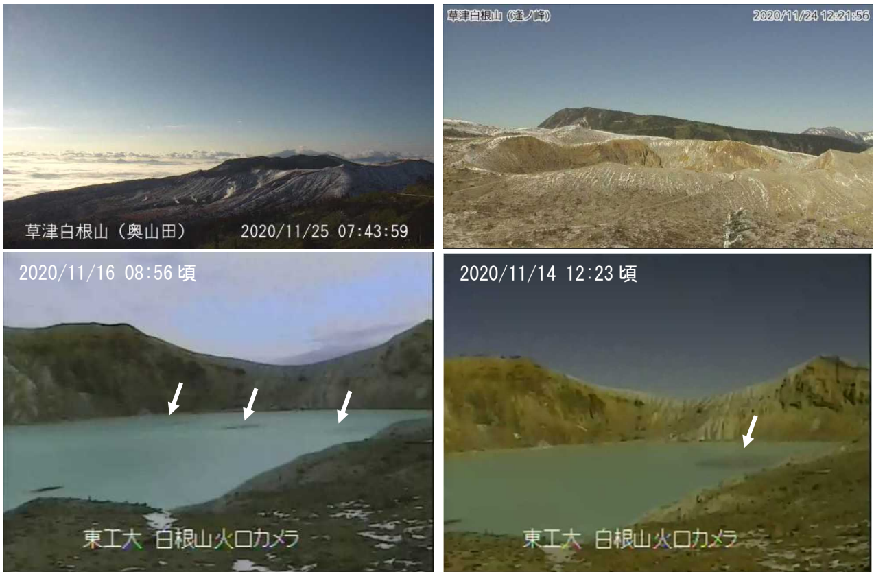
図3 草津白根山（白根山（湯釜付近）） 湯釜付近の状況
