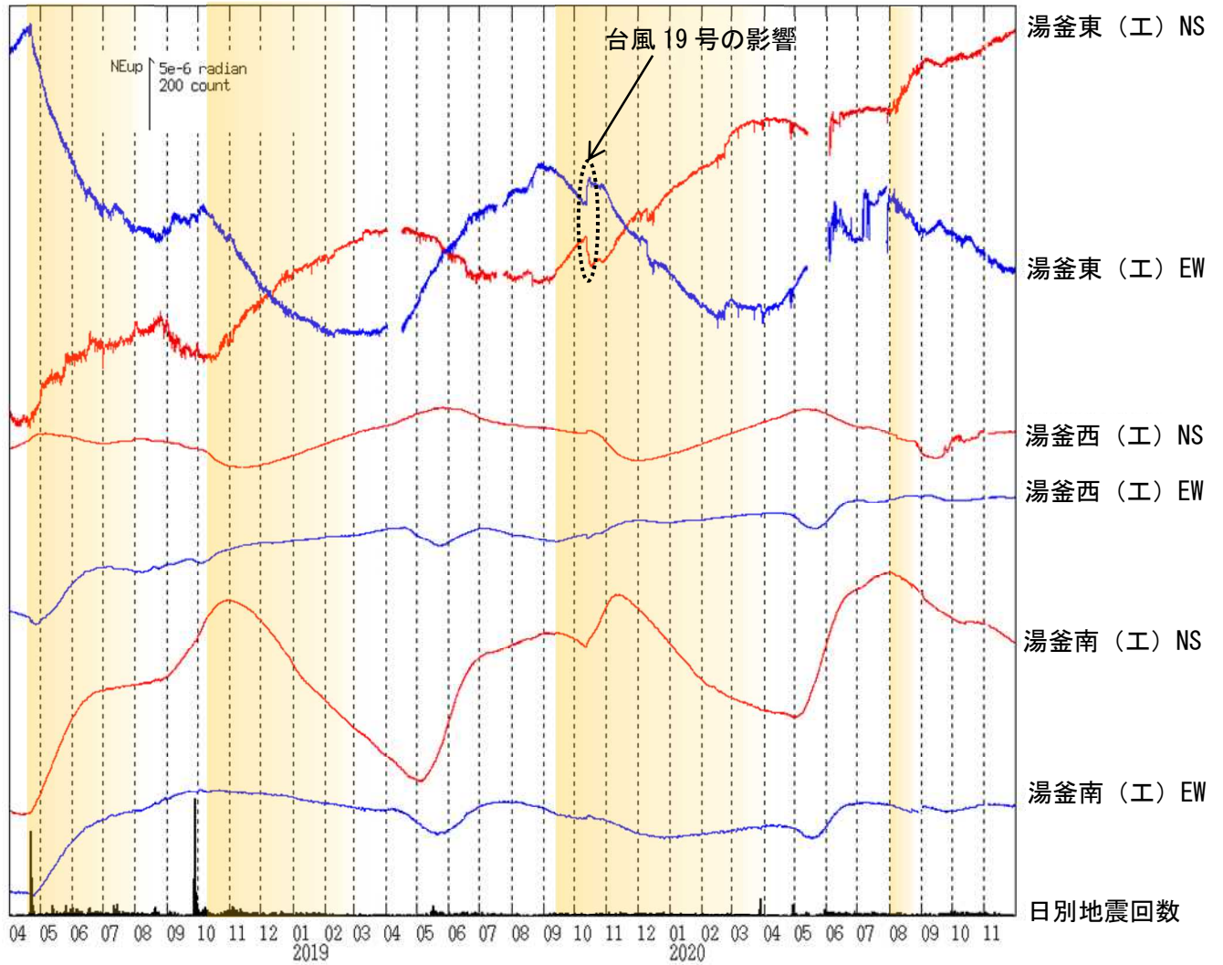
図6 草津白根山（白根山（湯釜付近）） 傾斜変動（2018年4月1日～2020年11月30日）
