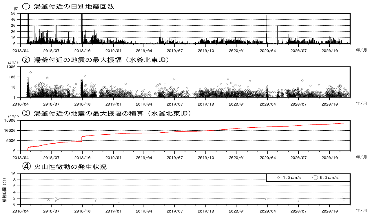
図2 草津白根山（白根山（湯釜付近）） 湯釜付近の地震活動及び火山性微動の発生状況（2018年4月1日～2020年11月30日）
