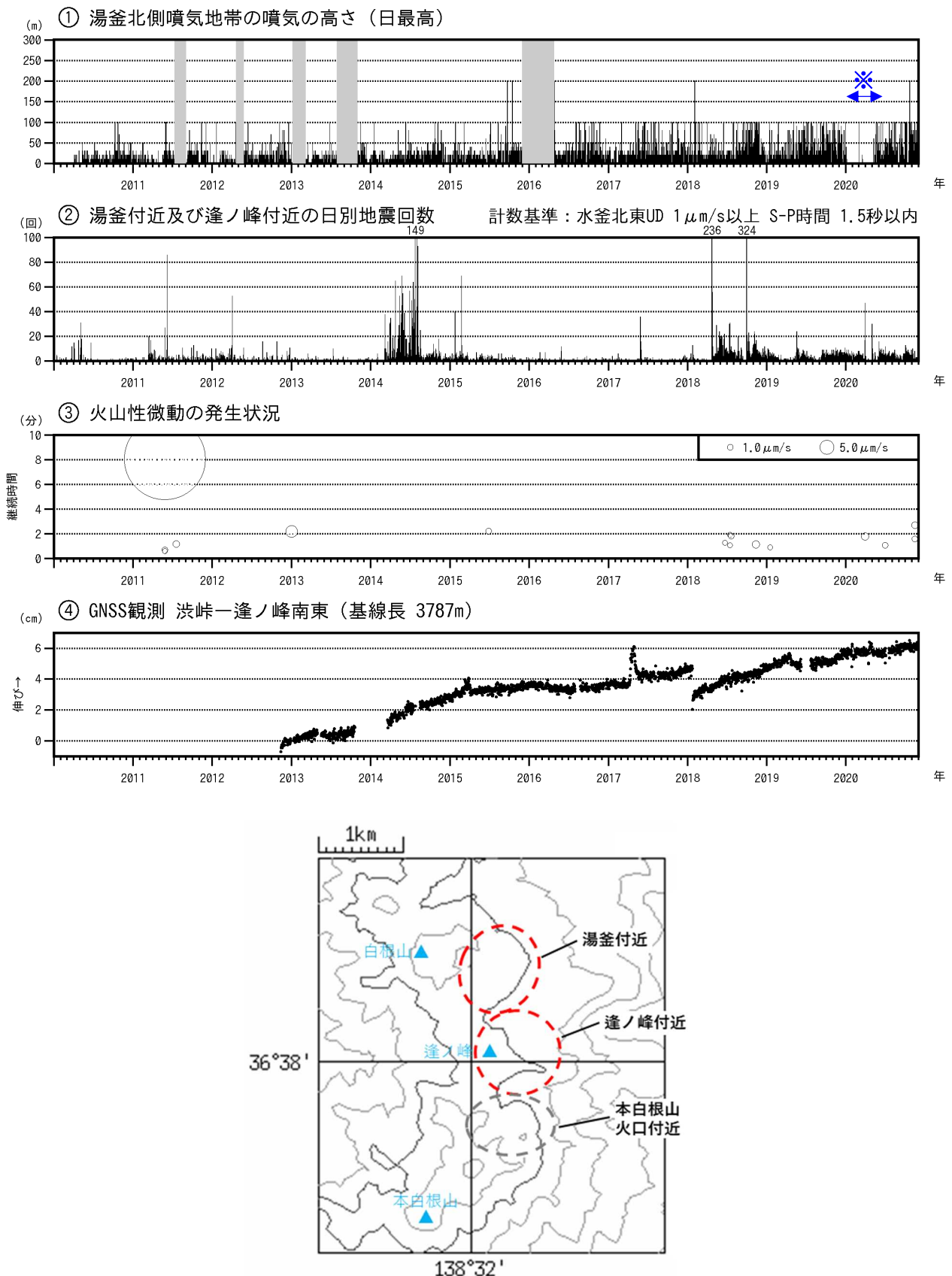
図4 草津白根山（白根山（湯釜付近））火山活動経過図（2010年1月1日～2020年11月30日）
