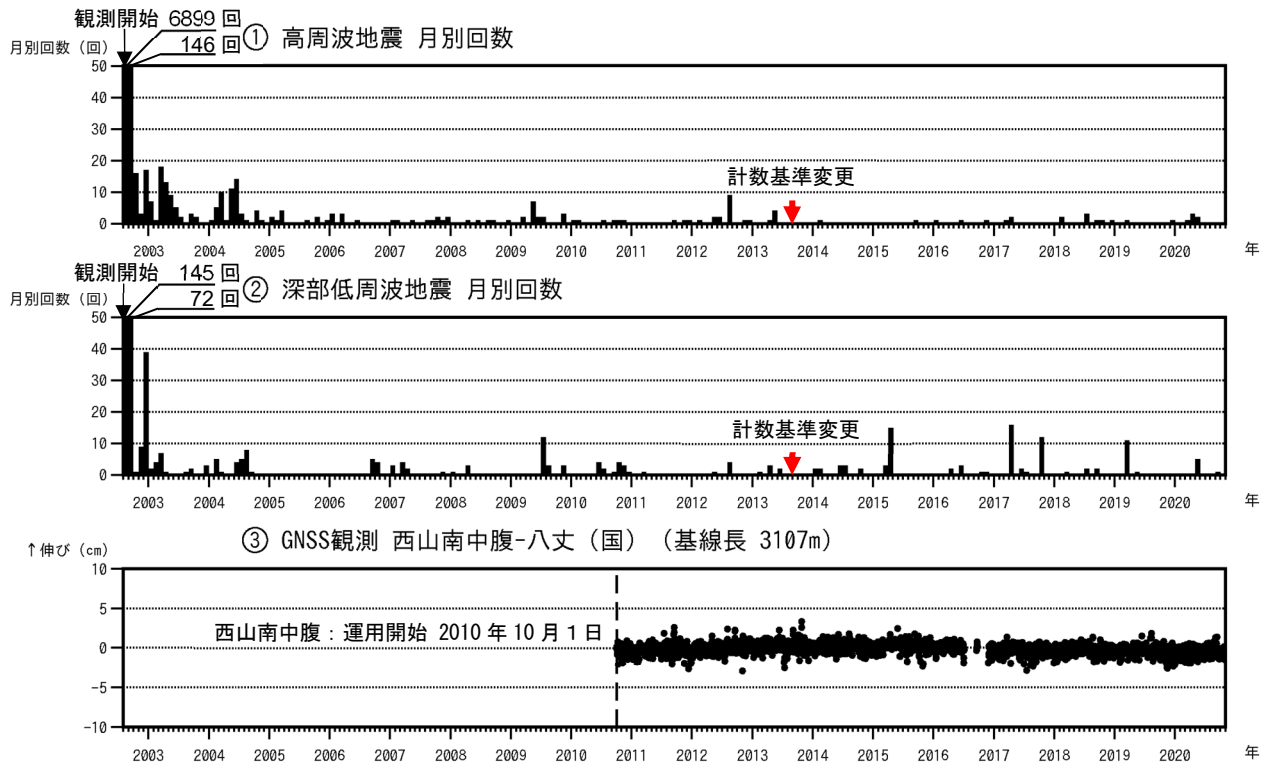
図2 八丈島 火山活動経過図（2002年8月13日～2020年10月31日）
