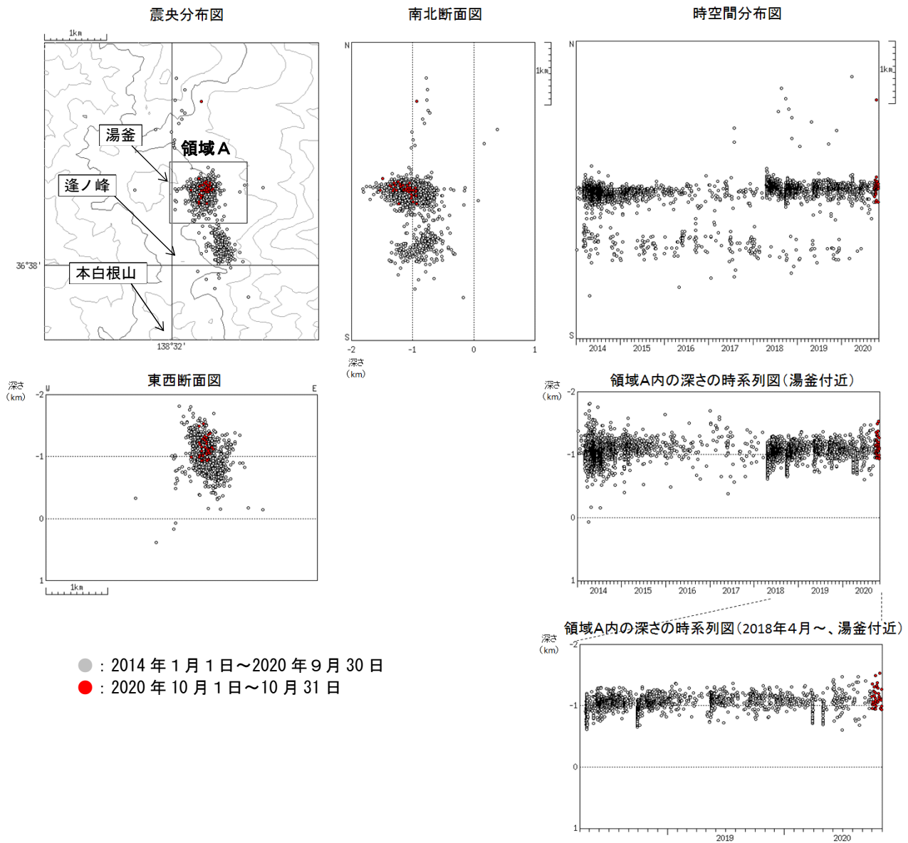
図5 草津白根山 震源分布図（2014年1月1日～2020年10月31日）
