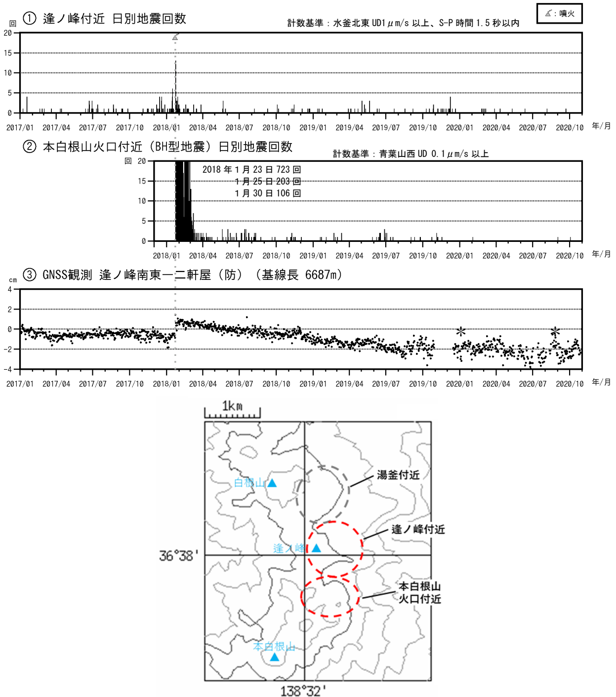
図13 草津白根山（本白根山） 火山活動経過図（2017年1月1日～2020年10月31日）
