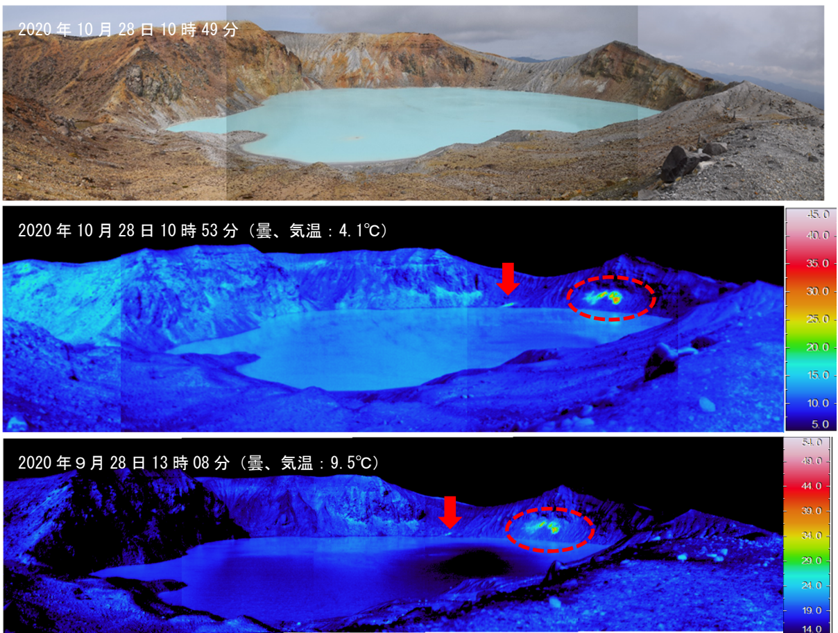
図1-1 草津白根山(白根山(湯釜付近)) 湯釜火口内の状況
