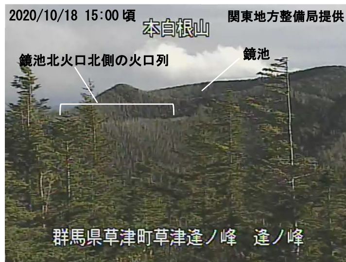
図12 草津白根山（本白根山） 本白根山付近の状況（10月18日逢ノ峰監視カメラ）
