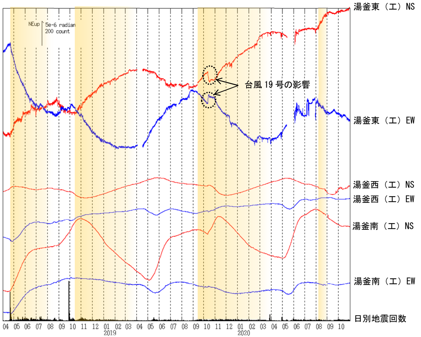
図6 草津白根山（白根山（湯釜付近）） 傾斜変動（2018年4月1日～2020年10月31日）
