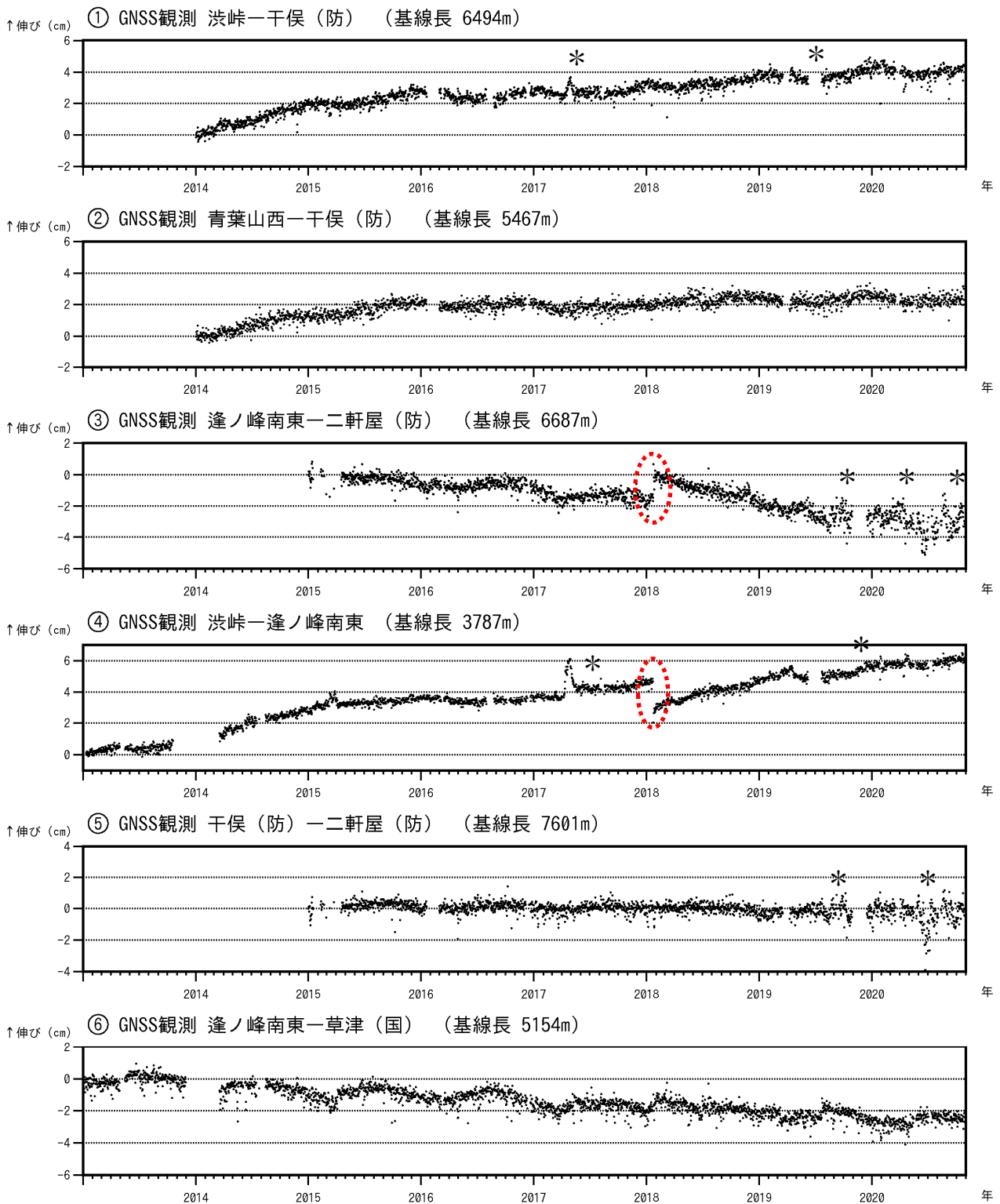
図7 草津白根山 GNSS連続観測の結果 (2013年1月1日～2020年10月31日)
