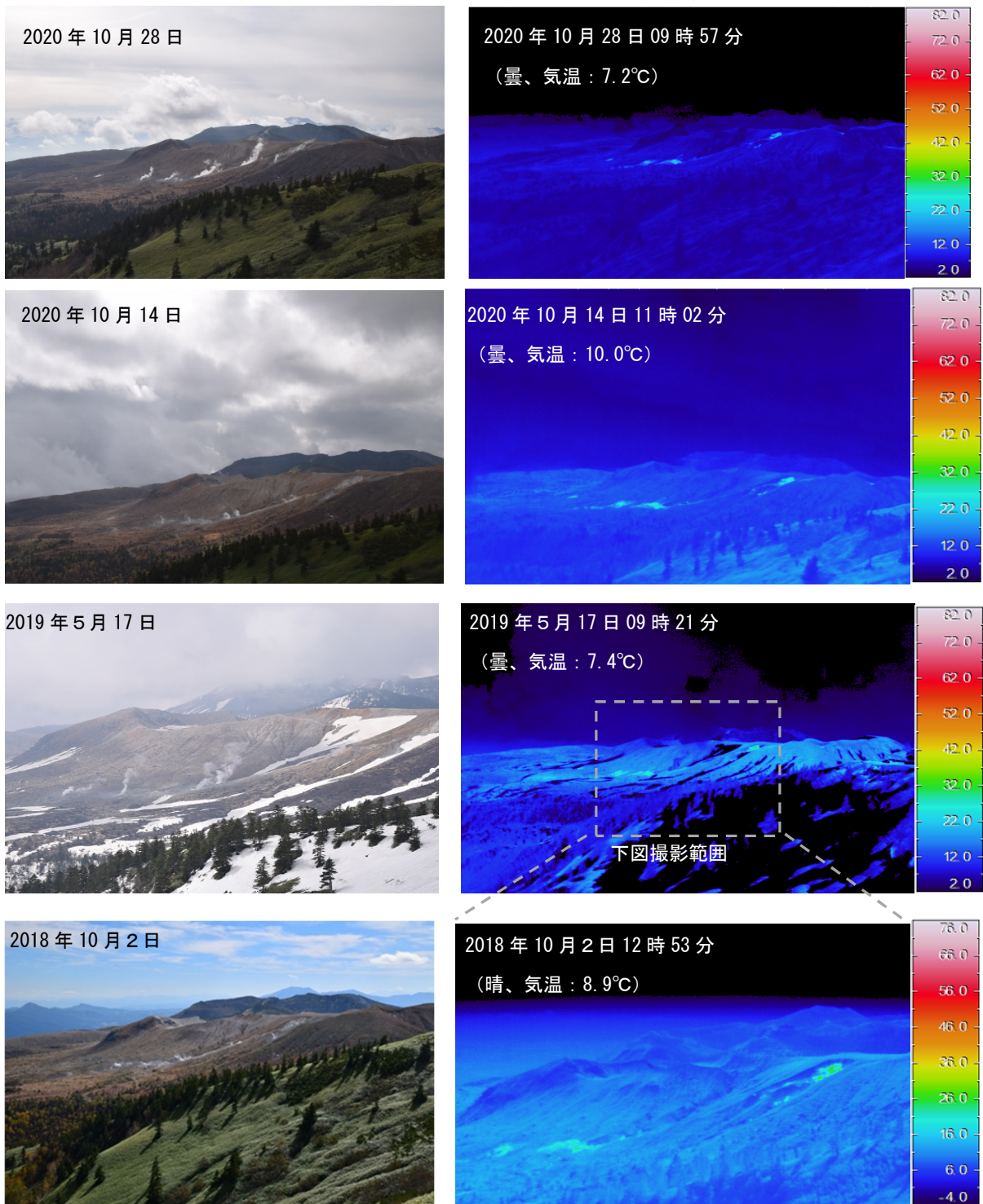
図1-3 草津白根山（白根山（湯釜付近）） 湯釜火口北側噴気地帯の状況
