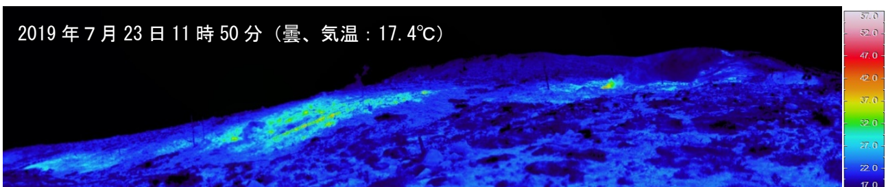
図1 - 4 草津白根山（白根山（湯釜付近）） 湯釜火口北側噴気地帯の状況
