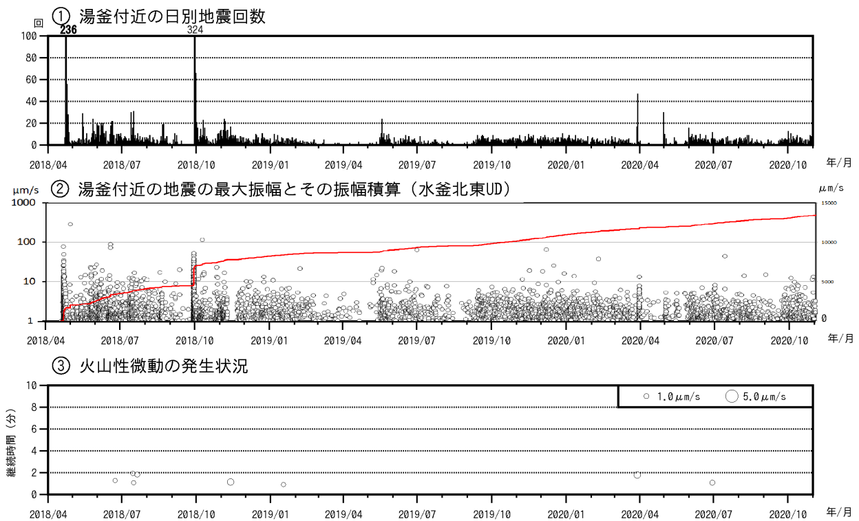
図2 草津白根山（白根山（湯釜付近）） 湯釜付近の地震活動及び火山性微動の発生状況 （2018年4月1日～2020年10月31日）（中段○：最大振幅（左軸）、赤線：最大振幅の積算（右軸）） ・湯釜付近を震源とする火山性地震は、やや多い状態で経過しました。 ・火山性微動は、6月30日以降観測されていません。
