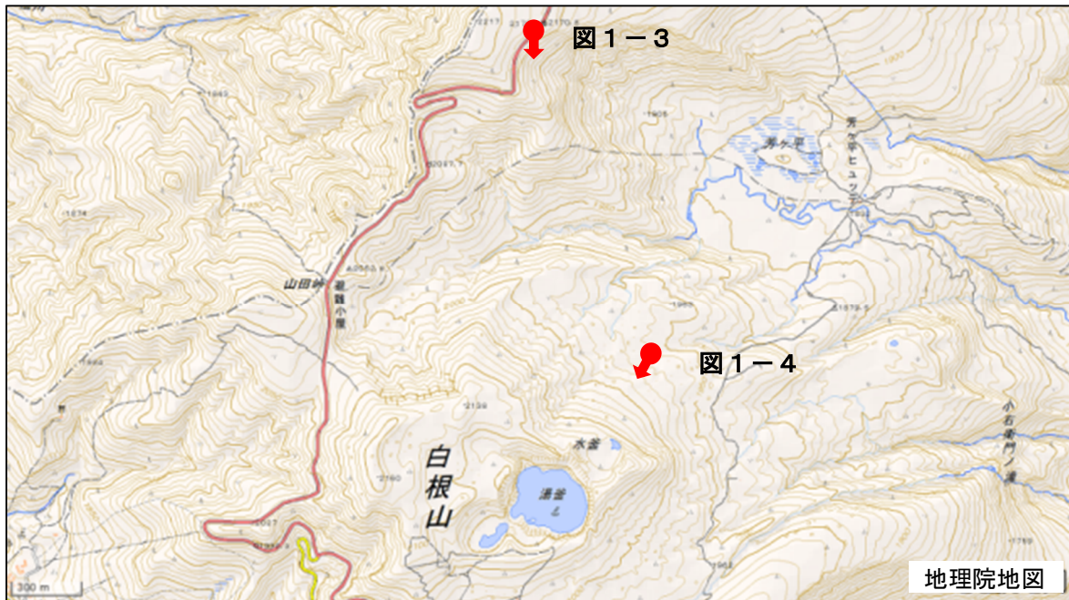
図1-5 草津白根山（白根山（湯釜付近）） 写真撮影位置と撮影方向 ・赤丸及び赤矢印は、図1-3、図1-4の撮影位置と撮影方向を示します。
