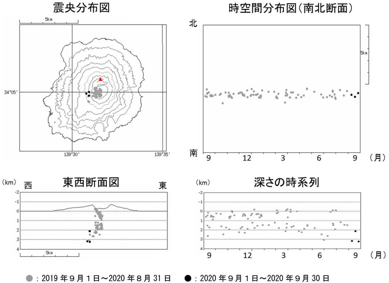
図8 三宅島 震源分布図（2019年9月1日～2020年9月30日）
