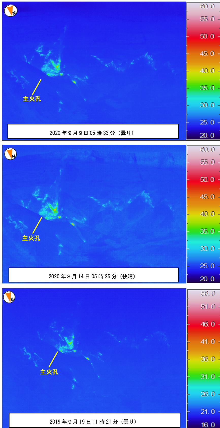
図4 三宅島 赤外熱映像装置による山頂火口内の地表面温度分布 9日に実施した機動観測では、8月や昨年と同様に主火孔内及びその周辺で引き続き高温領域が認められました。高温領域の分布に特段の変化は認められません。
