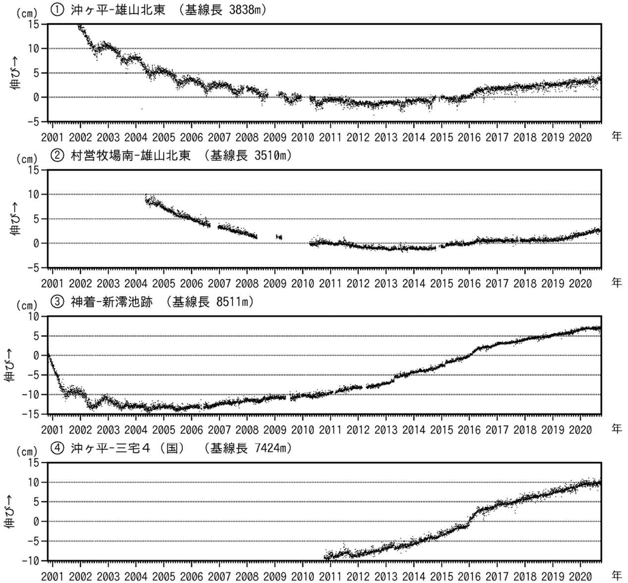
図7 三宅島 GNSS 連続観測結果（2000年10月26日～2020年9月30日）
