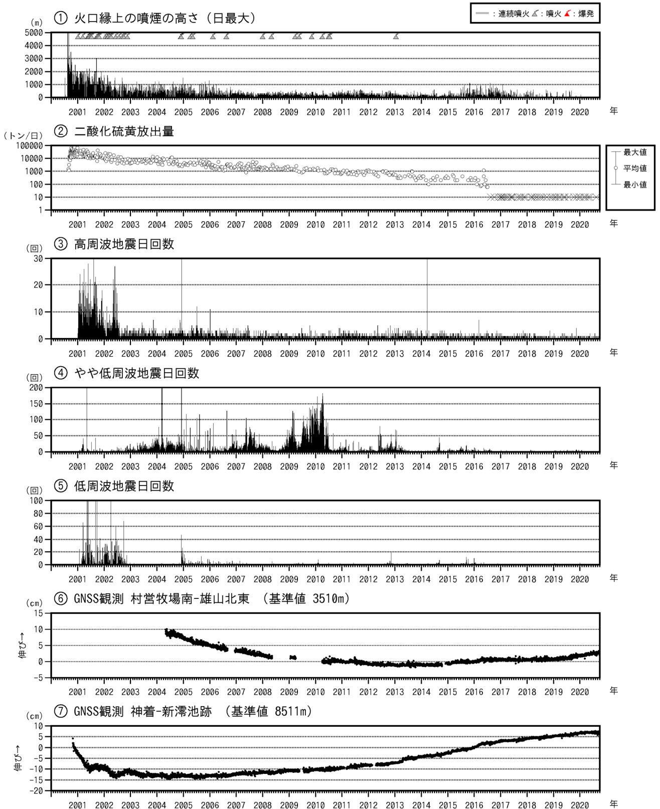
図5 三宅島 火山活動長期経過図（2000年1月1日～2020年9月30日）
