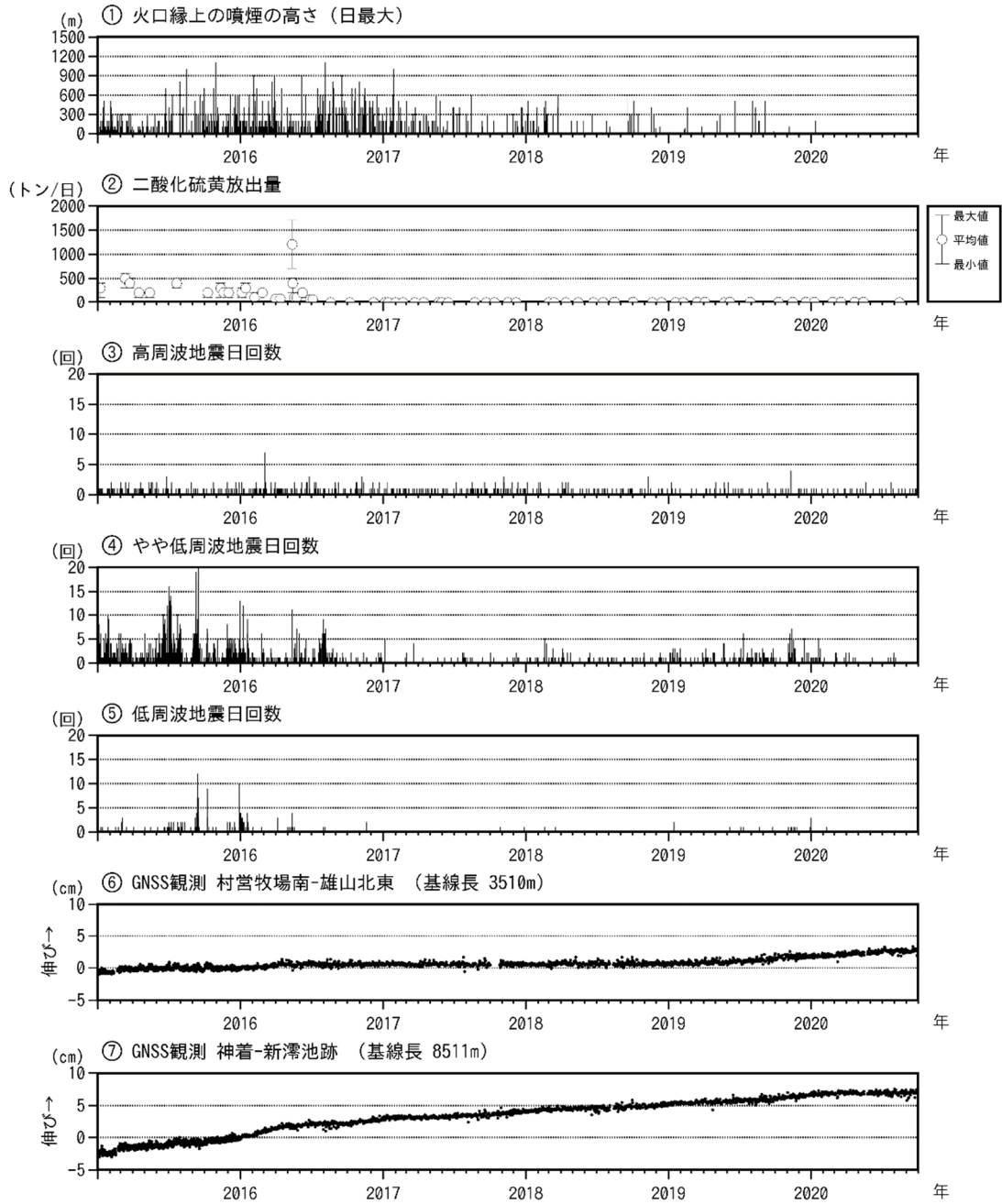
図6 三宅島 火山活動短期経過図（2015年1月1日～2020年9月30日）
