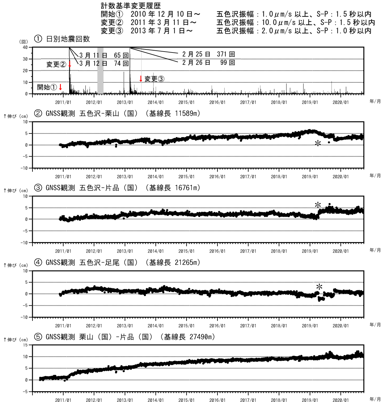
図2 日光白根山 火山活動経過図（2010年4月1日～2020年9月30日）
