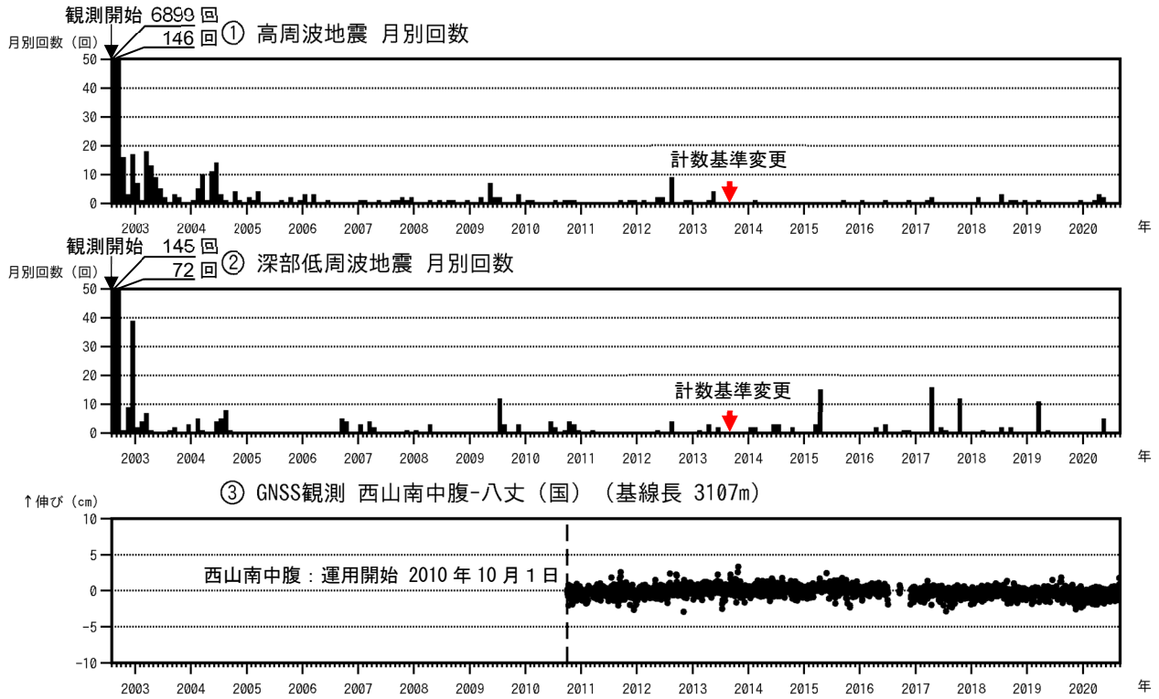
図2 八丈島 火山活動経過図（2002年8月13日～2020年8月31日）
