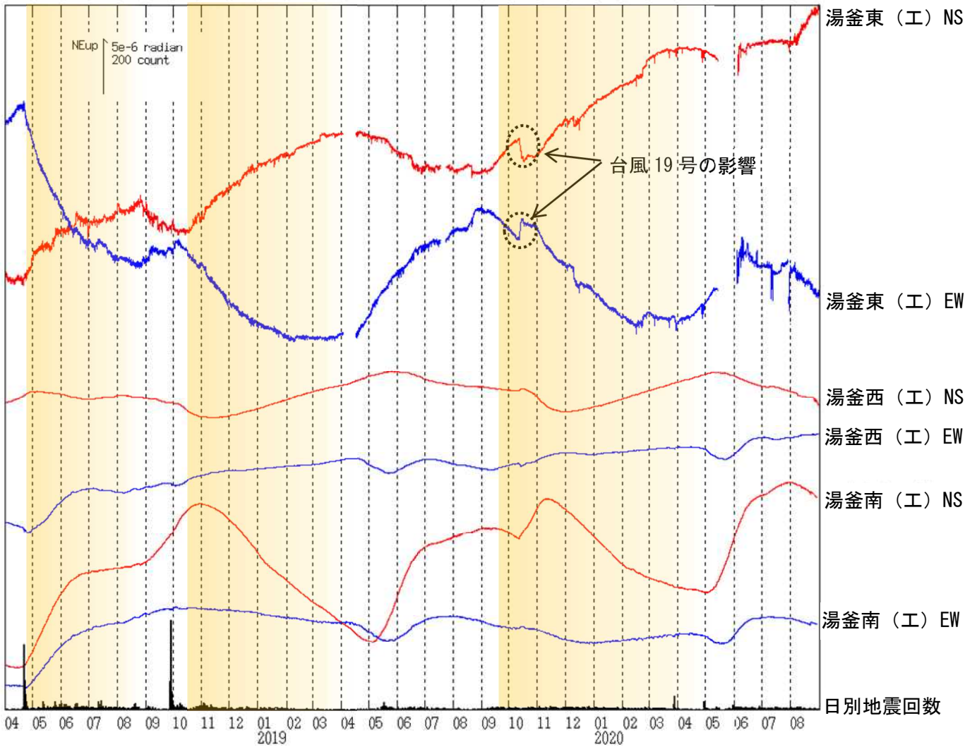
図6 草津白根山（白根山（湯釜付近）） 傾斜変動（2018年4月1日～2020年8月31日）
