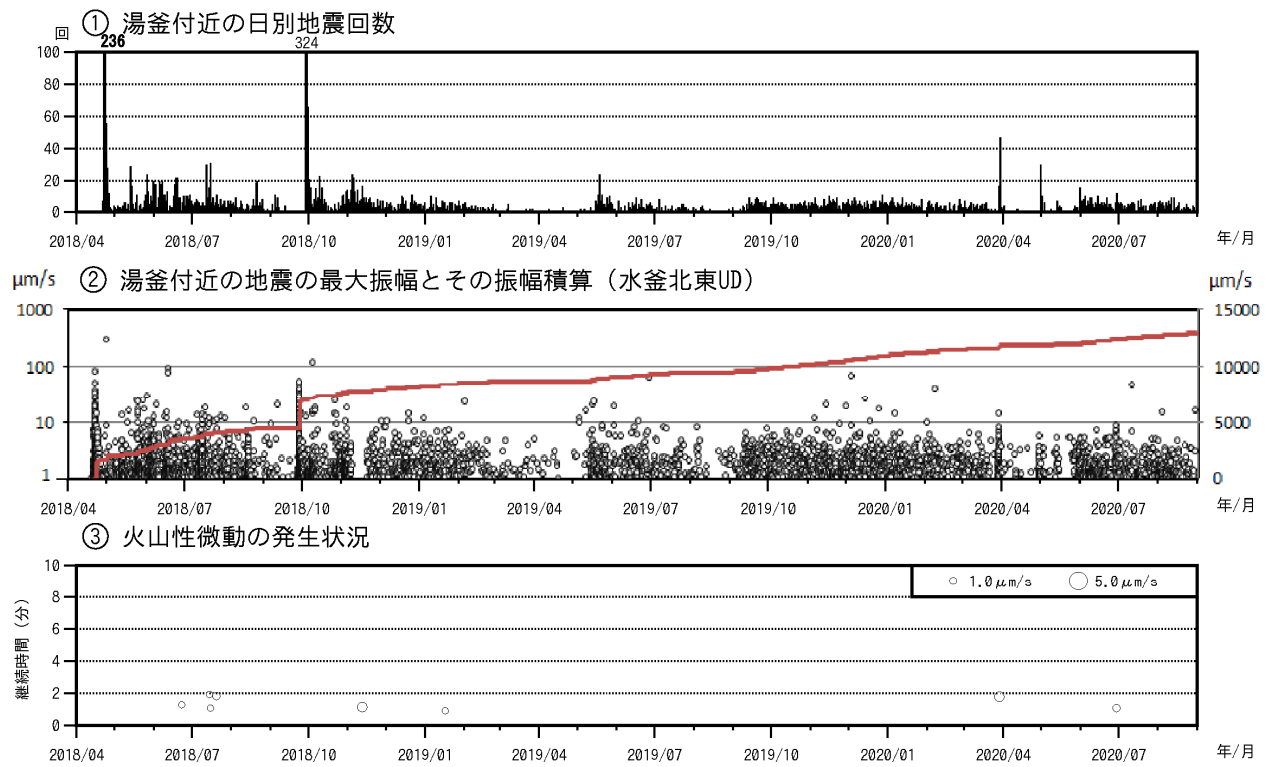
図2 草津白根山（白根山（湯釜付近）） 湯釜付近の地震活動及び火山性微動の発生状況（2018年4月1日～2020年8月31日）（中段 ○：最大振幅（左軸）、赤線：最大振幅の積算（右軸）） ・湯釜付近を震源とする火山性地震は、やや多い状態で経過しました。
