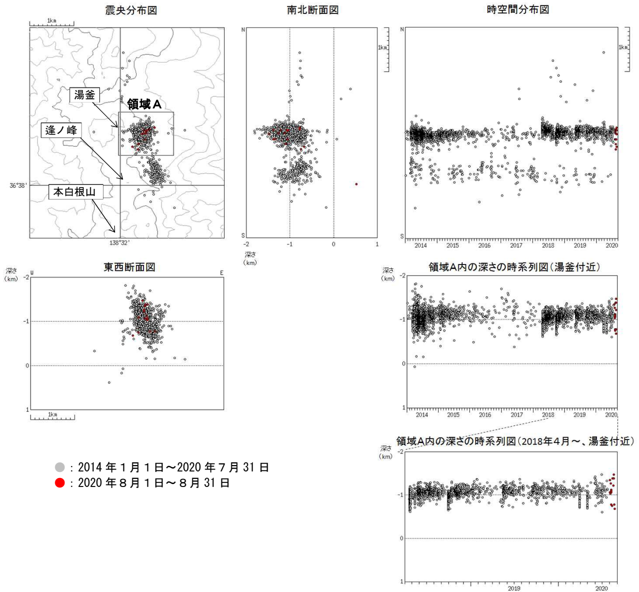
図5 草津白根山 震源分布図（2014年1月1日～2020年8月31日）
