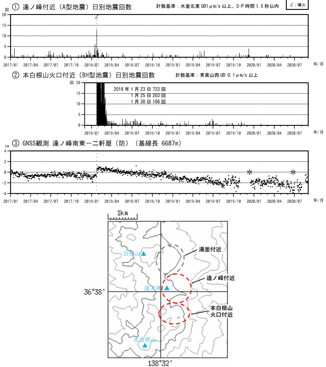
図 13 草津白根山（本白根山） 火山活動経過図（2017年1月1日～2020年8月31日）
