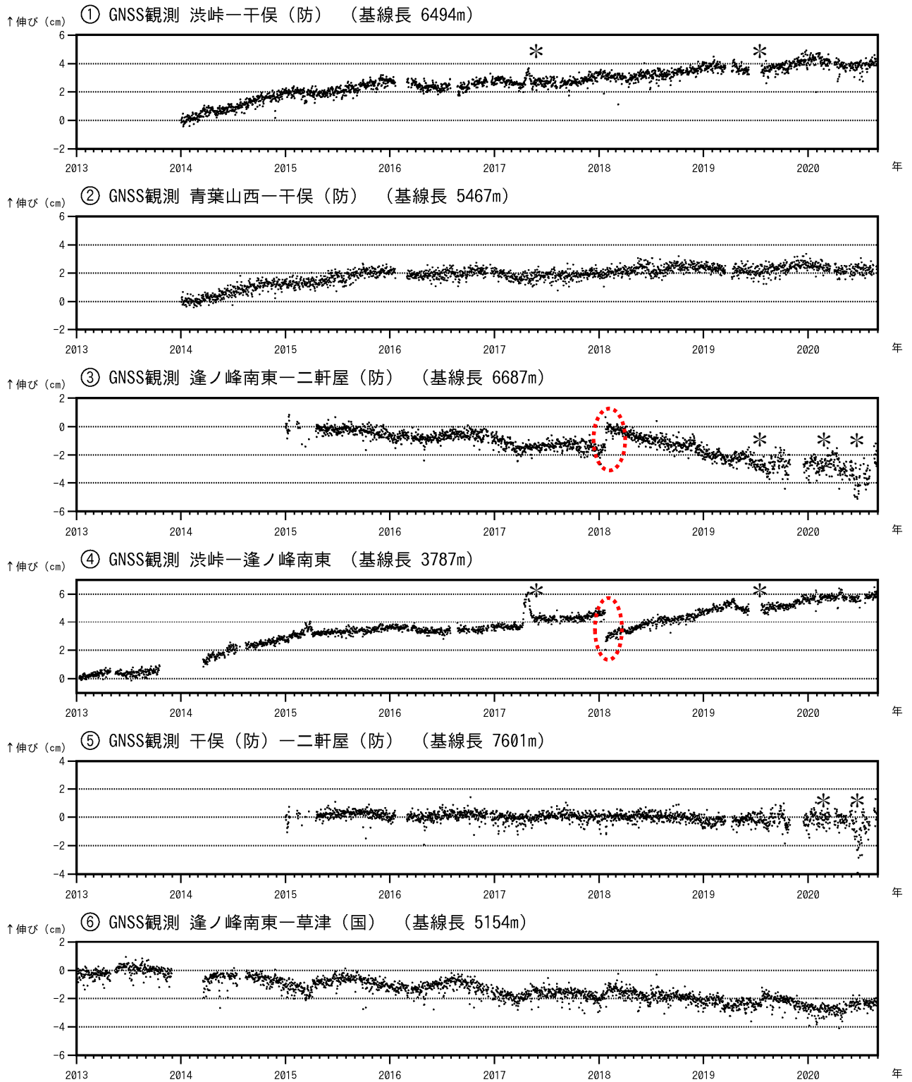
図7 草津白根山 GNSS連続観測の結果（2013年1月1日～2020年8月31日）
