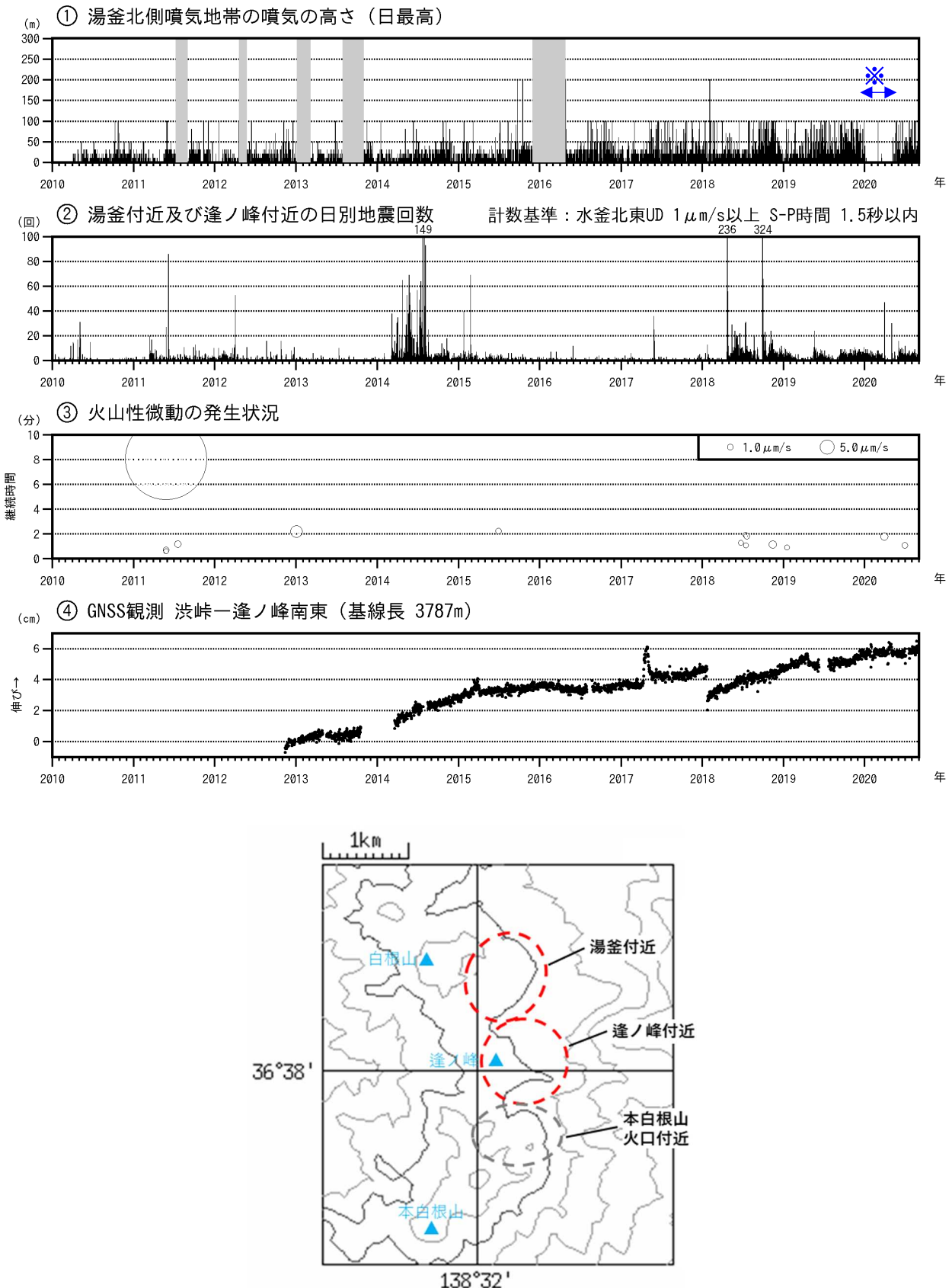
図4 草津白根山（白根山（湯釜付近））火山活動経過図（2010年1月1日～2020年8月31日） ①の灰色部分及び④の空白部分は欠測を示します。また、※の青矢印期間（2020年1月から4月にかけて）は、一部の観測機器で障害が発生しているため、100m未満の噴気については観測できていない期間があります。 ④は図8の④の基線に対応しています。2013年1月に解析方法を変更しています。 最下段の図は、図2①②と図4②の地震の震源の概ねの位置を示しています。 ・GNSS連続観測では、火山活動によるとみられる変動は認められません。
