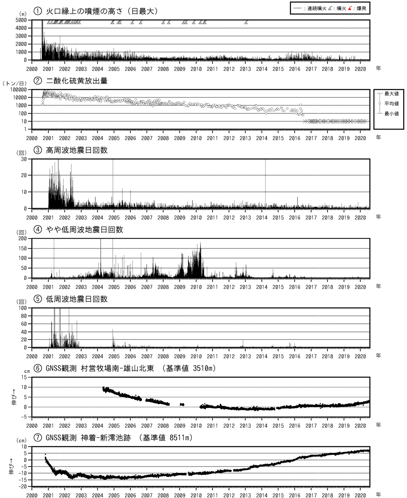
図5 三宅島 火山活動長期経過図（2000年1月1日～2020年7月31日）
