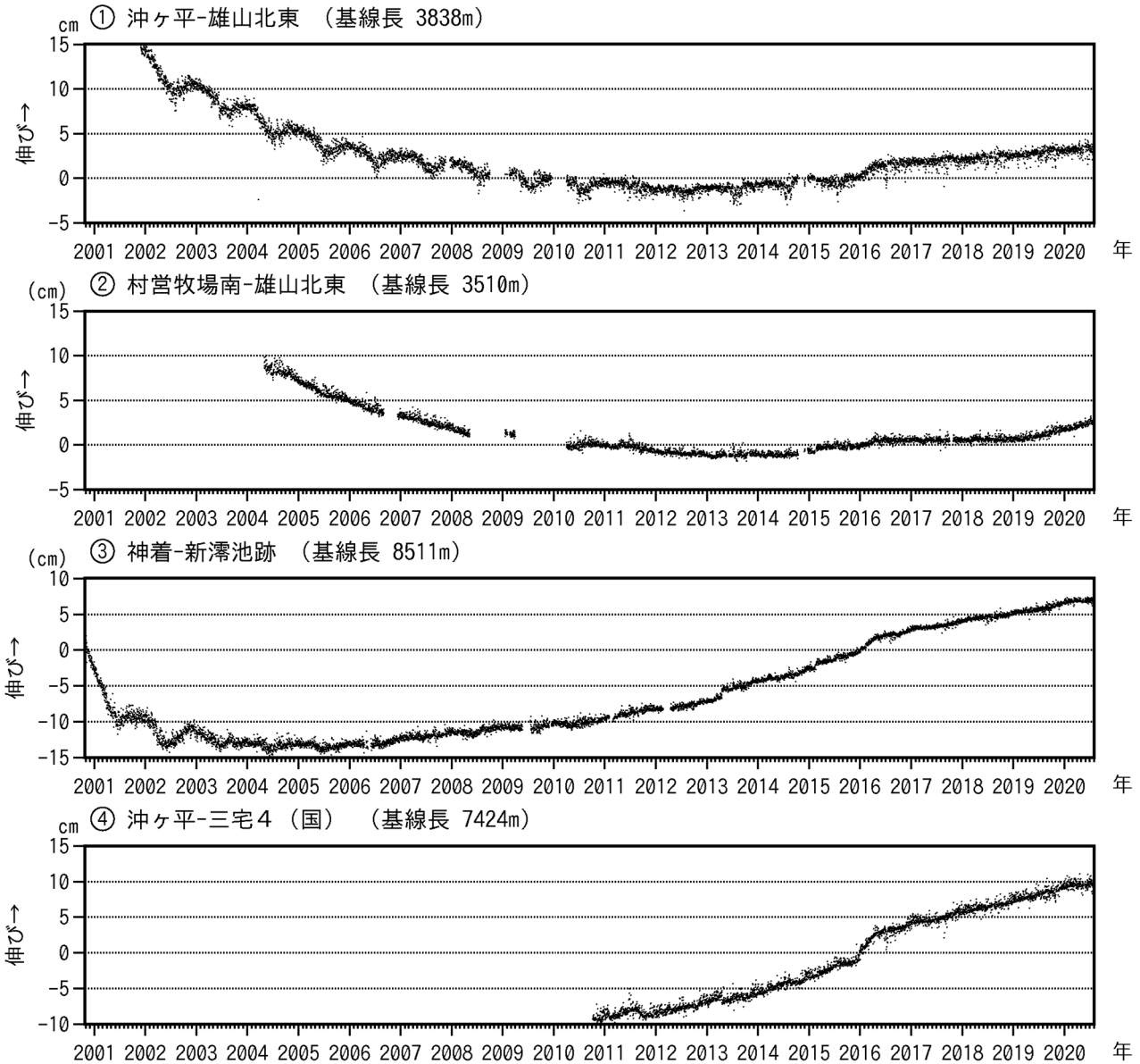
図7 三宅島 GNSS 連続観測結果（2000年10月26日～2020年7月31日）
