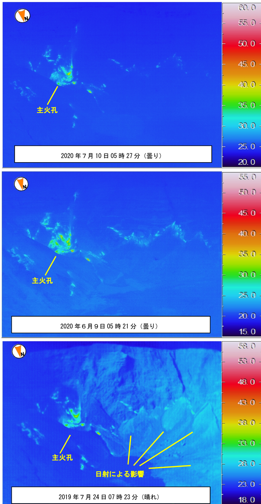
図4 三宅島 赤外熱映像装置による山頂火口内の地表面温度分布 10日に実施した機動観測では、6月や昨年と同様に主火孔内及びその周辺で引き続き高温領域が認められました。高温領域の分布に特段の変化は認められません。
