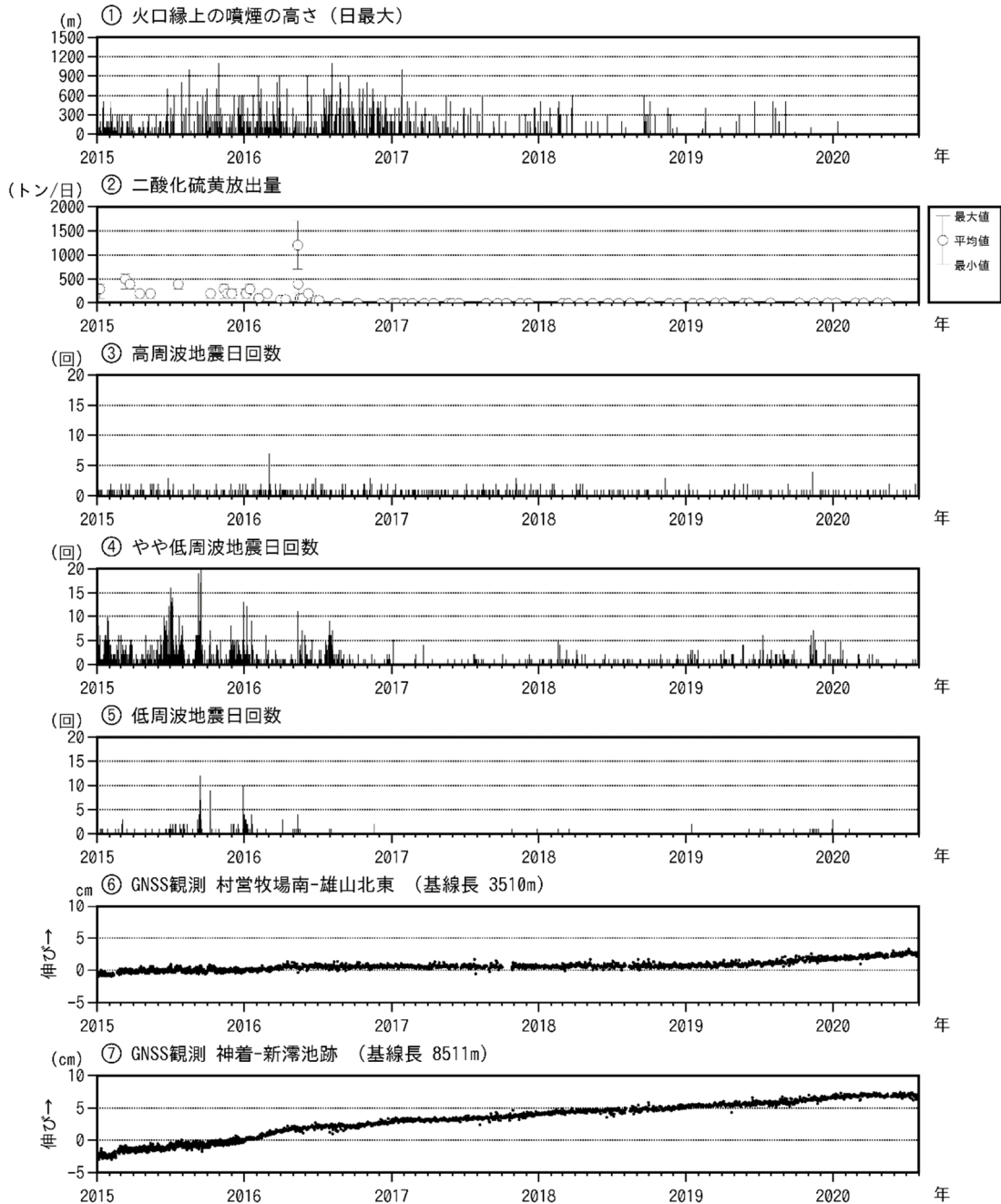
図6 三宅島 火山活動短期経過図（2015年1月1日～2020年7月31日）
