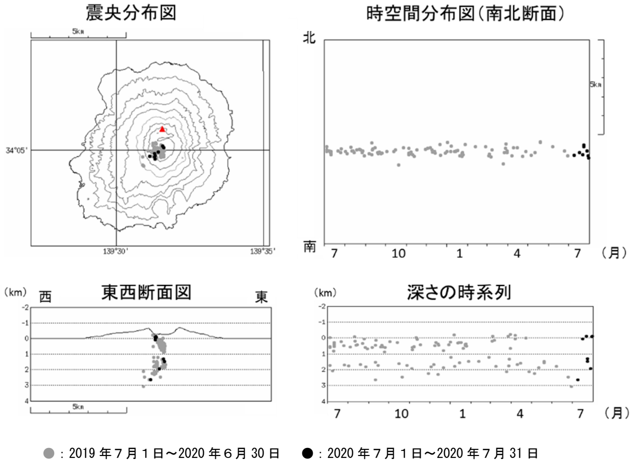
図8 三宅島 震源分布図（2019年7月1日～2020年7月31日）
