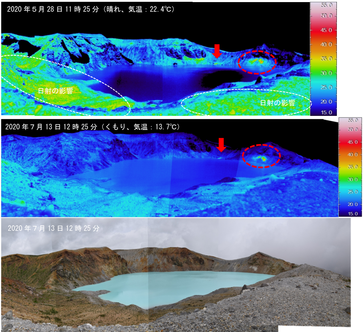
図1 - 1 草津白根山（白根山（湯釜付近）） 湯釜火口内の状況 ・13日に実施した現地調査では、前回（5月28日）の観測でも確認されていた湯釜火口内北東側火口壁の地熱域（赤破線、および赤矢印）が引き続き確認されました。
