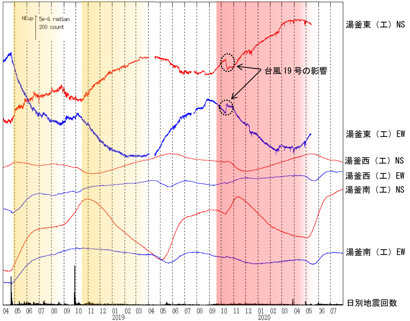
図6 草津白根山（白根山（湯釜付近）） 傾斜変動（2018年4月1日～2020年7月31日）
