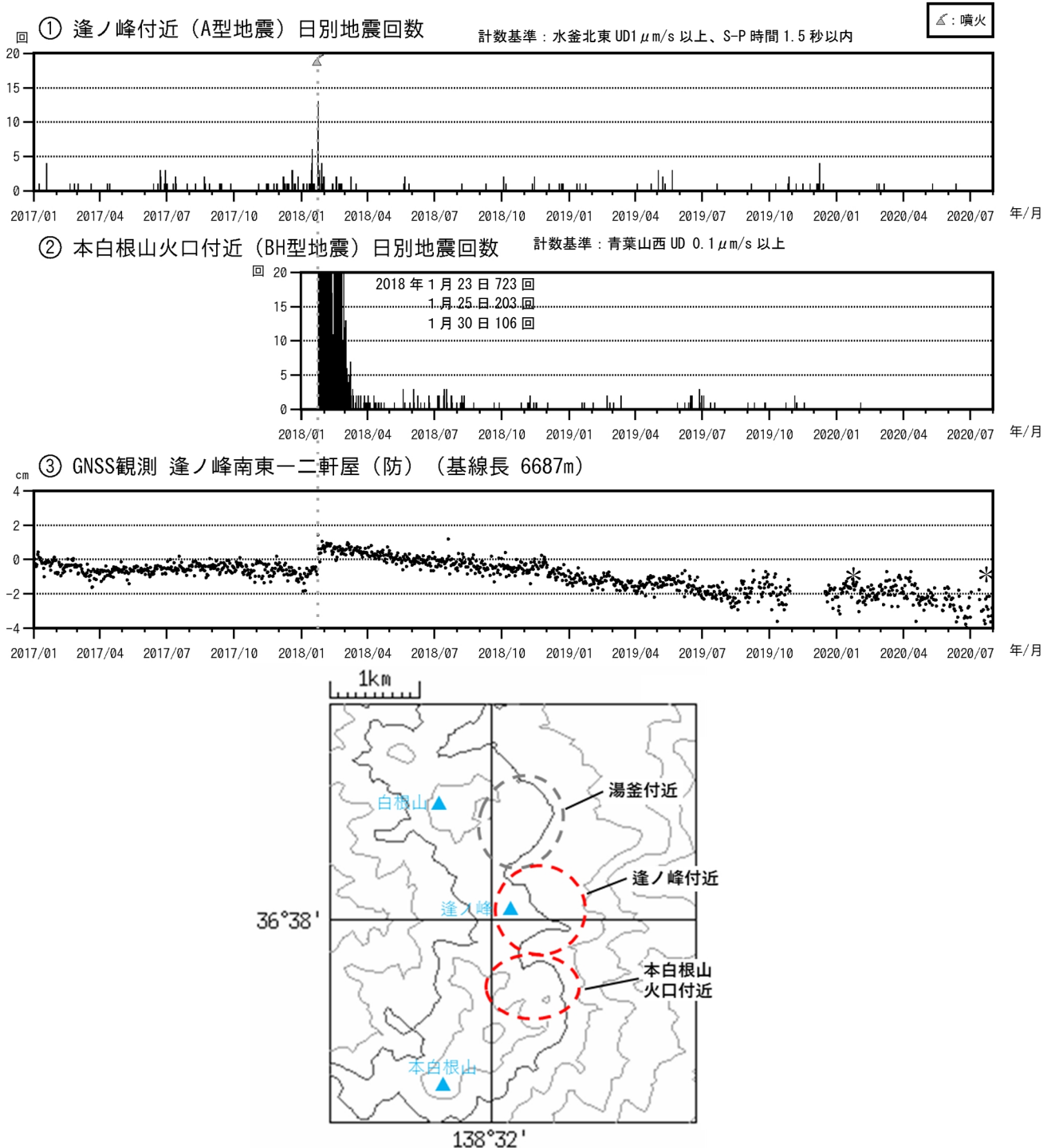
図13 草津白根山（本白根山） 火山活動経過図（2017年1月1日～2020年7月31日）
