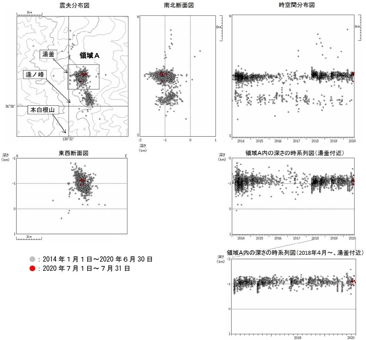
図5 草津白根山 震源分布図（2014年1月1日～2020年7月31日）
