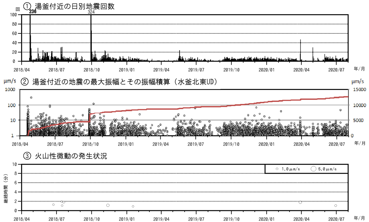
図2 草津白根山（白根山（湯釜付近）） 湯釜付近の地震活動及び火山性微動の発生状況 （2018年4月1日～2020年7月31日）（中段 ○：最大振幅（左軸）、赤線：最大振幅の積算（右軸）） ・湯釜付近を震源とする火山性地震は、やや多い状態で経過しました。
