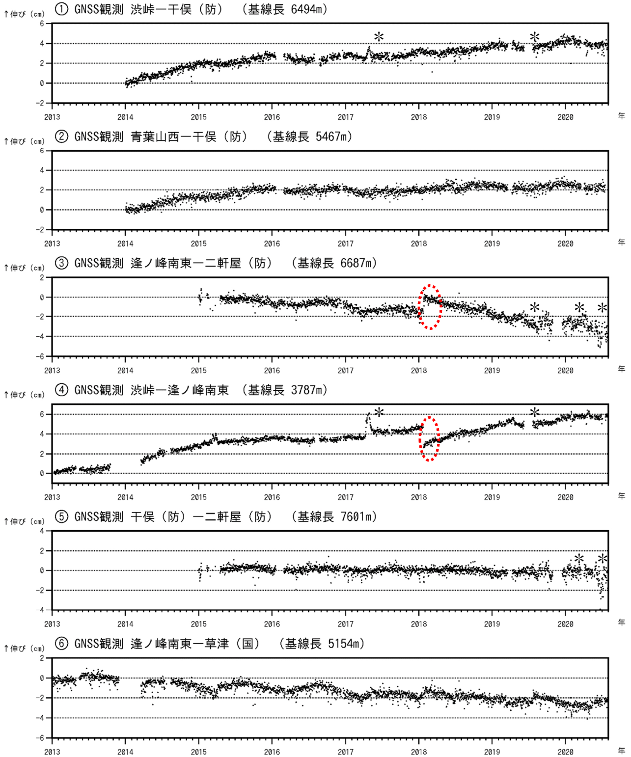
図7 草津白根山 GNSS連続観測の結果（2013年1月1日～2020年7月31日）
