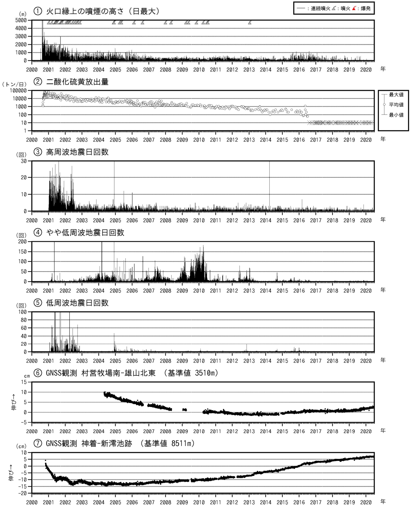
図5 三宅島 火山活動長期経過図（2000年1月1日～2020年6月30日）
