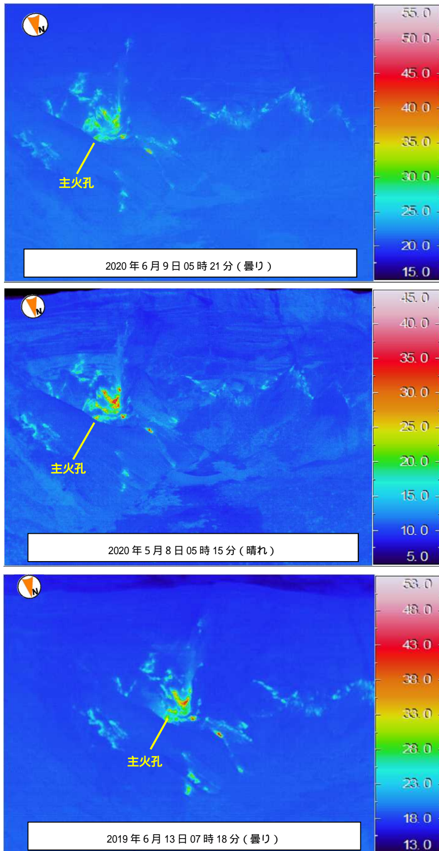
図4 三宅島 赤外熱映像装置による山頂火口内の地表面温度分布 9日に実施した機動観測では、5月や昨年と同様に主火口内及びその周辺で引き続き高温領域が認められました。高温領域の分布に特段の変化は認められません。
