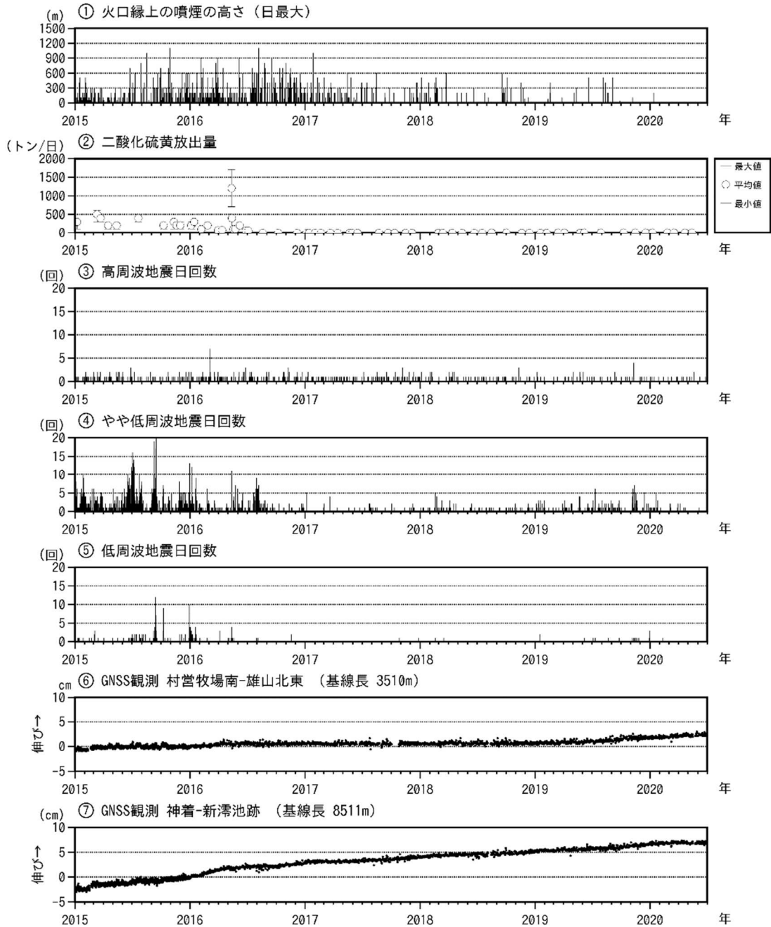
図6 三宅島 火山活動短期経過図（2015年1月1日～2020年6月30日）
