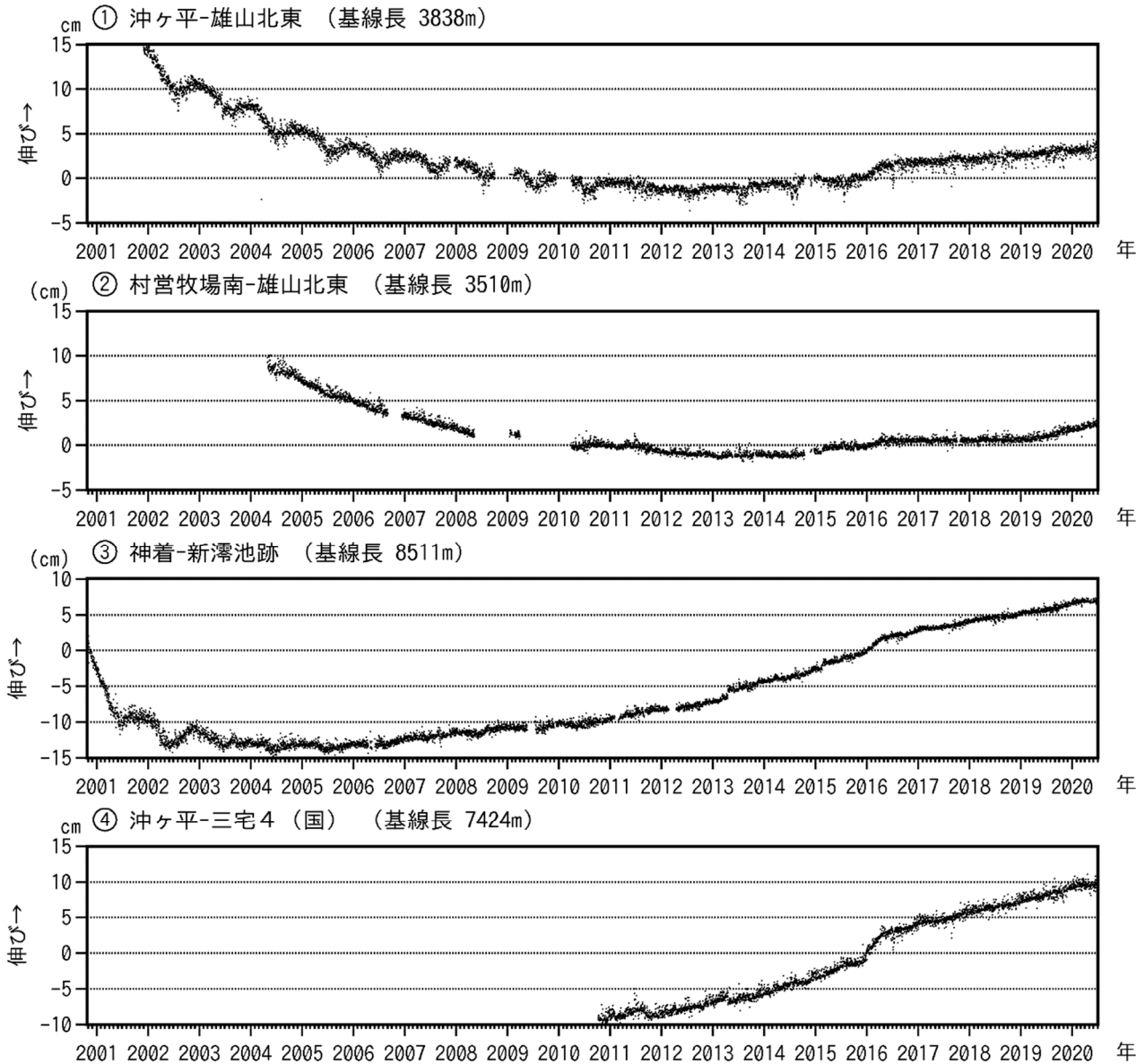
図7 三宅島 GNSS 連続観測結果 (2000年10月26日~2020年6月30日)
