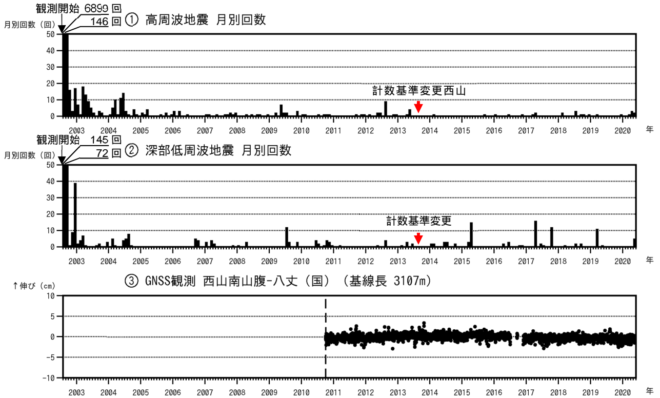
図2 八丈島 火山活動経過図（2002年8月13日～2020年5月31日）
