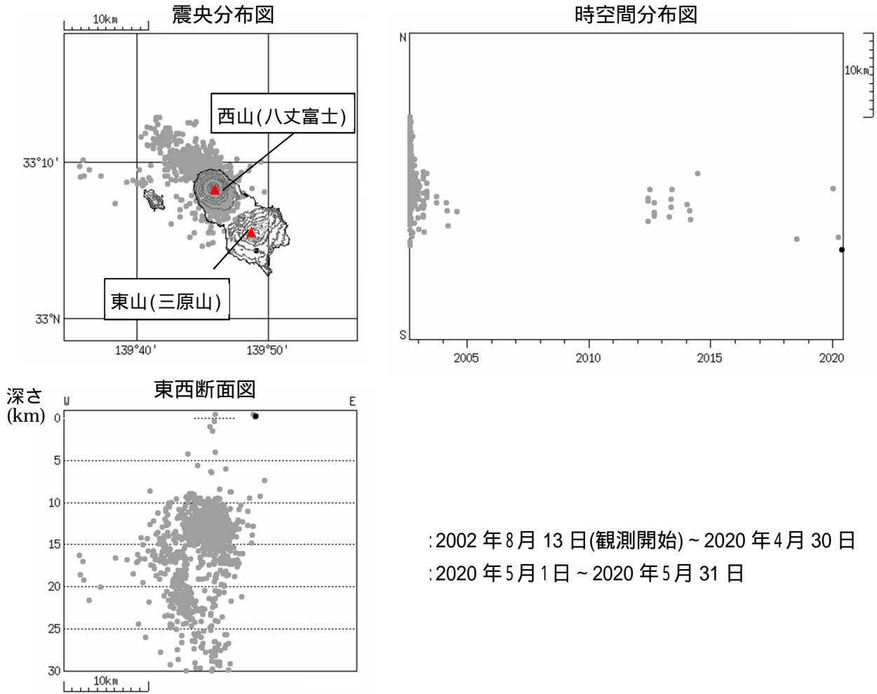
図3 八丈島 震源分布図（2002年8月13日～2020年5月31日） 今期間発生した火山性地震の震源は、東山（三原山）直下の海拔0 km 付近に求まりました。
