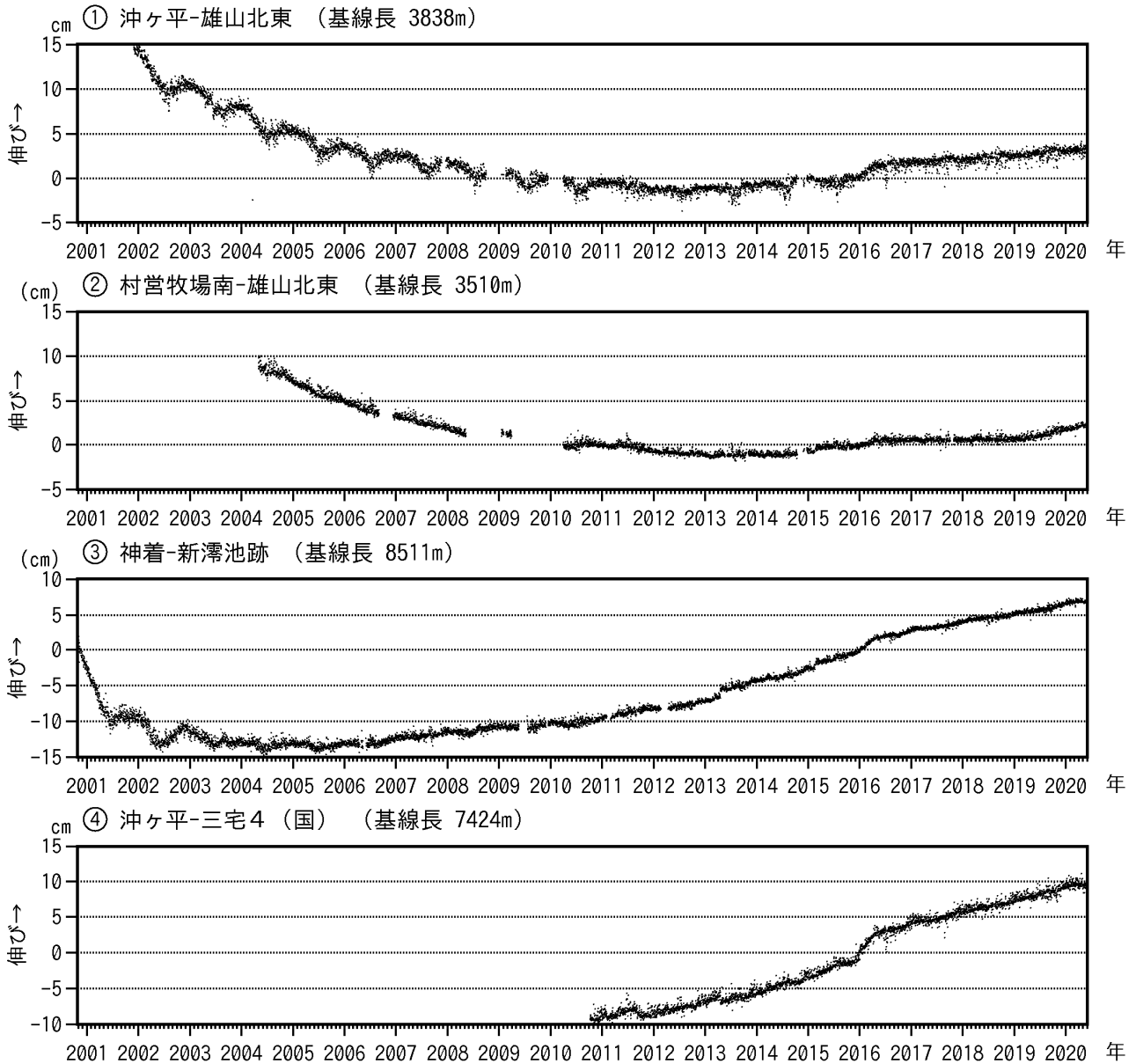
図7 三宅島 GNSS 連続観測結果（2000年10月26日～2020年5月31日）
