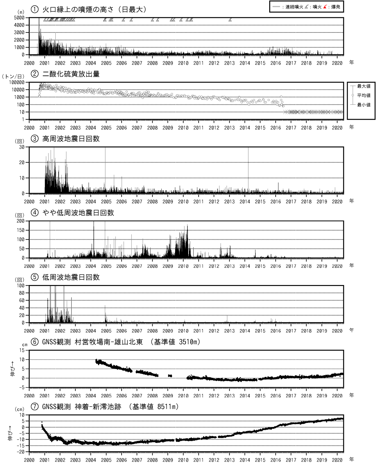
図5 三宅島 火山活動長期経過図（2000年1月1日～2020年5月31日） ※図5の説明は次ページに掲載しています。
