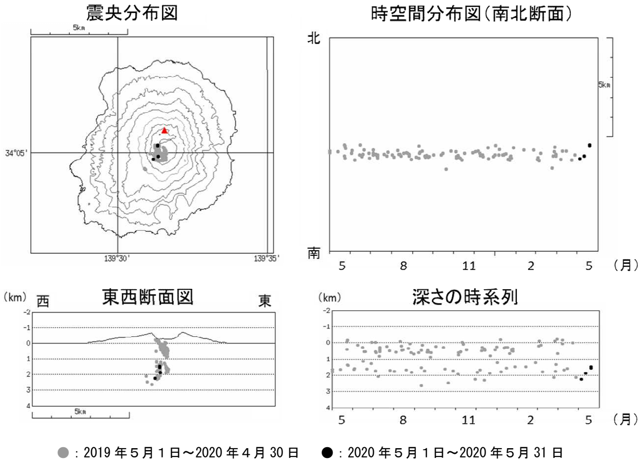
図8 三宅島 震源分布図（2019年5月1日～2020年5月31日）
