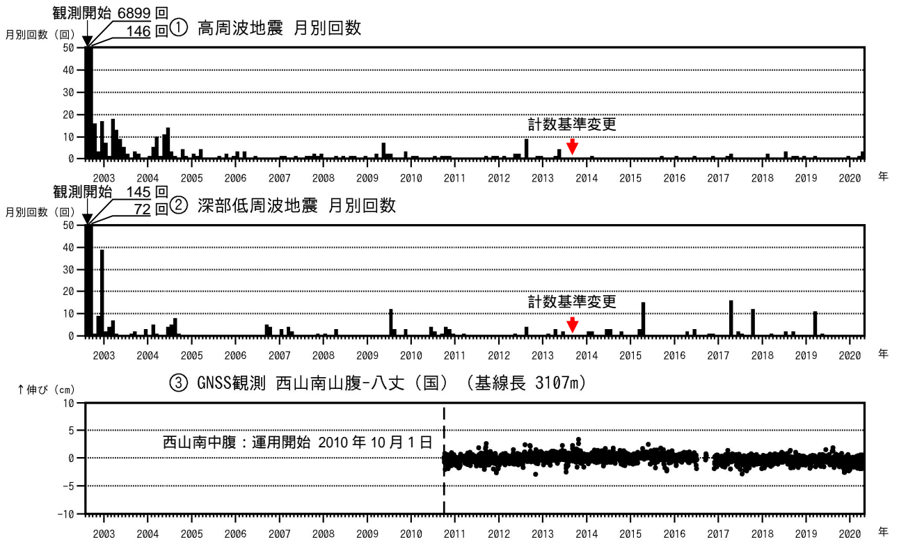
図2 八丈島 火山活動経過図（2002年8月13日～2020年4月30日）
