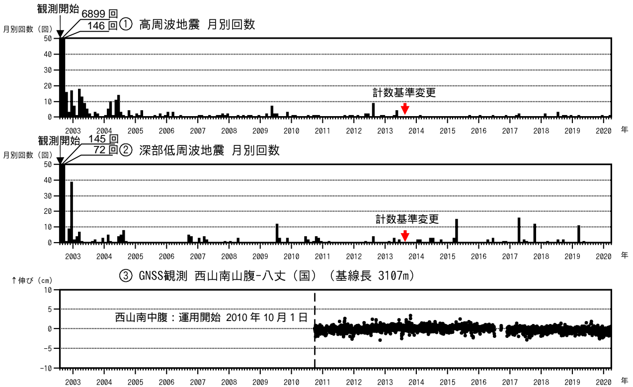
図2 八丈島 火山活動経過図(2002年8月13日~2020年3月31日)
