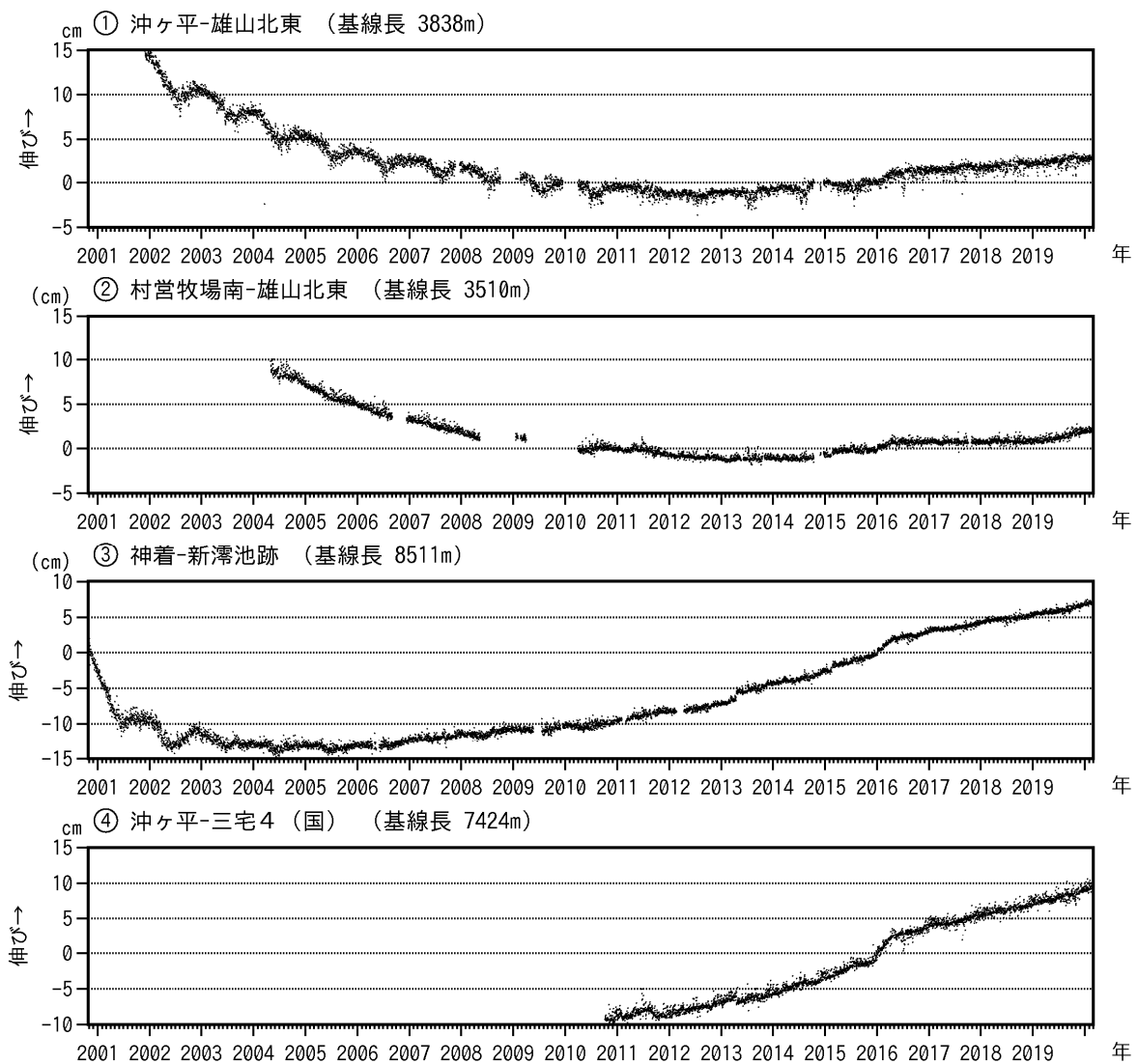
図7 三宅島 GNSS 連続観測結果（2000年10月26日～2020年2月29日）
