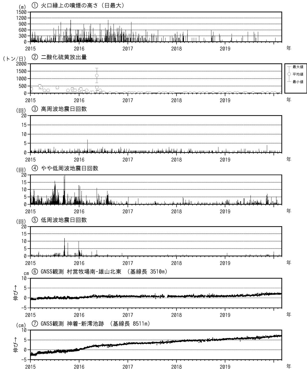
図6 三宅島 火山活動短期経過図（2015年1月1日～2020年2月29日）
