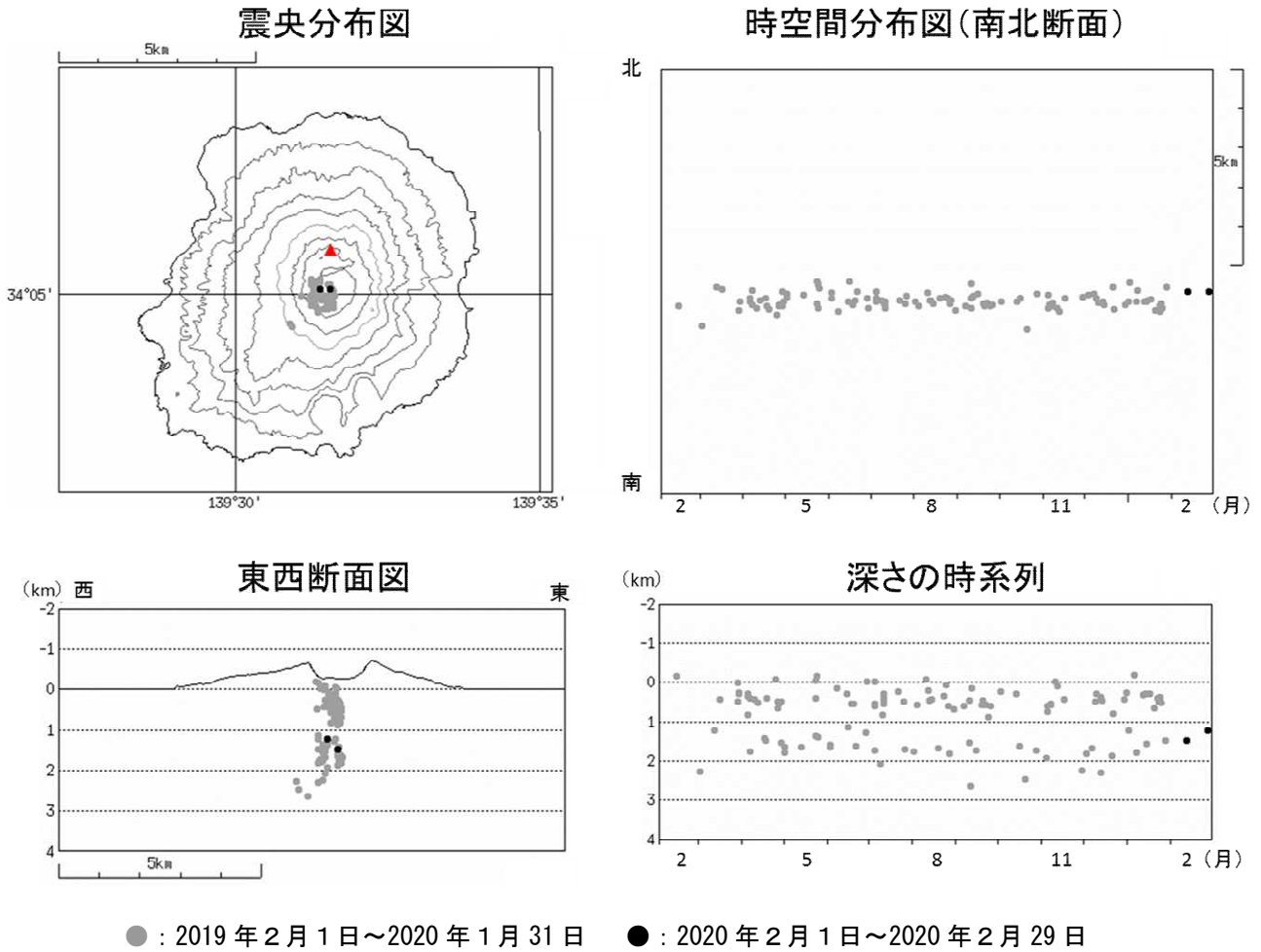
図8 三宅島 震源分布図（2019年2月1日～2020年2月29日）
