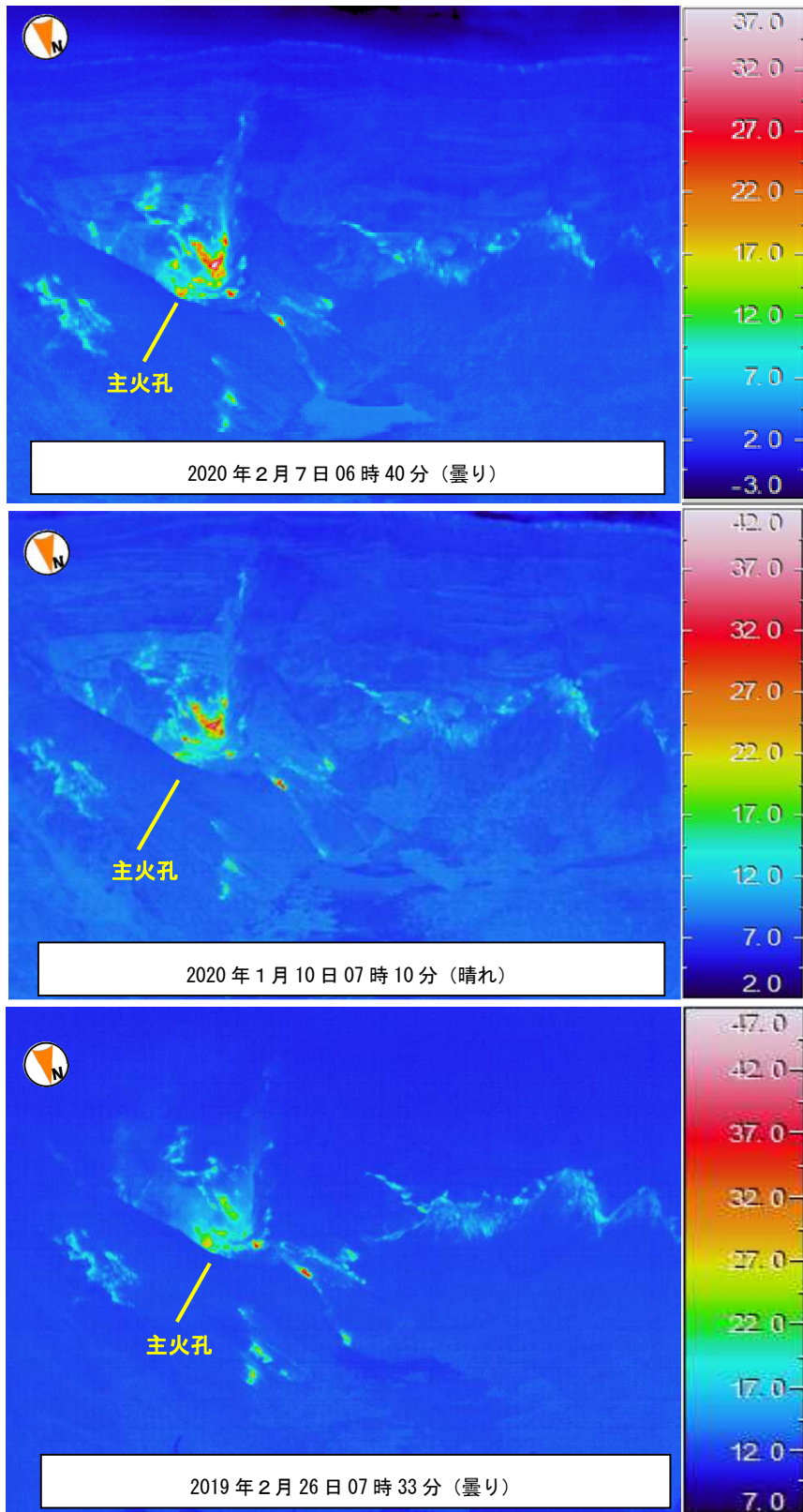
図4 三宅島 赤外熱映像装置による山頂火口内の地表面温度分布 7日に実施した機動観測では、1月や昨年と同様に主火口内及びその周辺で引き続き高温領域が認められました。高温領域の分布に特段の変化は認められません。
