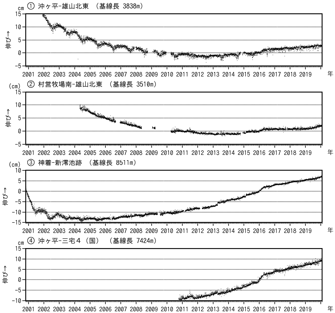
図7 三宅島 GNSS 連続観測結果（2000年10月26日～2020年1月31日）
