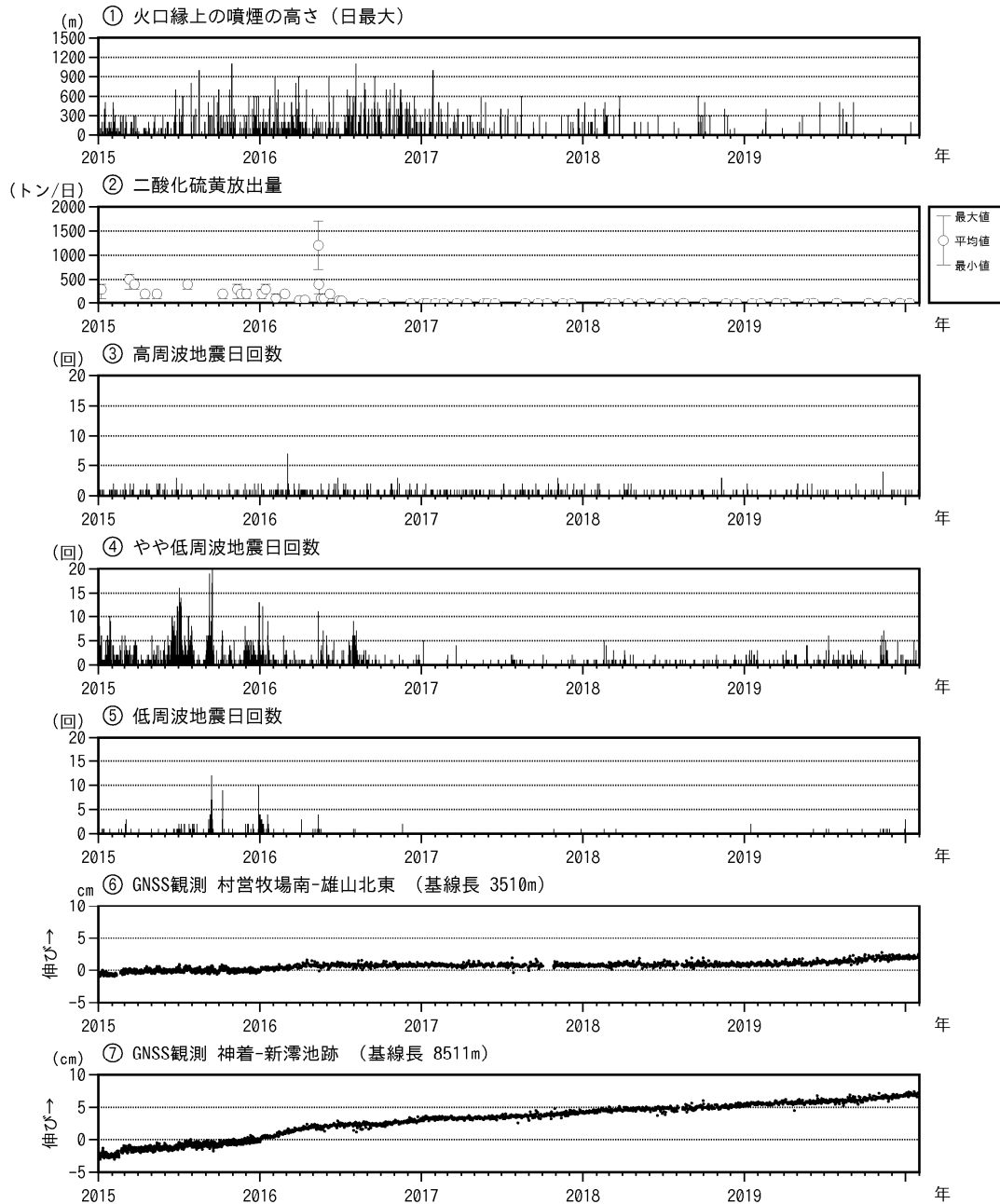
図6 三宅島 火山活動短期経過図（2015年1月1日～2020年1月31日）
