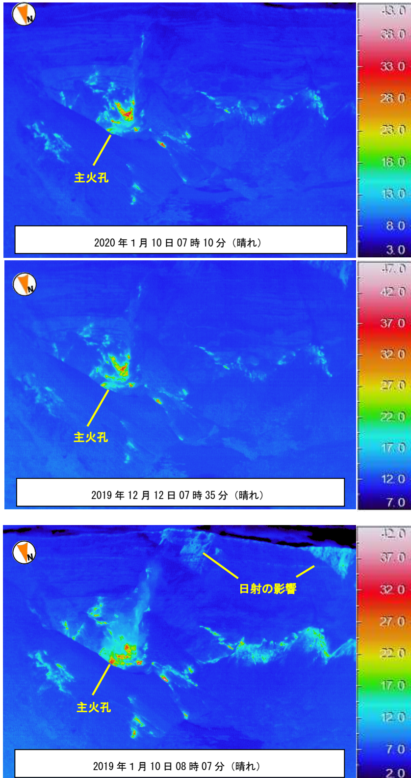
図4 三宅島 赤外熱映像装置による山頂火口内の地表面温度分布 10日に実施した機動観測では、2019年12月や昨年と同様に主火孔内及びその周辺で引き続き高温領域が認められました。高温領域の分布に特段の変化は認められません。
