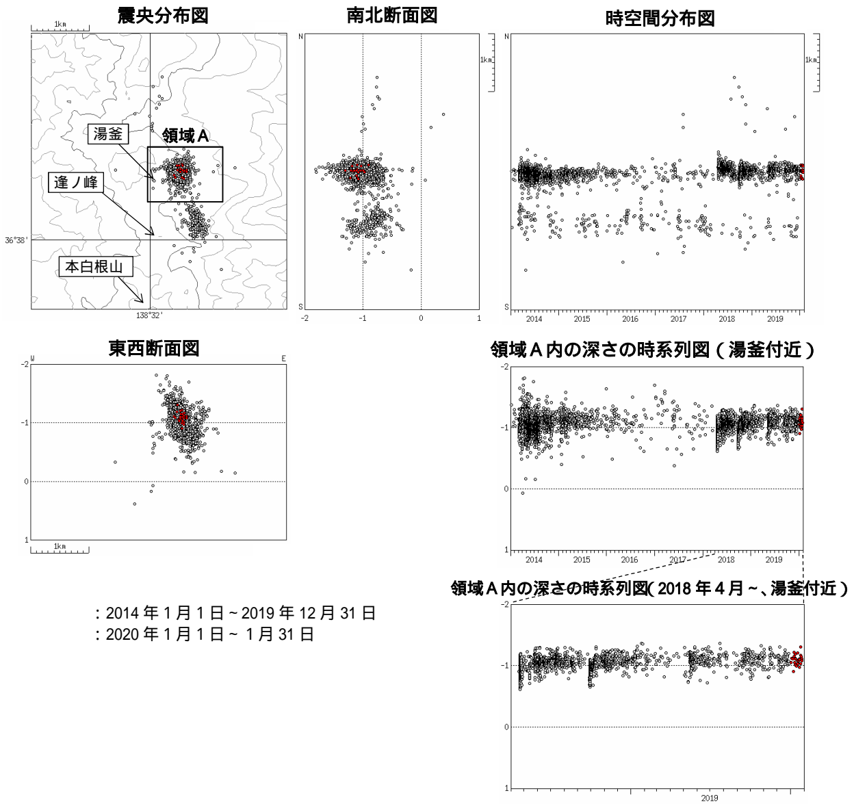
図4 草津白根山 震源分布図（2014年1月1日～2020年1月31日） 火山性地震の震源は、主に湯釜付近の海拔約1 km に分布しました。
