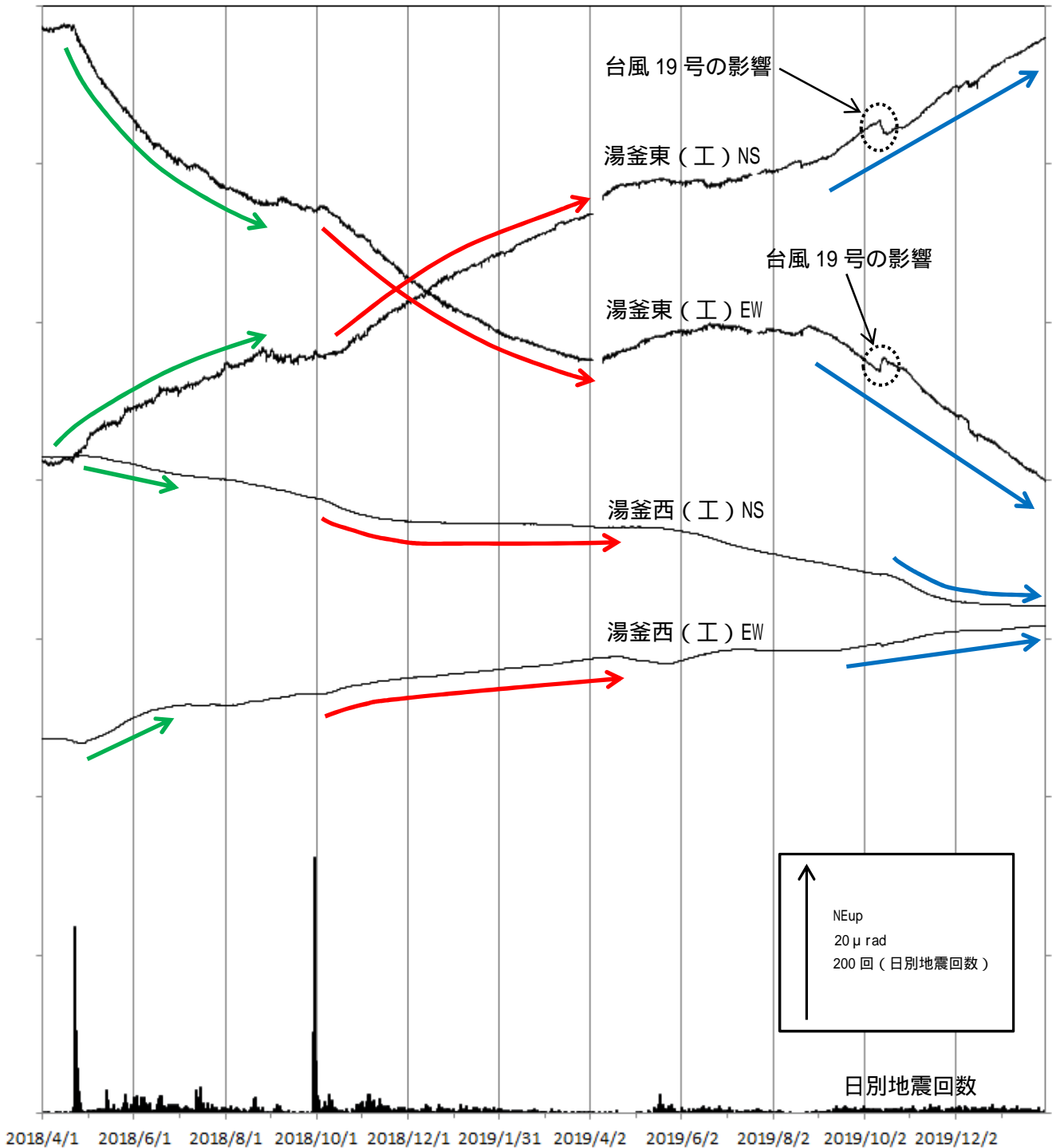
図5 草津白根山（白根山（湯釜付近）） 傾斜変動（2018年4月1日～2020年1月31日）
