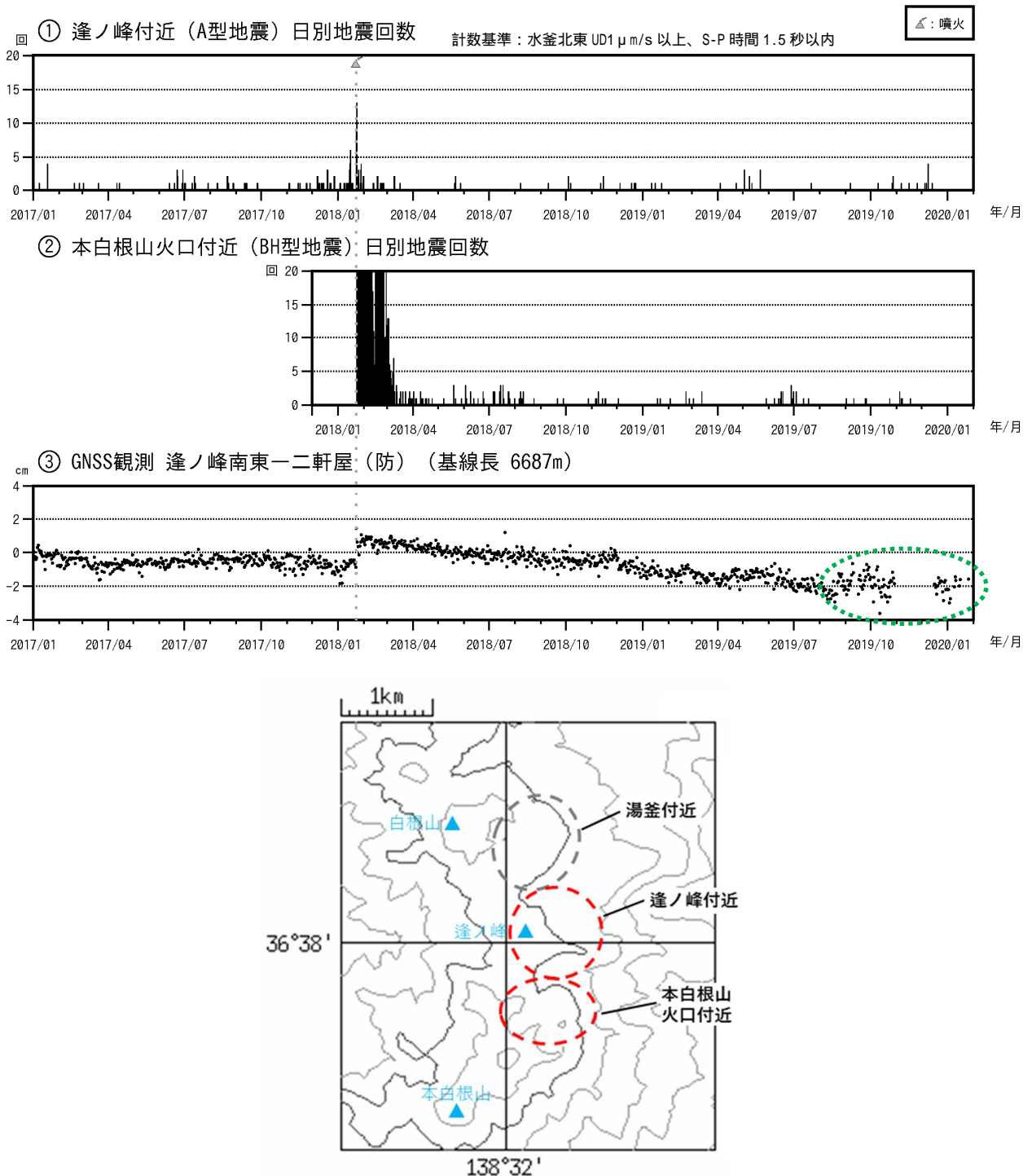
図12 草津白根山（本白根山） 火山活動経過図（2017年1月1日～2020年1月31日） 草津白根山では、火山性地震はその発生領域から、「湯釜付近」、「逢ノ峰付近」、「本白根山火口付近」に分けています。 本白根山の火山活動については、逢ノ峰付近と本白根山火口付近の地震活動に注目して監視しています。 火山性地震の種類については図13を参照してください。
