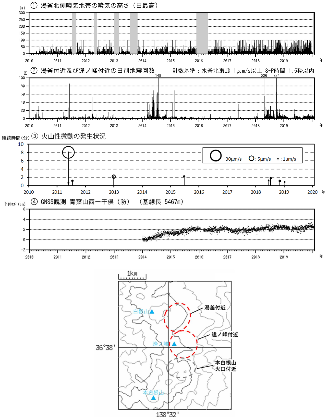
図3 草津白根山（白根山（湯釜付近））火山活動経過図（2010年1月1日～2020年1月31日） の灰色部分およびの空白部分は欠測を示します。 は図7のの基線に対応しています。 2013年1月に解析方法を変更しています。 最下段の図は、図2と図3の地震の震源の概ねの位置を示しています。 ・GNSS連続観測では、火山活動によるとみられる変動は認められません。
