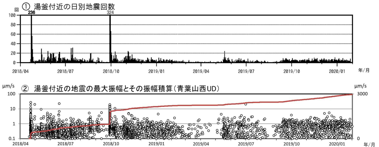
図2 草津白根山（白根山（湯釜付近）） 湯釜付近の地震活動（2018年4月1日～2020年1月31日） （○：最大振幅（左軸）、赤線：最大振幅の積算（右軸））
