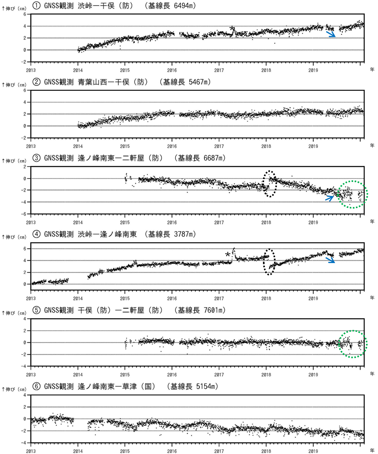
図6 草津白根山 GNSS連続観測の結果（2013年1月1日～2020年1月31日）
