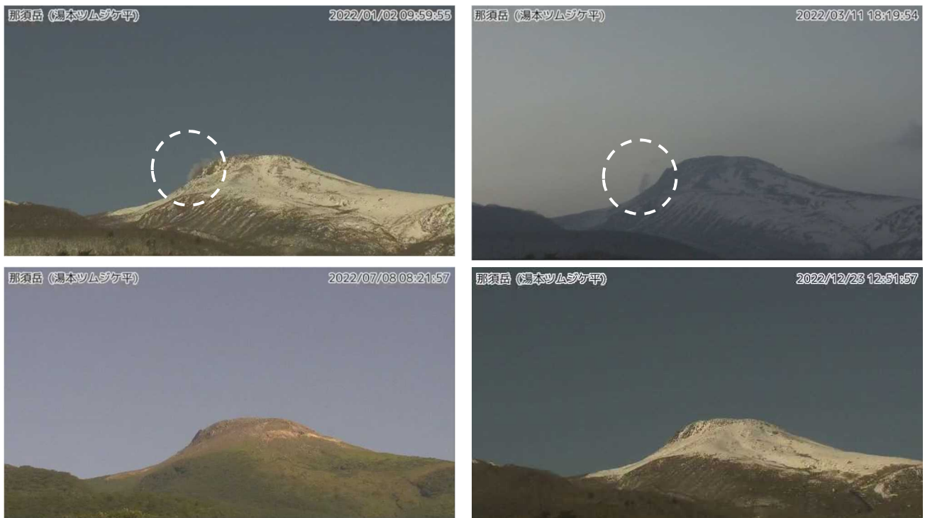
図1 那須岳 茶臼岳付近の状況（湯本ツムジケ平監視カメラによる） 左上図：2022年1月2日、右上図：2022年3月11日 左下図：2022年7月8日、右下図：2022年12月23日 白破線内は茶臼岳の西側斜面からの噴煙を示しています。
