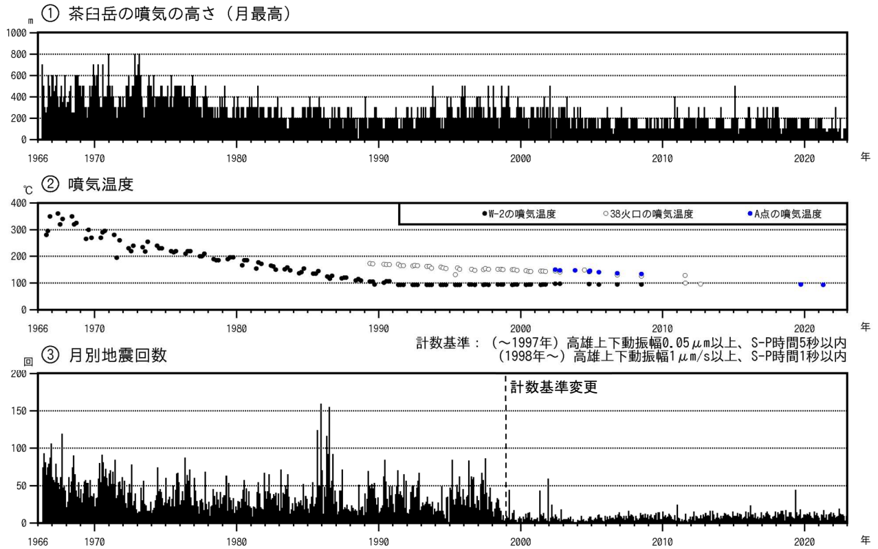
図4-1 那須岳 火山活動経過図 (1966年5月～2022年12月)
