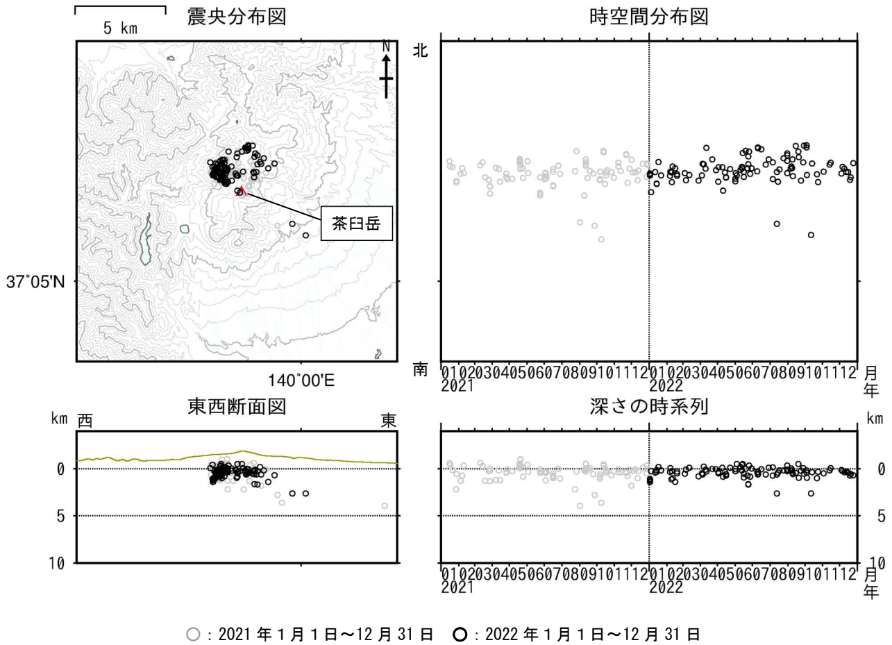
図6 那須岳 震源分布図 (2021年1月1日～2022年12月31日)
