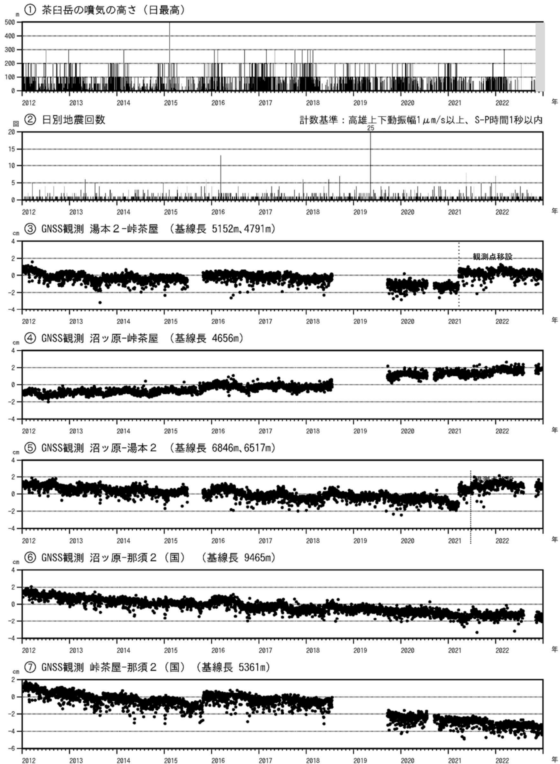
図5 那須岳 火山活動経過図 (2012年1月1日~2022年12月31日)
