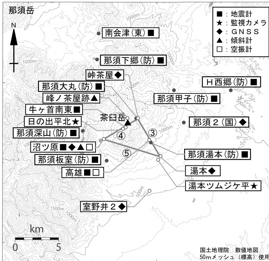
図 6 那須岳 観測点配置図
