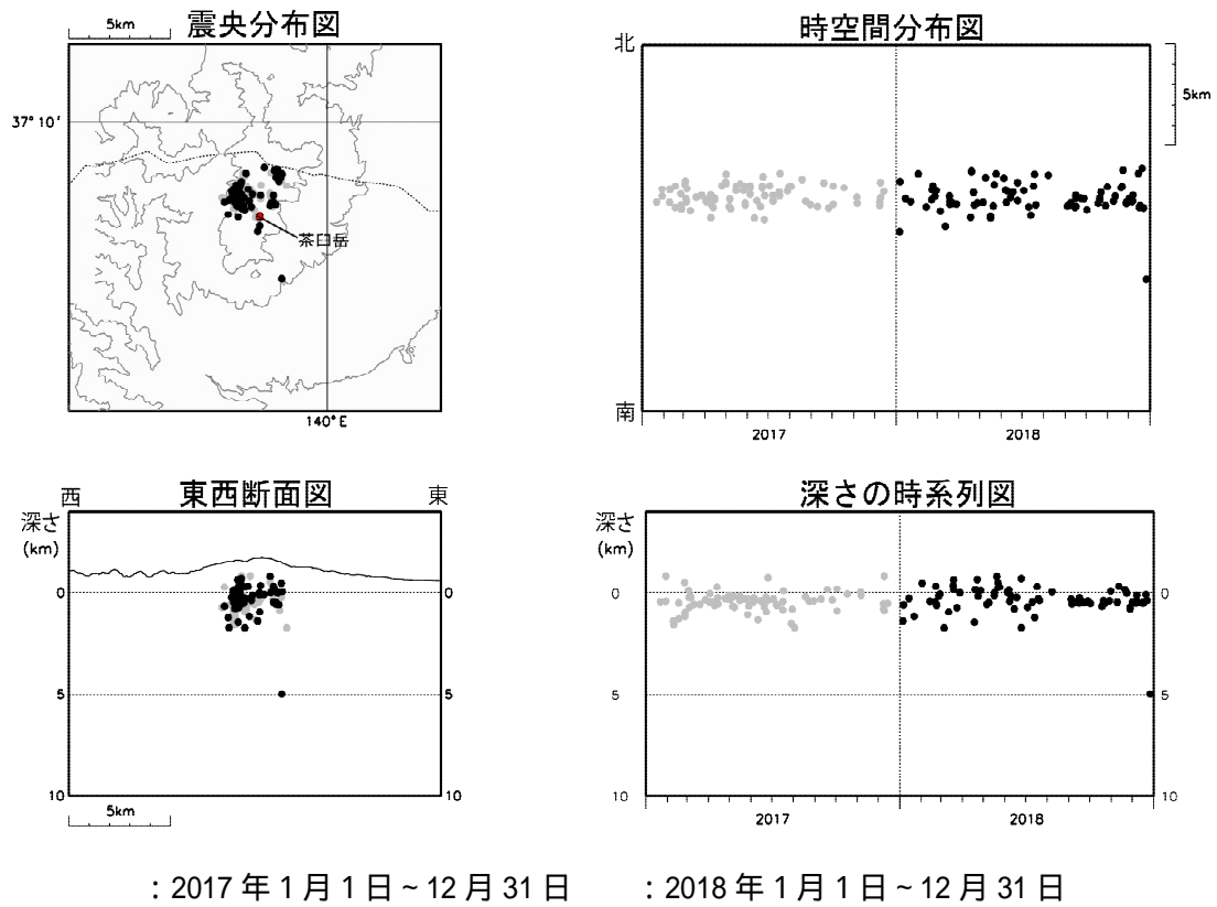
図5 那須岳 那須岳の地震観測点による震源分布図(2017年1月1日～2018年12月31日)
