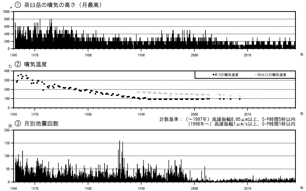
図3 那須岳 火山活動経過図 (1966年1月～2018年12月)
