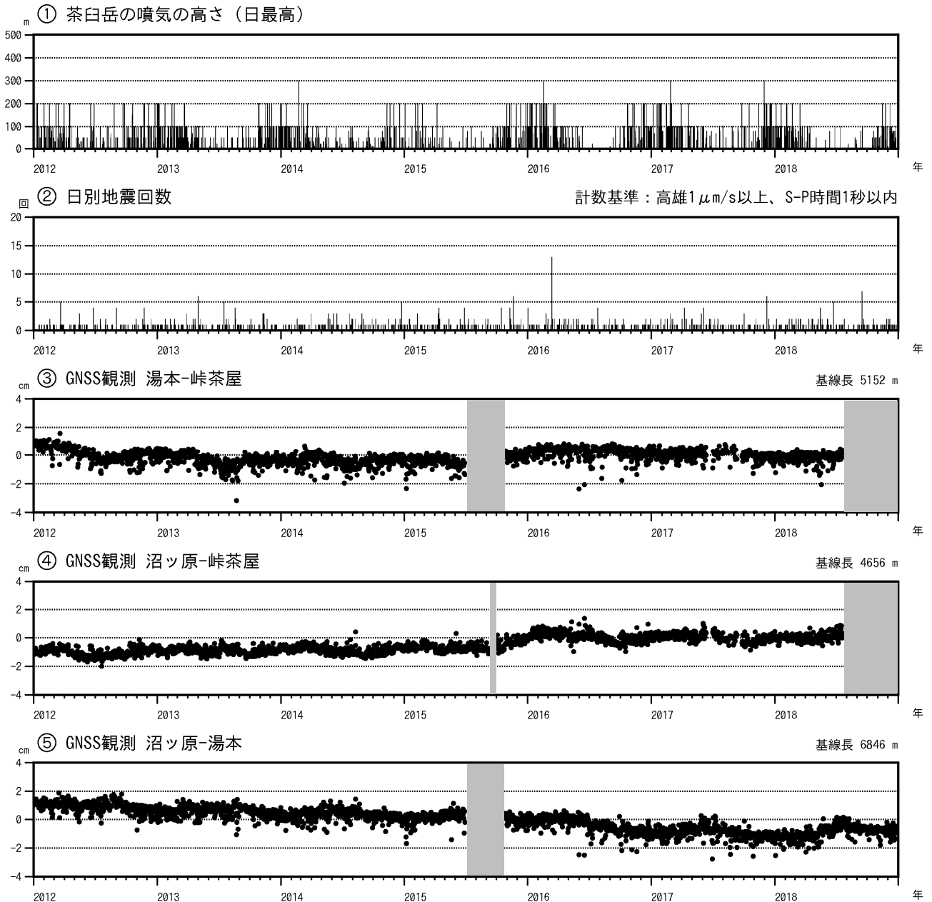
図4 那須岳 火山活動経過図 (2012年1月1日~2018年12月31日)
