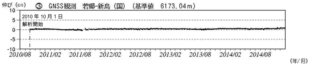
図2 新島 火山活動経過図(2010年8月2日～2014年12月31日) 新島周辺の日別地震回数 ・ 図の灰色部分は機器障害のため欠測。 GNSS連続観測による基線長変化 (国): 国土地理院 ・ は図4のGNSS基線に対応しています。
