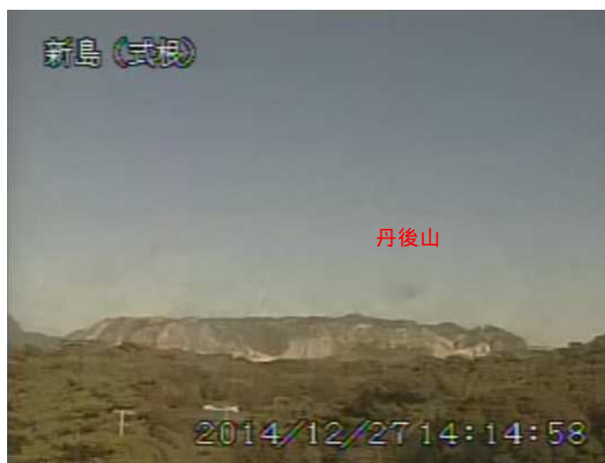
図 1 新島 丹後山山頂部の状況（12 月 27 日、式根遠望カメラによる）
