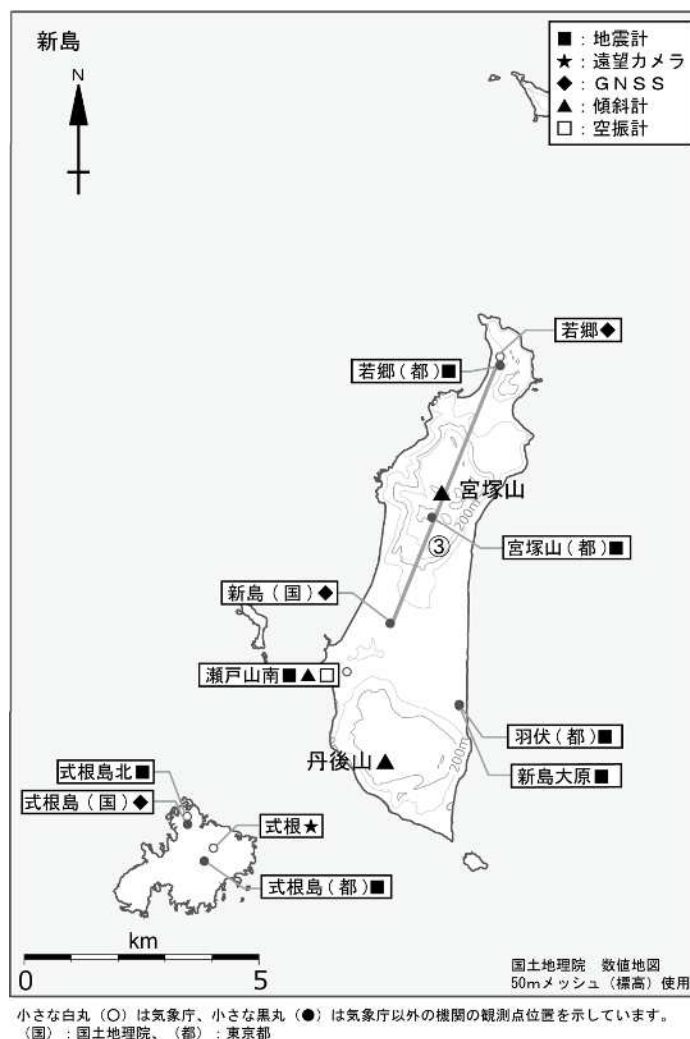
図 4 新島 観測点配置図 (GNSS 基線は図 2 の に対応しています。)
