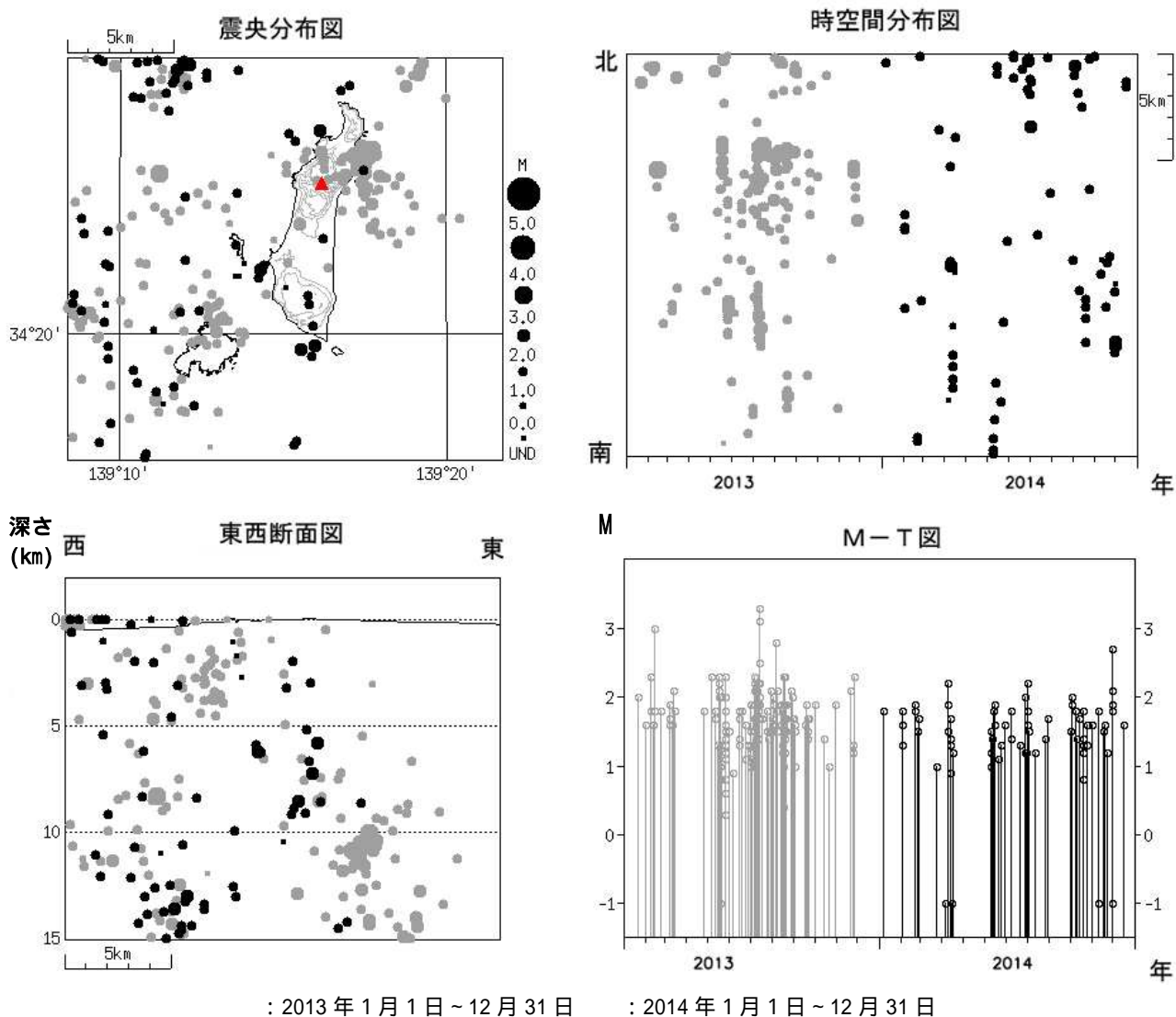
図 3 新島 広域地震観測網による山体・周辺の地震活動（2013 年 1 月 1 日～2014 年 12 月 31 日）
