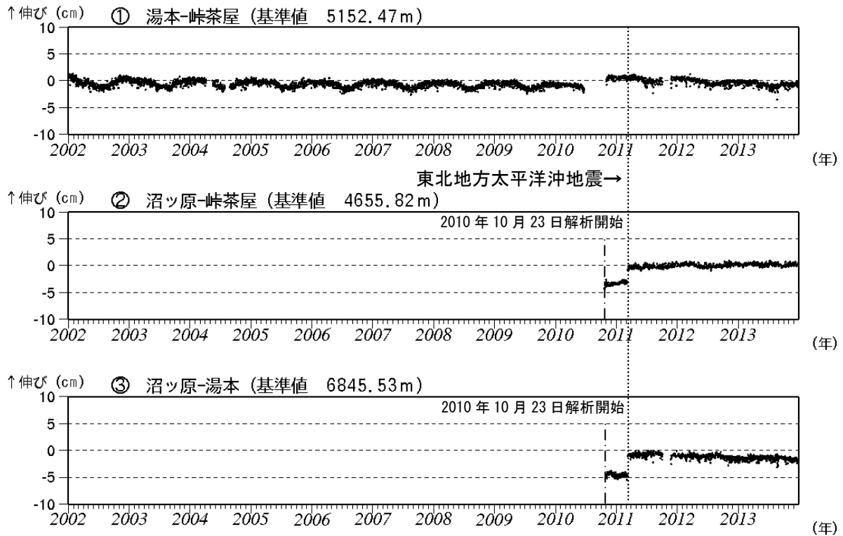
図4 那須岳 GPS連続観測による基線長変化(2002年1月～2013年12月)
