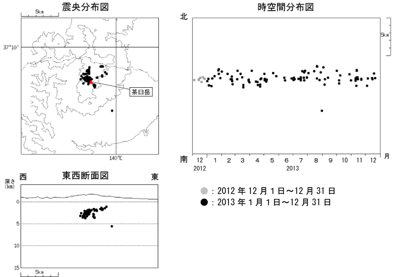
図3 那須岳 那須岳の地震観測点による震源分布図（2012年12月1日～2013年12月31日） 震源は山頂直下のごく浅い所に分布しました。
