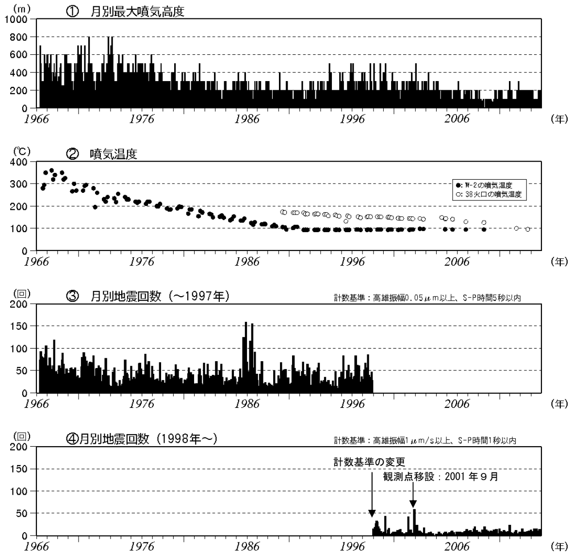
図2 那須岳 最近の火山活動の推移 (1966年1月~2013年12月)
