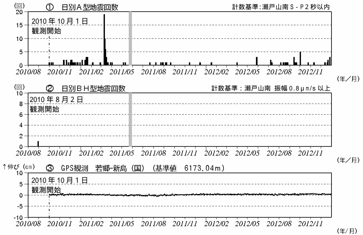
図 3 新島 火山活動経過図(2010年8月～2012年12月) : 新島周辺の日別地震回数 図の灰色部分は機器障害のため欠測。 : GPS 連続観測による基線長変化 図 5 の GPS 基線に対応しています。 (国): 国土地理院
