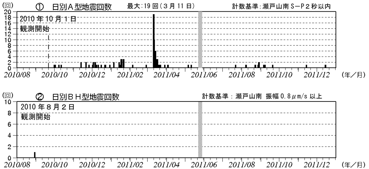
図3 新島 日別地震回数(2010年8月~2011年12月) 2011年3月~5月分は一部未処理の期間があります。 図の灰色部分は機器障害のため欠測。
