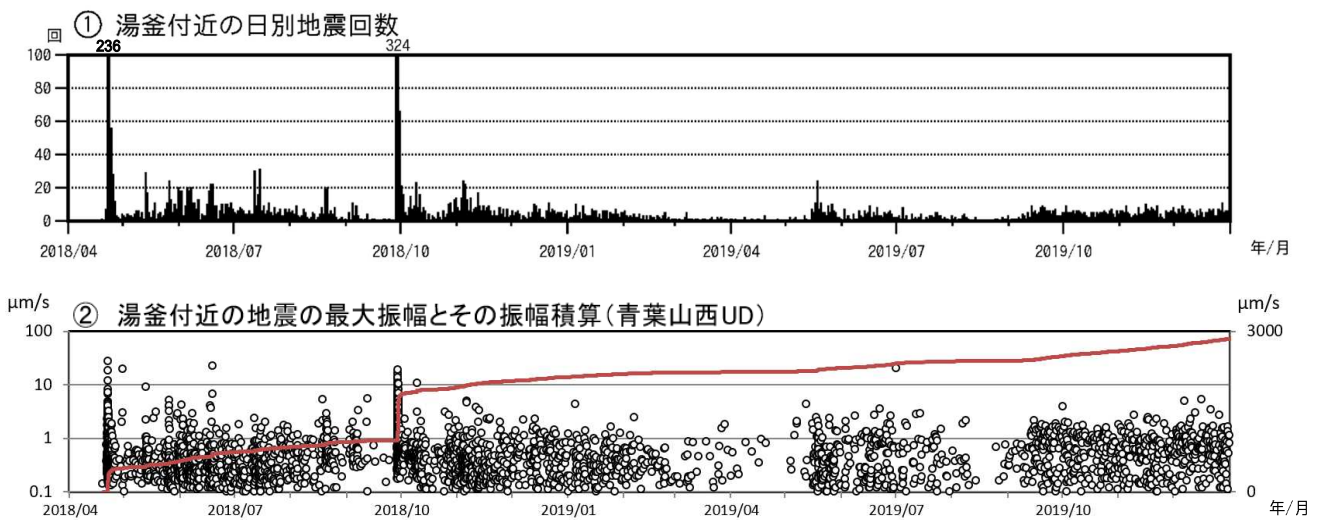
図5 草津白根山（白根山（湯釜付近）） 湯釜付近の地震活動（2018年4月1日～2019年12月31日） （○：最大振幅（左軸） 赤線：最大振幅の積算（右軸）） ・湯釜付近を震源とする火山性地震は、2019年9月上旬頃から概ねやや多い状態で経過しています。振幅の大きな火山性地震は発生していません。
