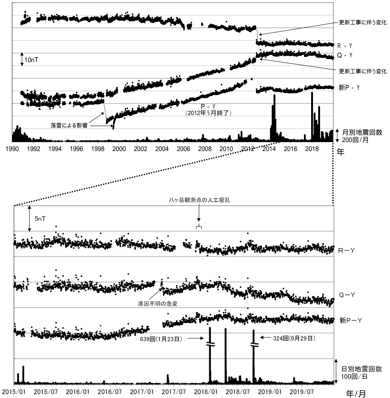
図 11 草津白根山（白根山（湯釜付近））全磁力連続観測による全磁力値の変化及び地震回数
