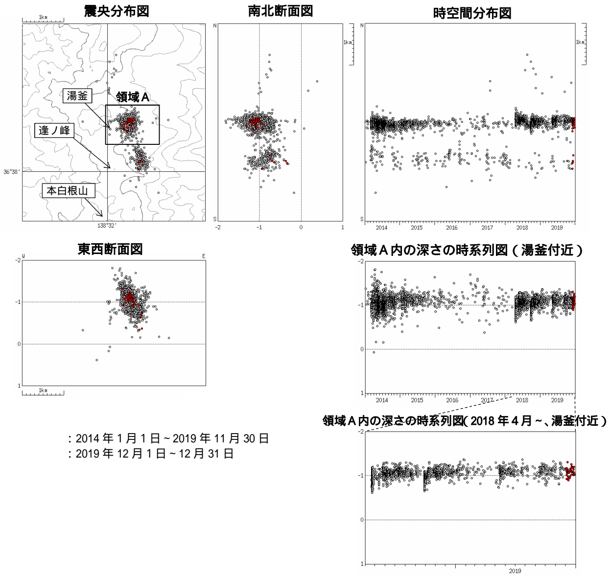
図7 草津白根山 震源分布図（2014年1月1日～2019年12月31日） 火山性地震の震源は、主に湯釜付近の海拔約1 km に分布しました。
