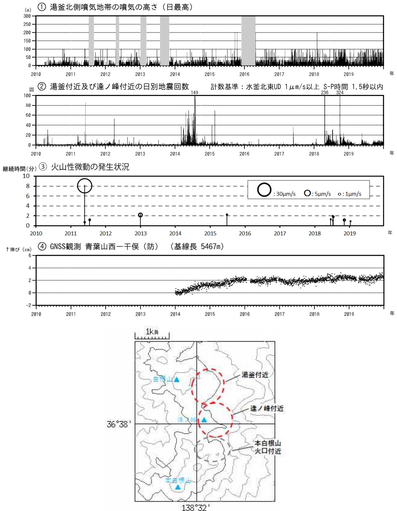
図6 草津白根山（白根山（湯釜付近））火山活動経過図（2010年1月1日～2019年12月31日） の灰色部分およびの空白部分は欠測を示します。 は図10のの基線に対応しています。 2013年1月に解析方法を変更しています。 最下段の図は、の地震の震源の概ねの位置を示しています。 ・GNSS連続観測では、火山活動によるとみられる変動は認められません。
