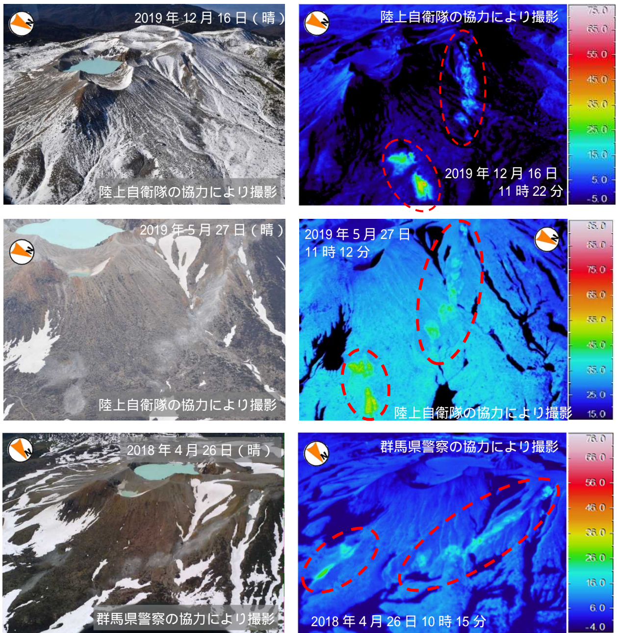
図3 草津白根山（白根山（湯釜付近）） 水釜火口北側及び北東側斜面の状況及び地表面温度分布 ・16日に陸上自衛隊の協力により実施した上空からの観測では、前回の観測（2019年5月27日）と比較して、水釜火口北側及び北東側斜面の地熱域の分布（赤破線）に特段の変化はみられませんでした。
