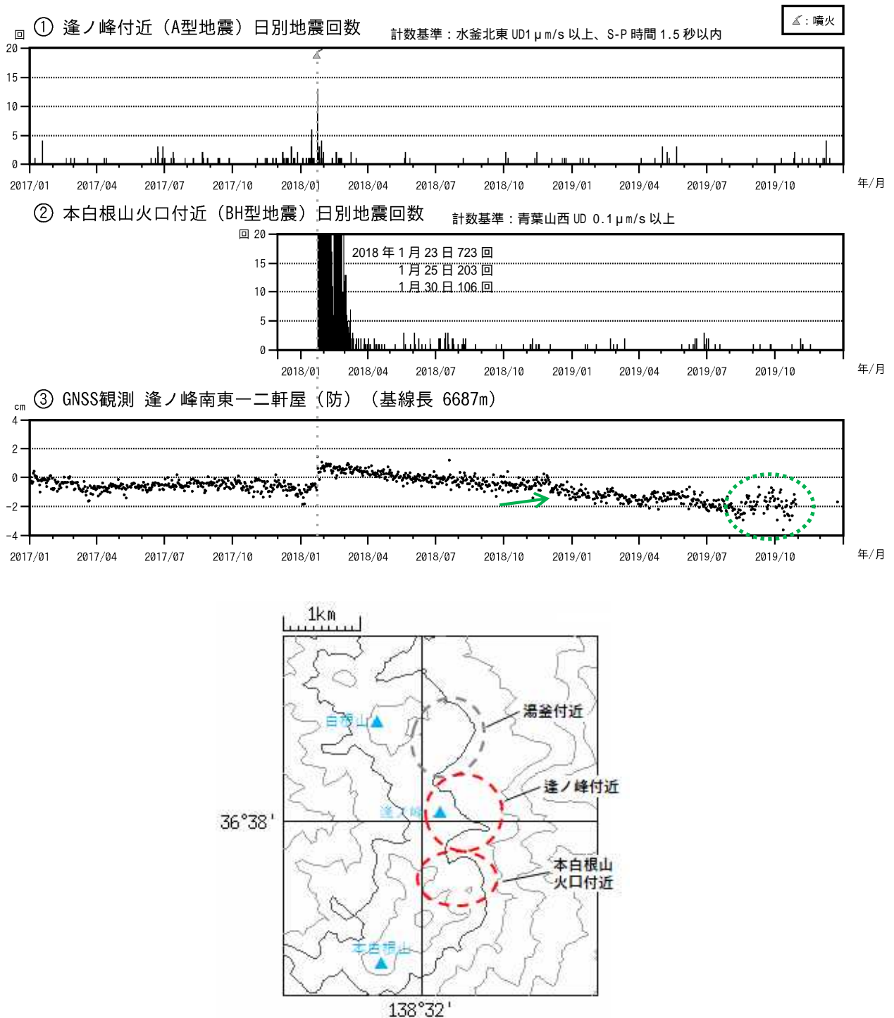
図 17 草津白根山（本白根山） 火山活動経過図（2017 年 1 月 1 日～2019 年 12 月 31 日） 草津白根山では、火山性地震はその発生領域から、「湯釜付近」、「逢ノ峰付近」、「本白根山火口付近」に分けています。本白根山の火山活動については、逢ノ峰付近と本白根山火口付近の地震活動に注目して監視しています。火山性地震の種類については図 18 を参照してください。 は図 10 の の基線に対応しています。 最下段の図は、 の地震の震源の概ねの位置を示しています。 ・ 逢ノ峰付近の火山性地震は、少ない状態で経過しています。 ・ 噴火発生後、本白根山火口付近で BH 型の火山性地震が多発しましたが、12 月以降、少ない状態で経過しています。なお、BH 型地震は、初動が不明瞭なため、震源は求まっていません。 ・ の基線で 2018 年 1 月以降にみられている変化は、本白根山の収縮によるものと考えられます。2018 年に、草津白根山の北西もしくは西側深部の膨張を示唆する変化がみられていました（緑矢印）。 ・ の基線で 2019 年 8 月頃からみられている変化（緑破線）は、火山活動によるものではないと考えられます。
