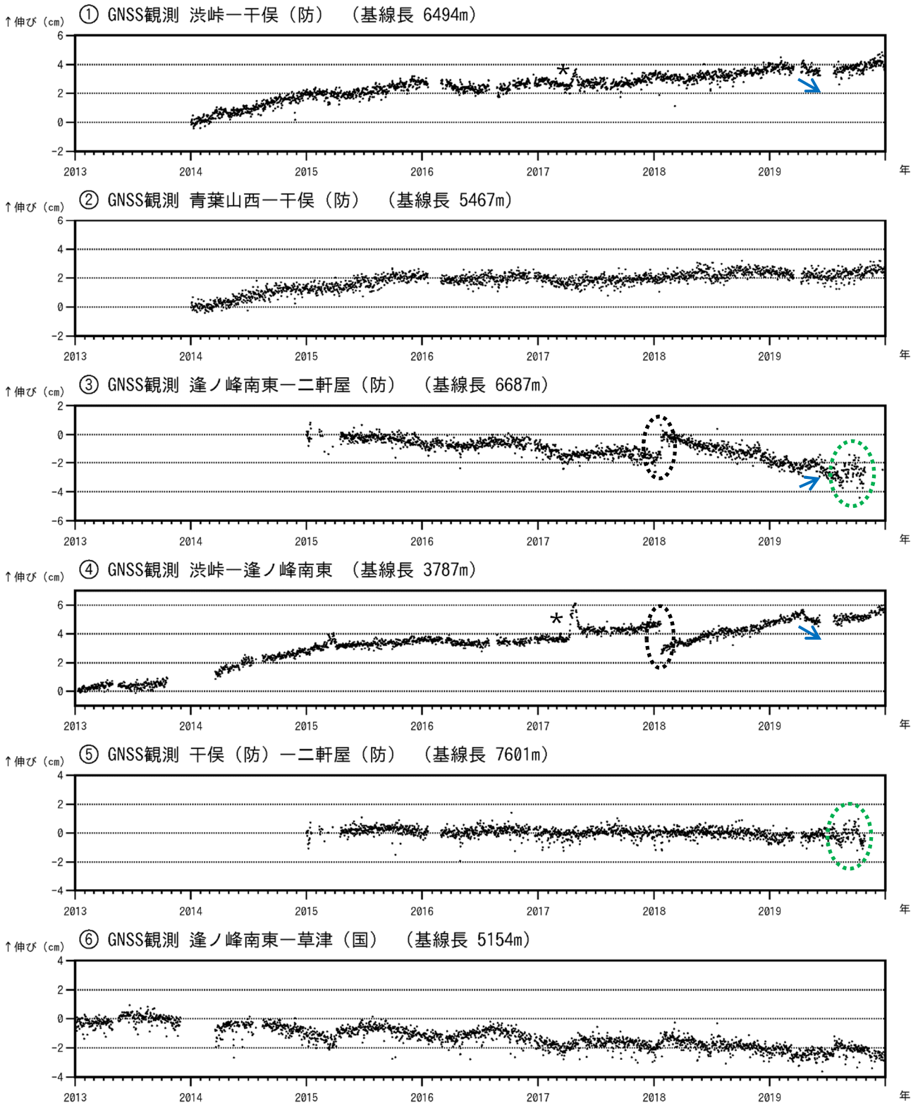
図9 草津白根山 GNSS連続観測の結果（2013年1月1日～2019年12月31日）
