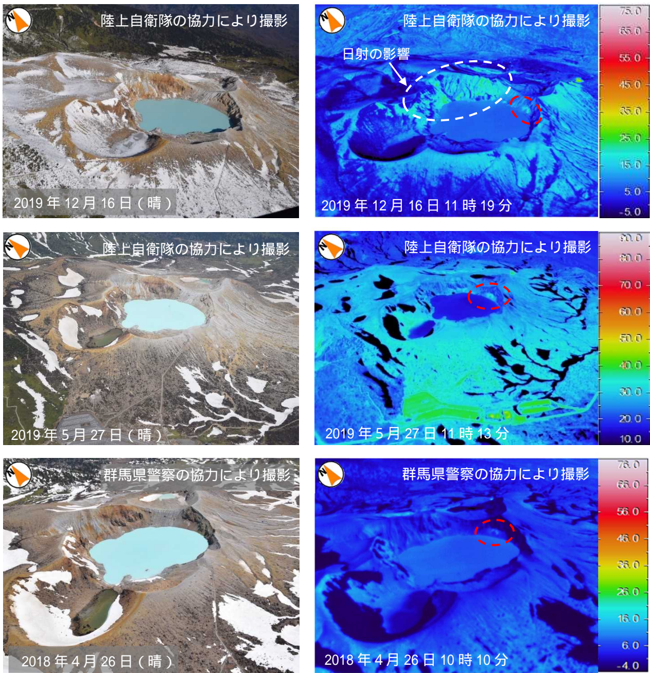
図2 草津白根山（白根山（湯釜付近）） 湯釜周辺の状況及び地表面温度分布
