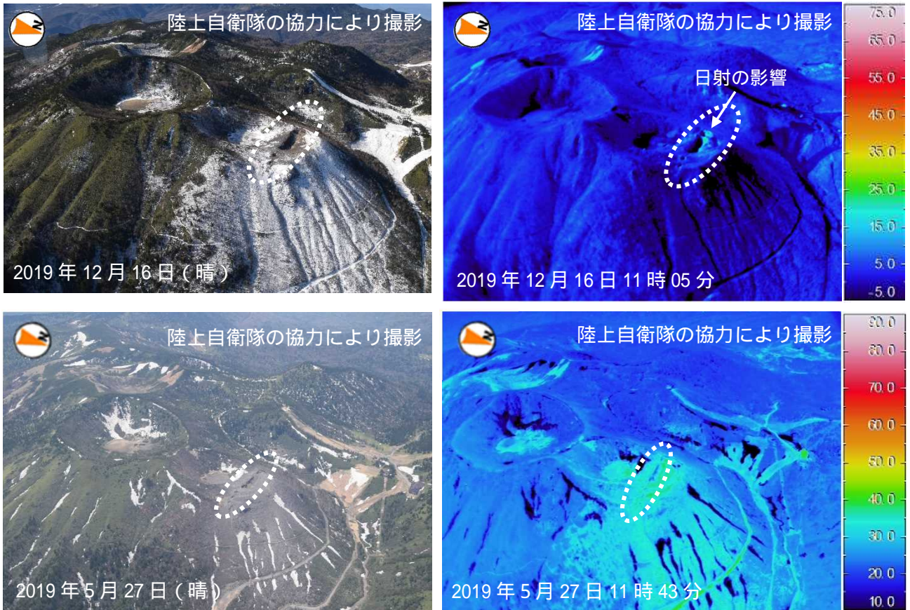
図 15 草津白根山(本白根山) 鏡池北火口北側の火口列と西側の火口の状況
