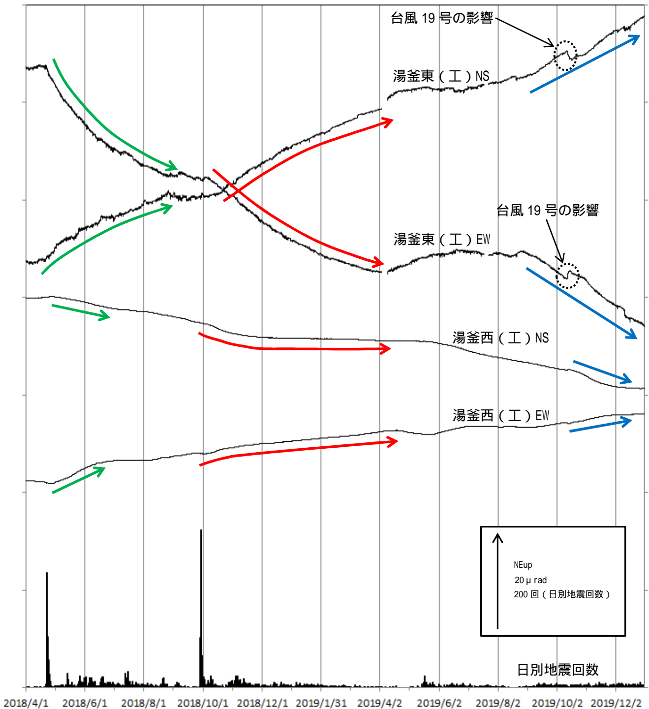
図 8 草津白根山（白根山（湯釜付近）） 傾斜変動（2018 年 4 月 1 日～2019 年 12 月 31 日）
