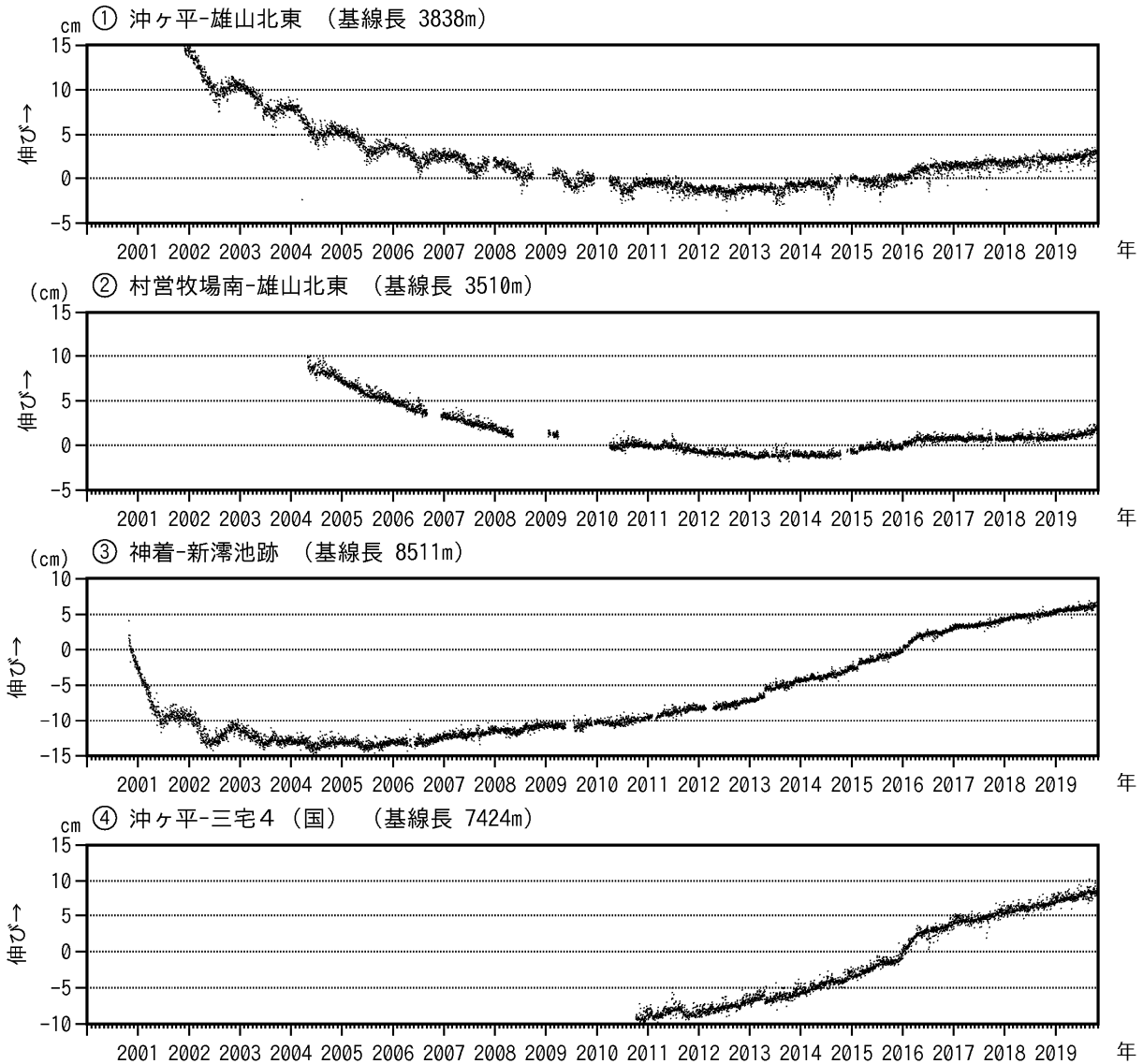
図7 三宅島 GNSS 連続観測結果(2000年10月26日~2019年10月31日)
