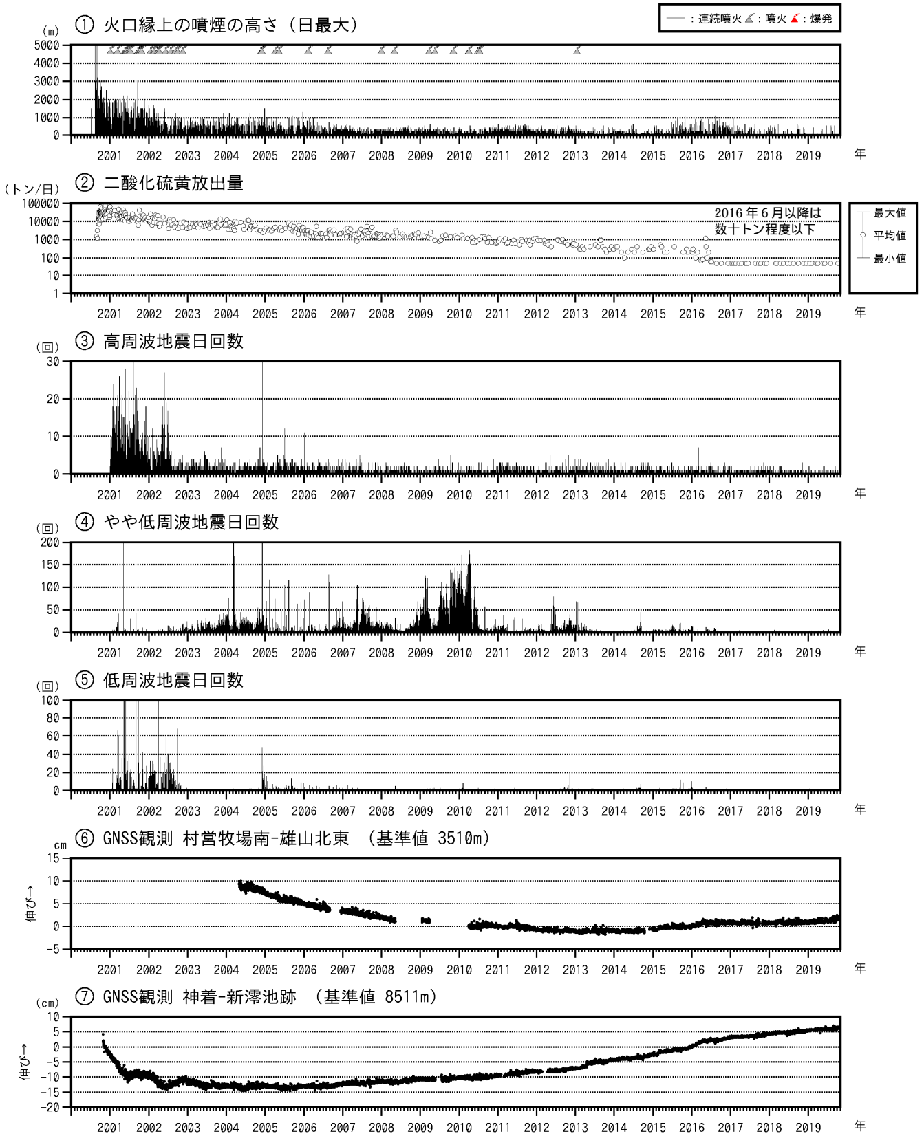
図5 三宅島 火山活動長期経過図（2000年1月1日～2019年10月31日）
