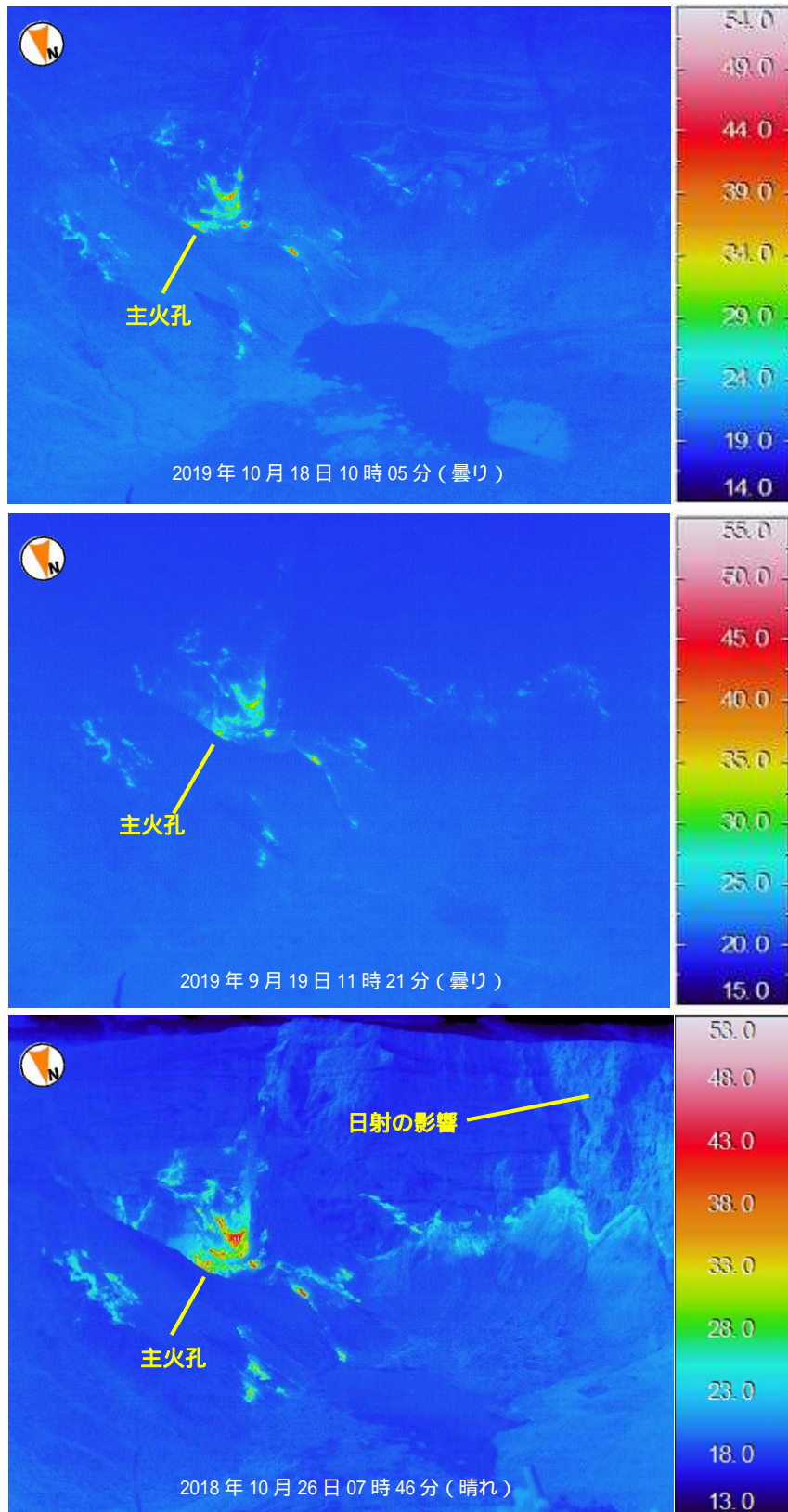
図4 三宅島 赤外熱映像装置による山頂火口内の地表面温度分布 18日に実施した現地調査では、9月や昨年と同様に主火孔内及びその周辺で引き続き高温領域が認められました。高温領域の分布に特段の変化は認められません。
