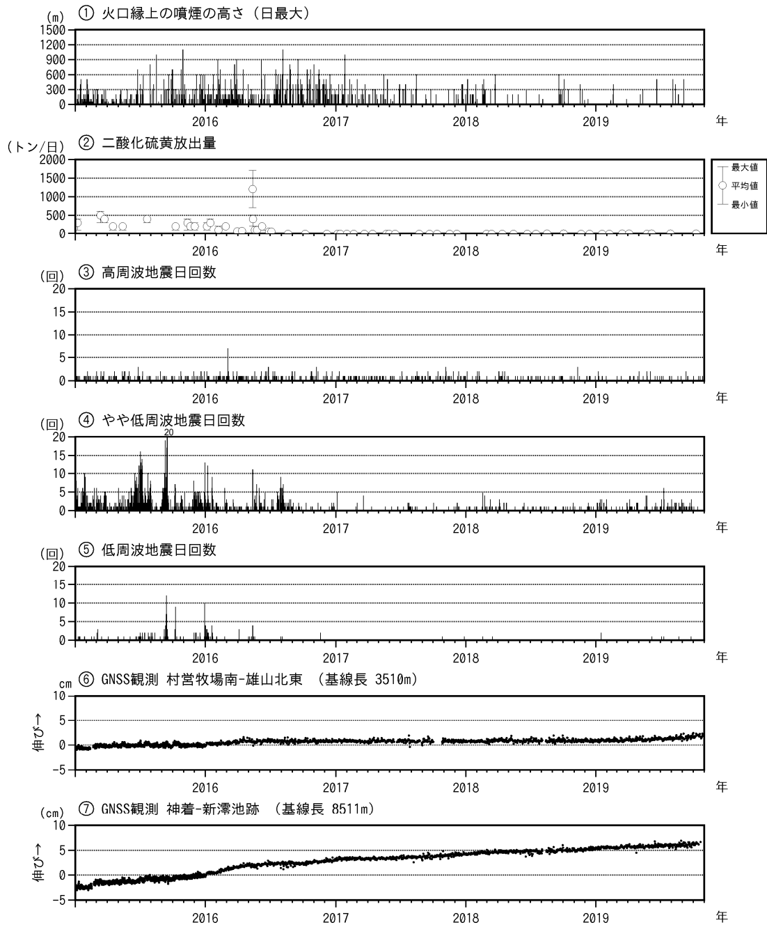
図 6 三宅島 火山活動短期経過図（2015 年 1 月 1 日～2019 年 10 月 31 日）
