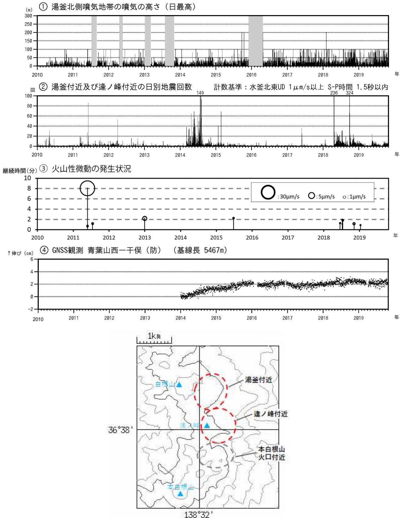
図3 草津白根山（白根山（湯釜付近））火山活動経過図（2010年1月1日～2019年10月31日） の灰色部分およびの空白部分は欠測を示します。 は図9のの基線に対応しています。 2013年1月に解析方法を変更しています。 最下段の図は、の地震の震源の概ねの位置を示しています。 ・GNSS連続観測では、火山活動によるとみられる変動は認められません。
