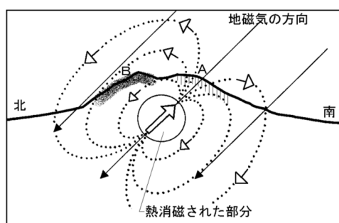
図 10 熱消磁に伴う全磁力変化のモデル
