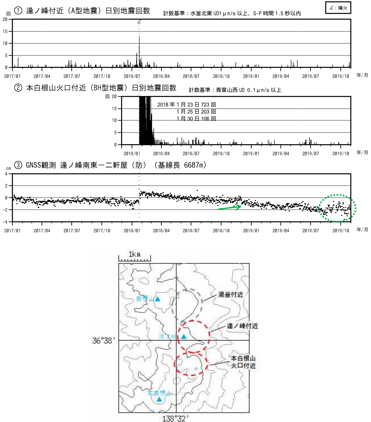
図 12 草津白根山（本白根山） 火山活動経過図（2017年1月1日～2019年10月31日）
