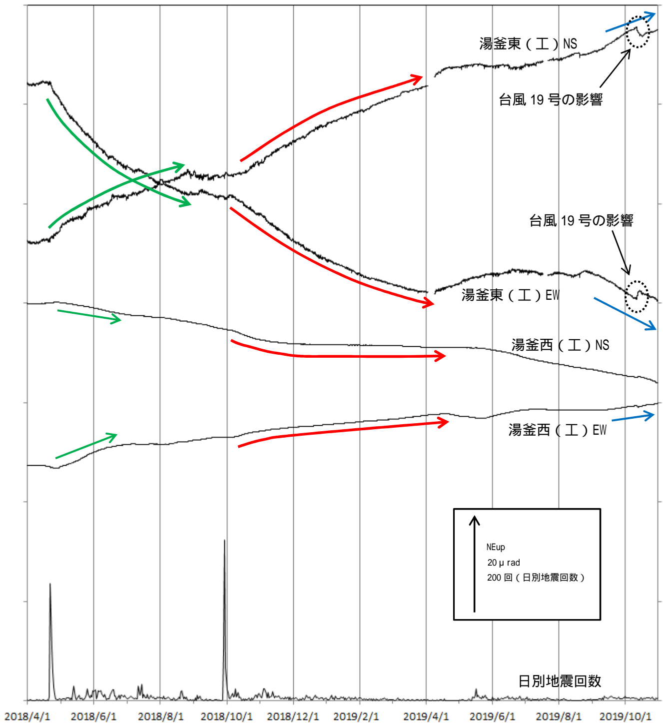
図5 草津白根山（白根山（湯釜付近））傾斜変動（2018年4月1日～2019年10月31日）
