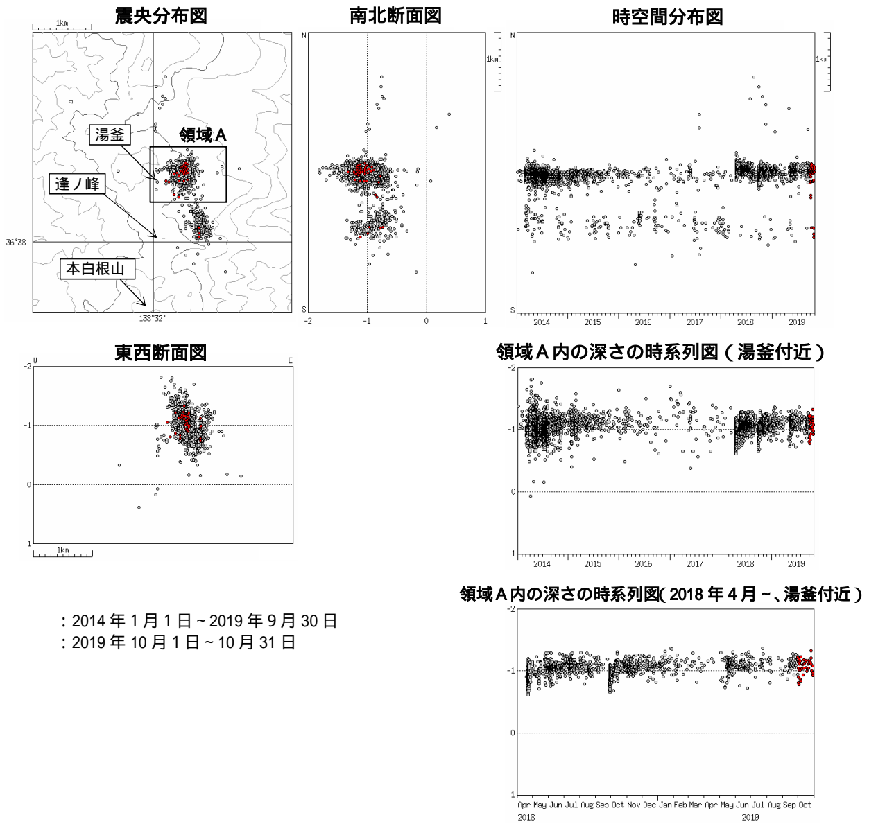
図4 草津白根山 震源分布図（2014年1月1日～2019年10月31日） 火山性地震の震源は、主に湯釜付近の海拔約1 km に分布しました。
