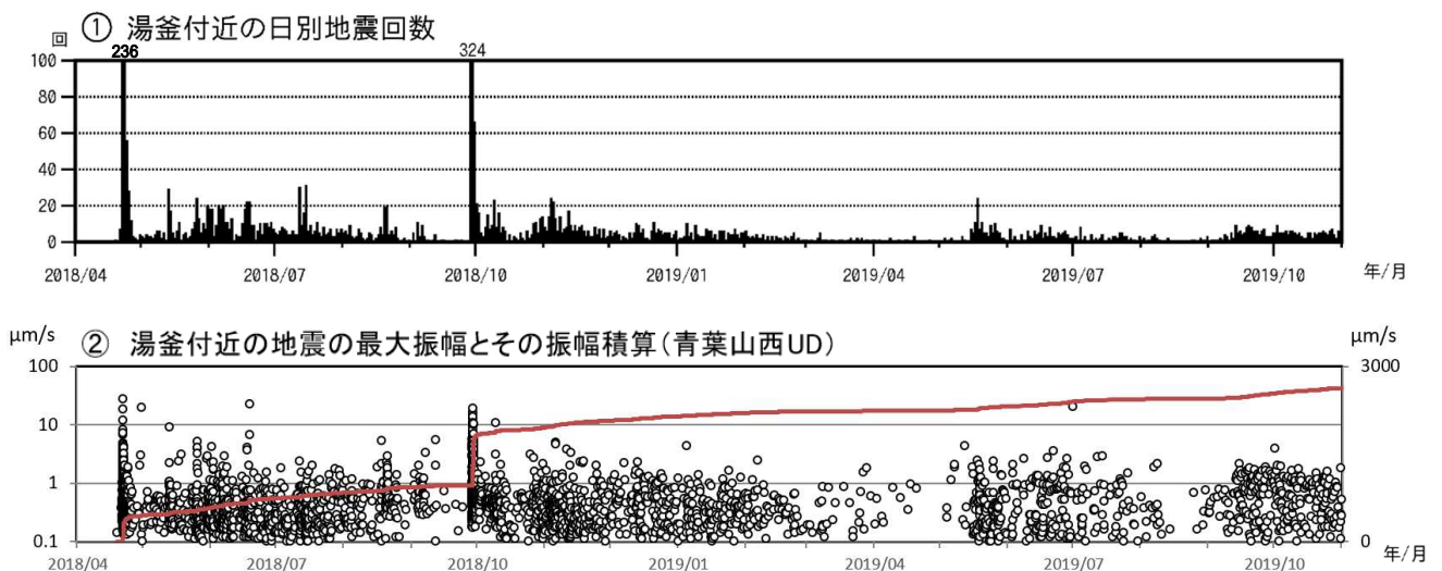
図2 草津白根山（白根山（湯釜付近）） 湯釜付近の地震活動（2018年4月1日～2019年10月31日） （○：最大振幅（左軸）、赤線：最大振幅の積算（右軸））
