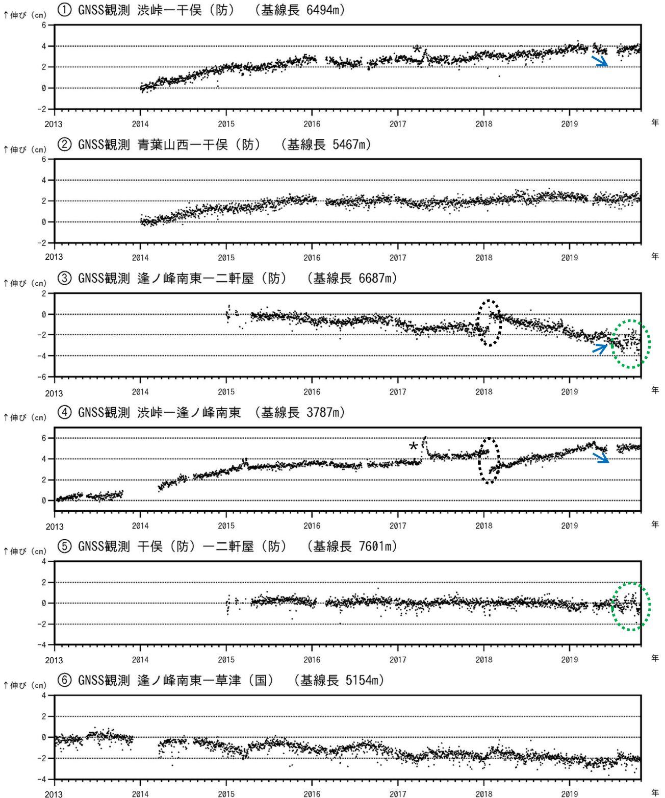
図6 草津白根山 GNSS連続観測の結果(2013年1月1日~2019年10月31日)
