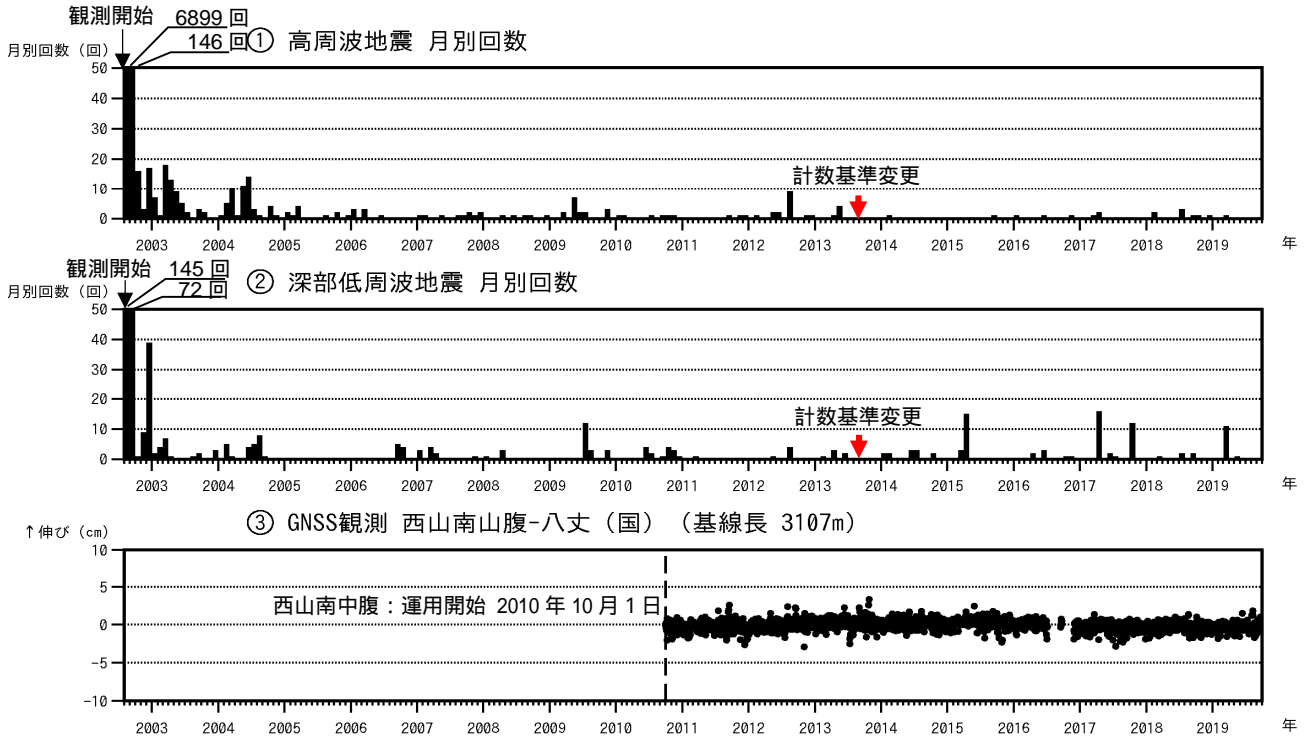
図2 八丈島 火山活動経過図（2002年8月13日～2019年9月30日）
