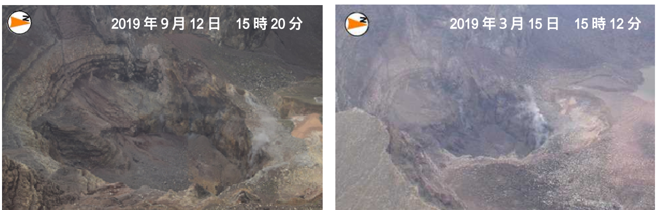
図4 三宅島 主火孔内の状況(陸上自衛隊の協力による) ・前回の観測(2019年3月15日)と比べて、主火孔内の地形等に特段の変化は認められません。
