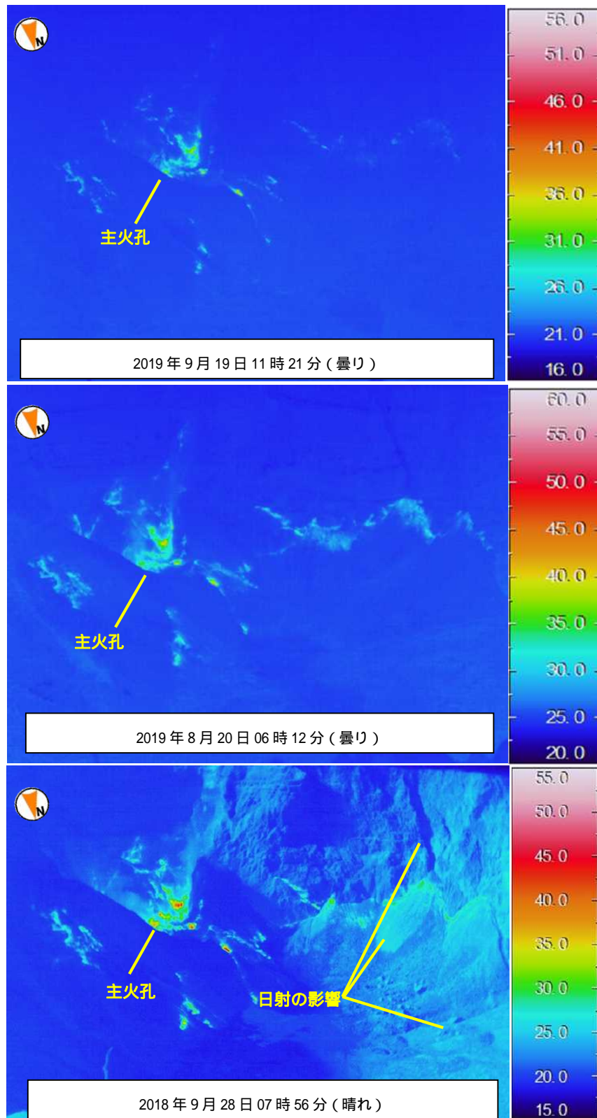
図7 三宅島 赤外熱映像装置による山頂火口内の地表面温度分布 19日に実施した現地調査では、8月や昨年と同様に主火孔内及びその周辺で引き続き地熱域が認められました。地熱域の分布に特段の変化は認められません。
