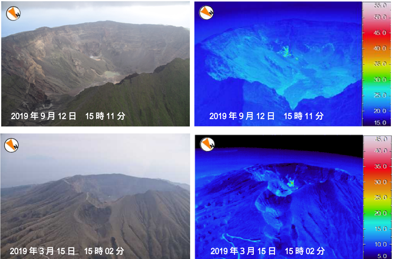
図3 三宅島 山頂火口の様子と赤外熱映像装置によるその地表面温度分布(陸上自衛隊の協力による) 上段：天気：薄曇り（高度約900mより撮影） 下段：天気：薄曇り（高度約1000mより撮影） 火口の地形及び主火孔付近の地熱の分布に特段の変化は認められません。
