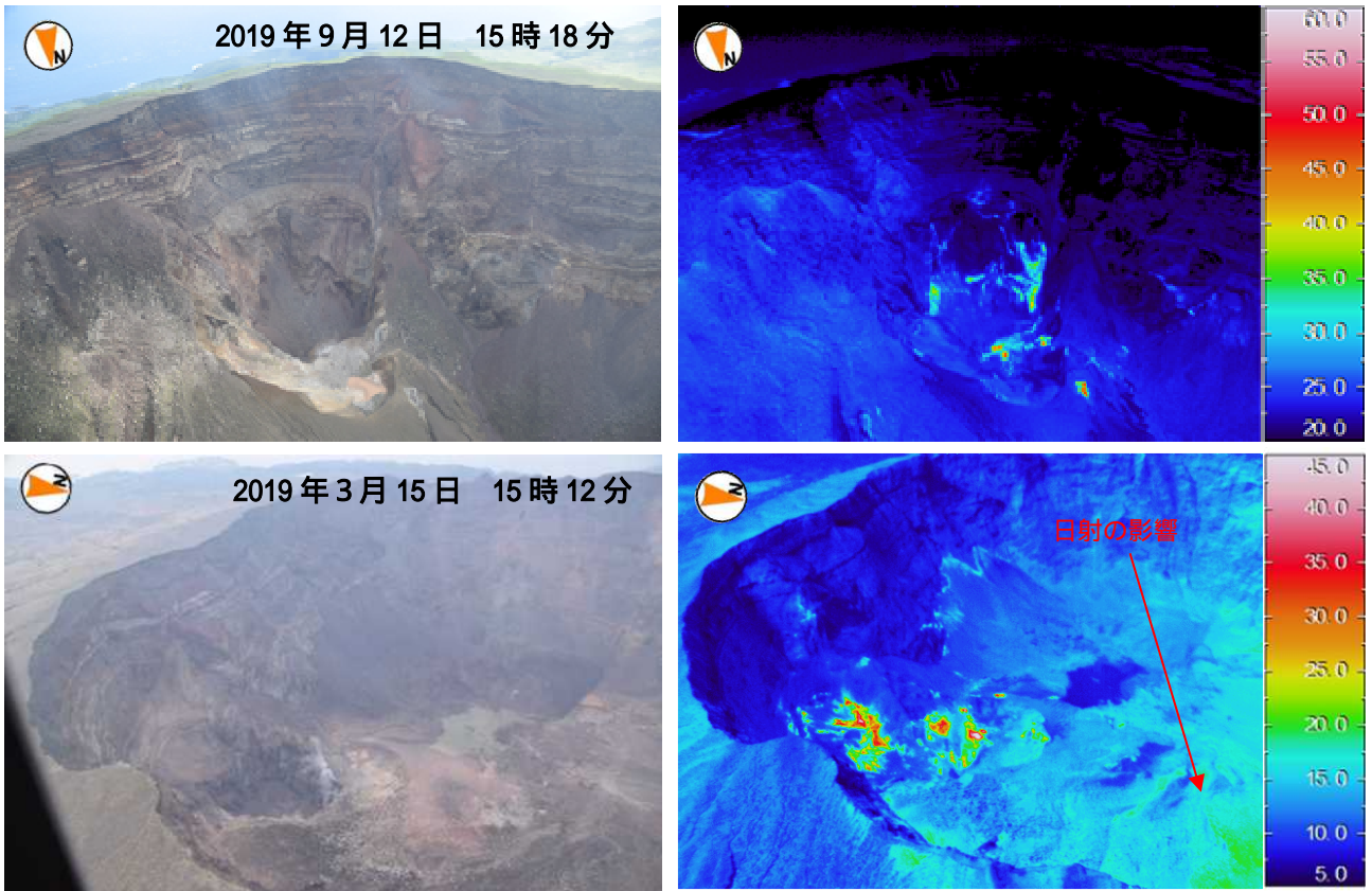
図5 三宅島 主火孔内の状況と赤外熱映像装置によるその地表面温度分布(陸上自衛隊の協力による) ・前回の観測(2019年3月15日)と比べて、主火孔内の地形及び地熱の分布に特段の変化は認められません。
