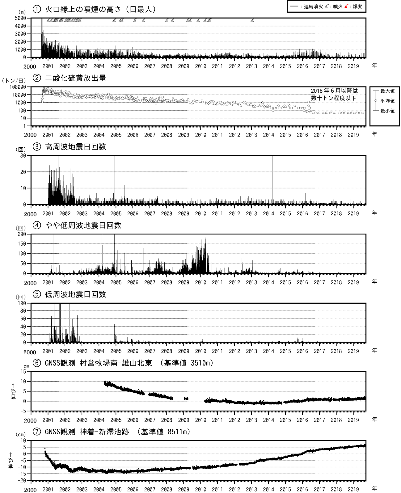
図8 三宅島 火山活動長期経過図（2000年1月1日～2019年9月30日）
