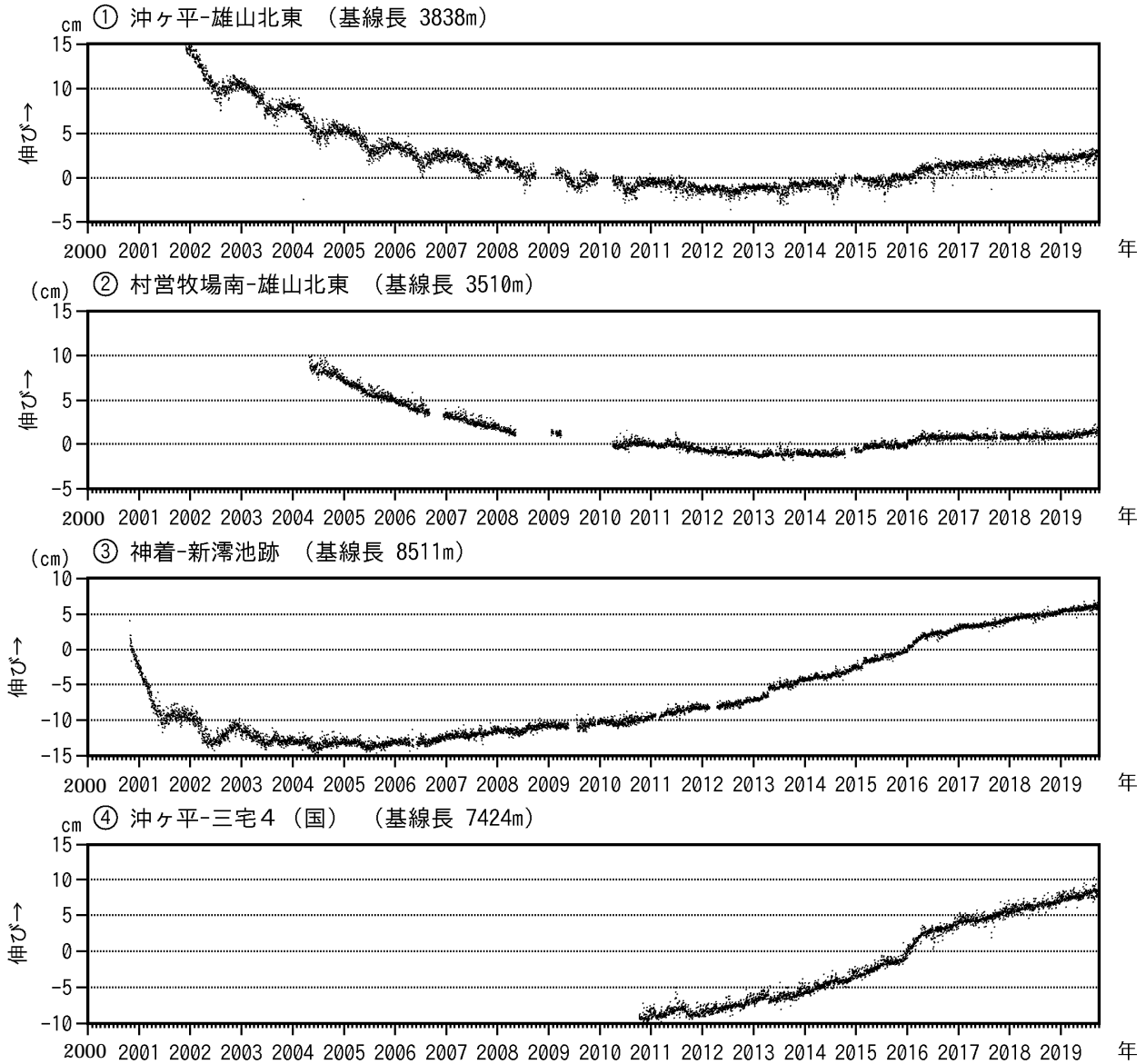
図10 三宅島 GNSS 連続観測結果（2000年10月26日～2019年9月30日）
