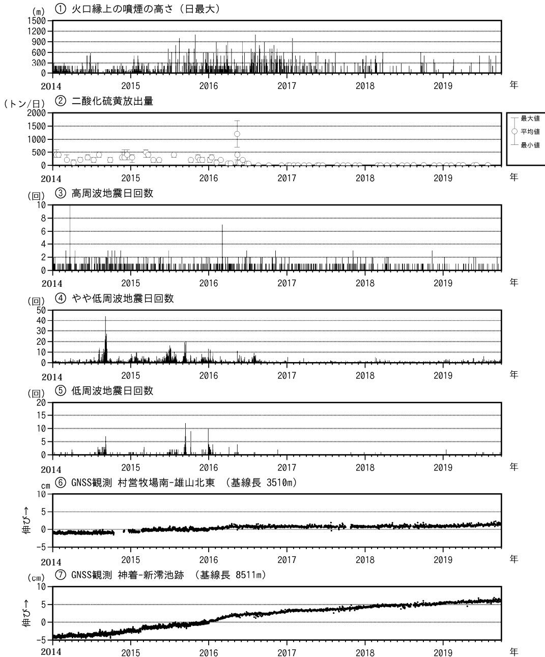
図9 三宅島 火山活動短期経過図（2014年1月1日～2019年9月30日）
