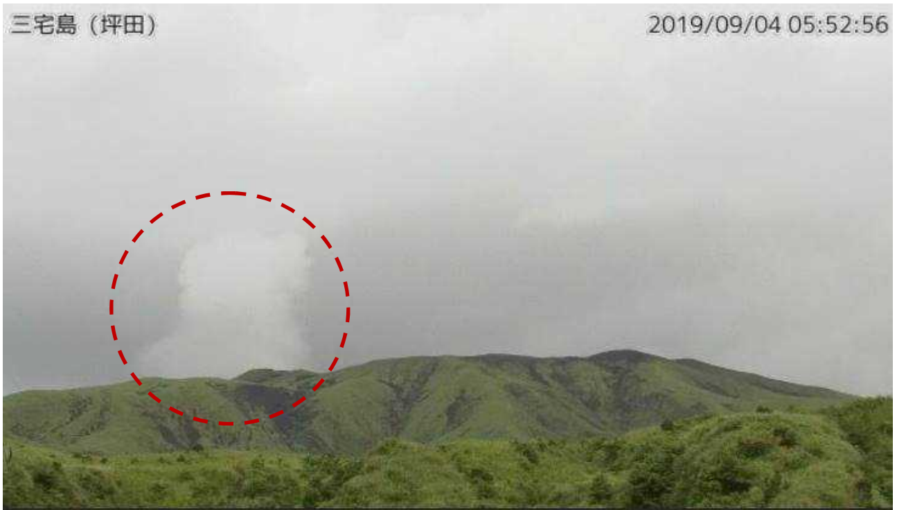
図1 三宅島 雄山山頂部の状況 坪田監視カメラ（9月4日）による。赤破線は噴煙を示す。
