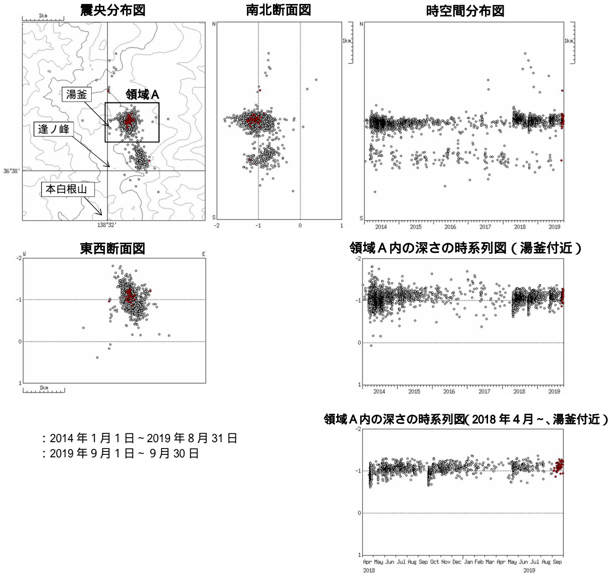
図6 草津白根山 震源分布図(2014年1月1日～2019年9月30日) 火山性地震の震源は、主に湯釜付近の海拔約1 kmに分布しました。
