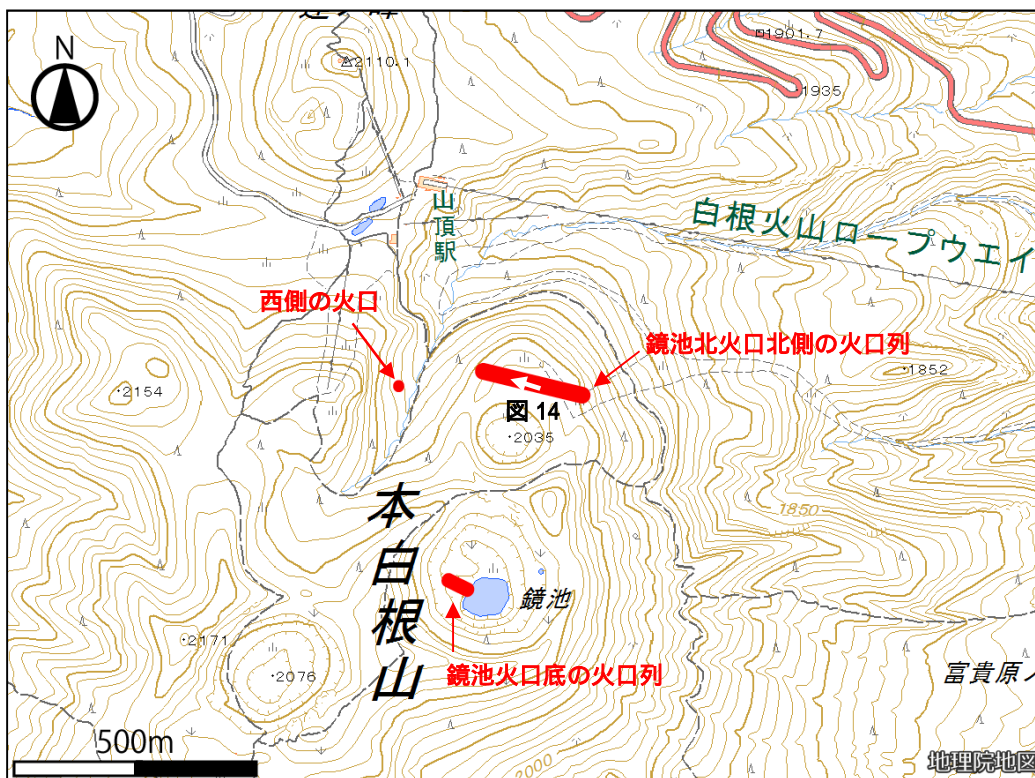
図15 草津白根山（本白根山） 本白根山周辺図 ・赤丸及び赤線は火口を示す。 ・白丸及び白矢印は、図14の撮影位置と撮影方向を示します。
