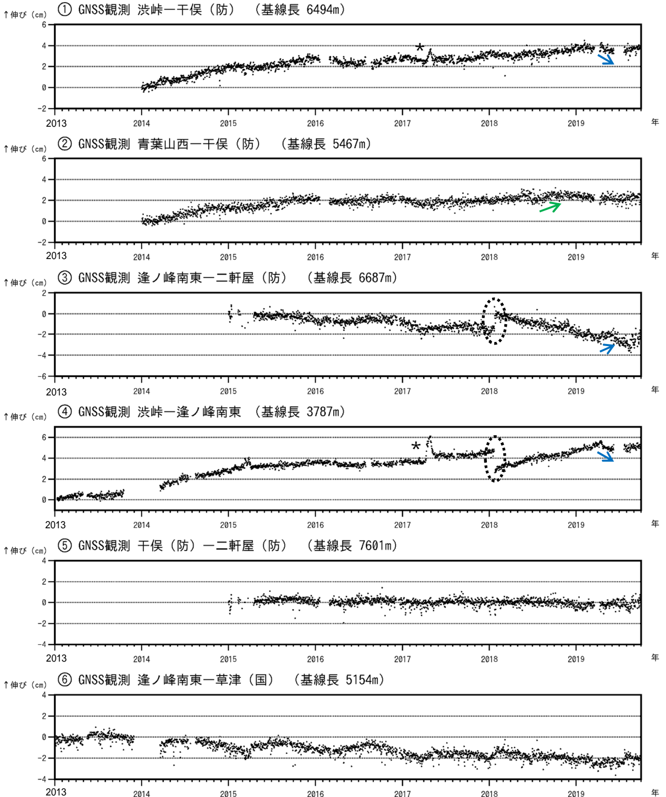
図8 草津白根山 GNSS連続観測の結果（2013年1月1日～2019年9月30日）
