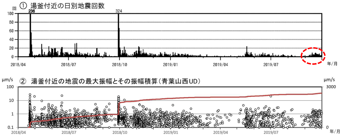
図4 草津白根山（白根山（湯釜付近）） 湯釜付近の地震活動（2018年4月1日～2019年9月30日） （○：最大振幅（左軸） 赤線：最大振幅の積算（右軸）） ・湯釜付近を震源とする火山性地震は、9月上旬頃からやや増加しています（赤破線）。振幅の大きな火山性地震は発生していません。
