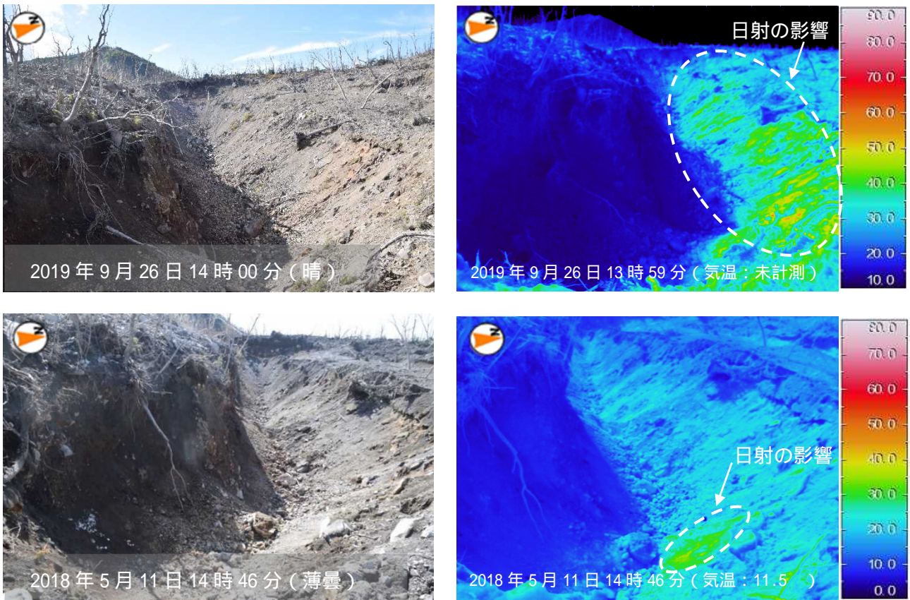
図14 草津白根山（本白根山） 鏡池北火口北側の火口列の状況 ・26日に実施した現地調査では、前回（2018年5月11日）の観測に引き続き、鏡池北火口北側の火口内に噴気や日射の影響を超えるような地熱域は認められませんでした。
