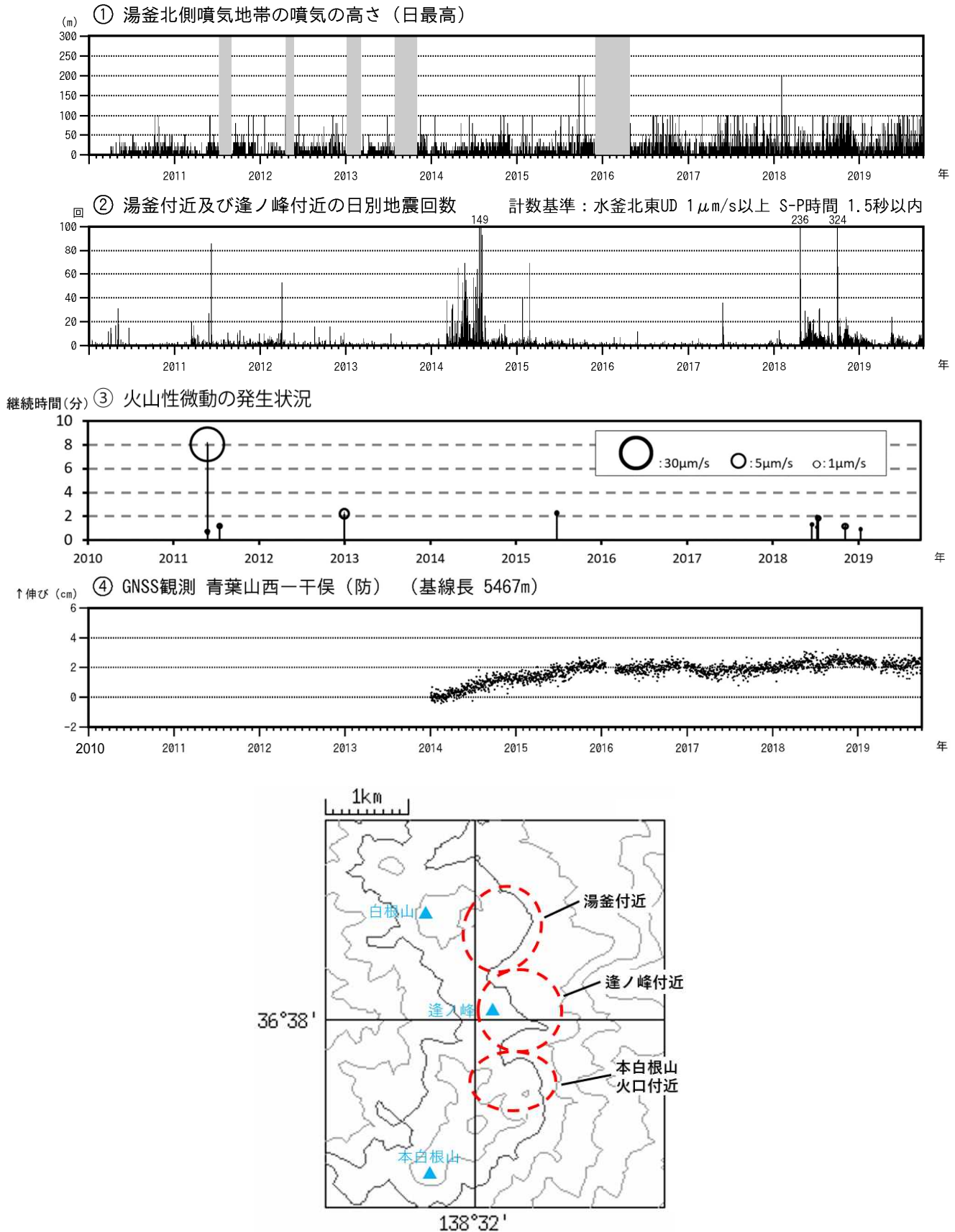
図5 草津白根山（白根山（湯釜付近））火山活動経過図（2010年1月1日～2019年9月30日） の灰色部分およびの空白部分は欠測を示します。 は図9のの基線に対応しています。 2013年1月に解析方法を変更しています。 最下段の図は、の地震の震源の概ねの位置を示しています。 ・GNSS連続観測では、火山活動によるとみられる変動は認められません。
