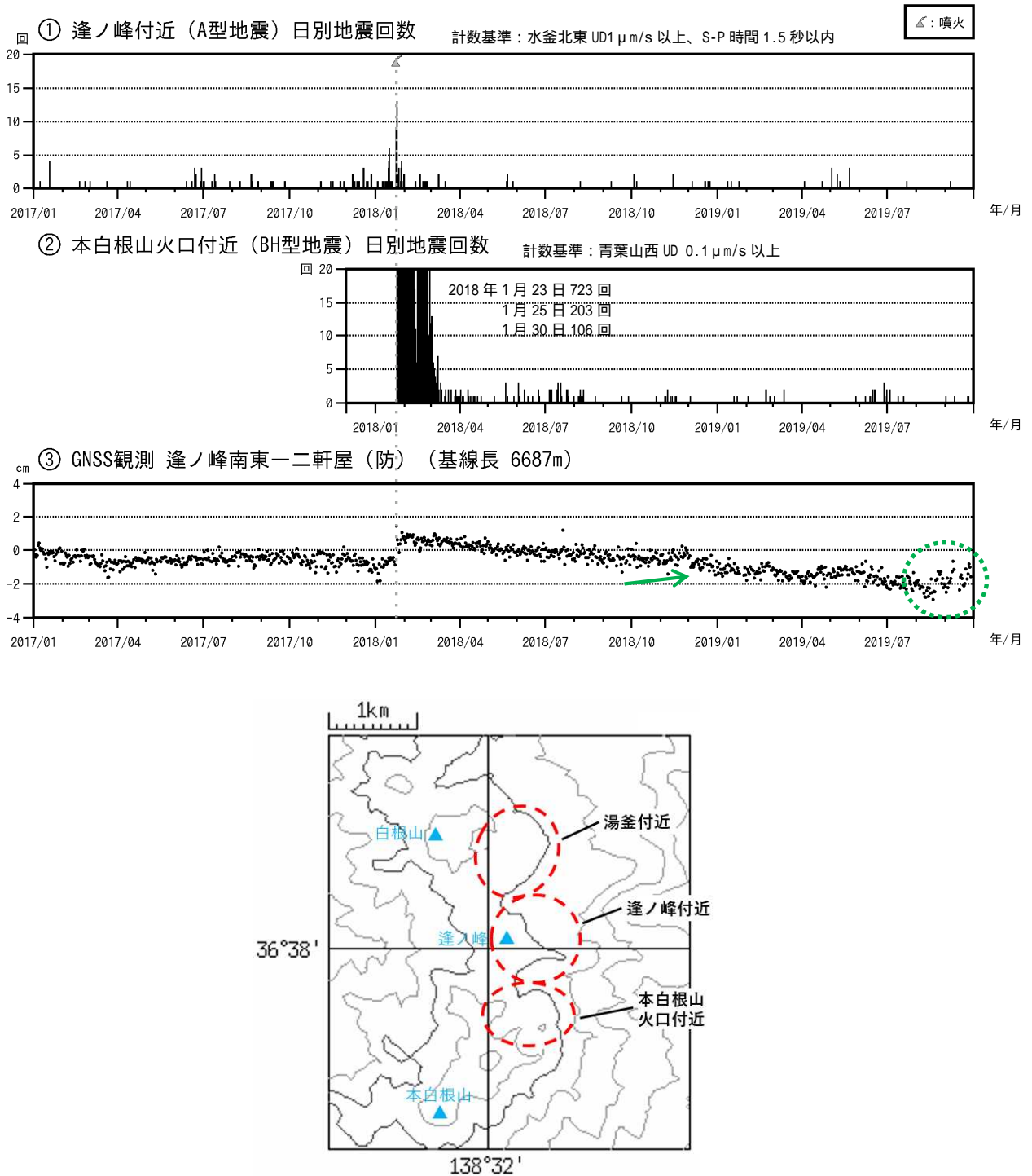
図 16 草津白根山（本白根山） 火山活動経過図（2017年1月1日～2019年9月30日） 草津白根山では、火山性地震はその発生領域から、「湯釜付近」、「逢ノ峰付近」、「本白根山火口付近」に分けています。本白根山の火山活動については、逢ノ峰付近と本白根山火口付近の地震活動に注目して監視しています。火山性地震の種類については図 17 を参照してください。 は図 9 の の基線に対応しています。 最下段の図は、 の地震の震源の概ねの位置を示しています。 ・ 逢ノ峰付近の火山性地震は、少ない状態で経過しています。 ・ 噴火発生後、本白根山火口付近で BH 型の火山性地震が多発しましたが、12 月以降、少ない状態で経過しています。なお、BH 型地震は、初動が不明瞭なため、震源は求まっていません。 ・ の基線で 2018 年 1 月以降にみられている変化は、本白根山の収縮によるものと考えられます。2018 年に、草津白根山の北西もしくは西側深部の膨張を示唆する変化がみられていました（緑矢印）。 ・ の基線で 2019 年 8 月頃からみられている変化（緑破線）は、火山活動によるものではないと考えられます。
