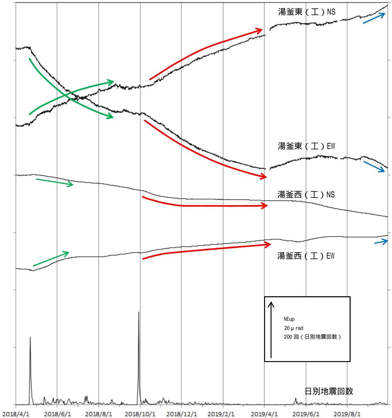
図7 草津白根山（白根山（湯釜付近）） 傾斜変動（2018年4月1日～2019年9月30日）
