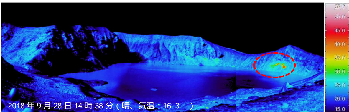
図2 草津白根山（白根山（湯釜付近）） 湯釜火口内の状況
