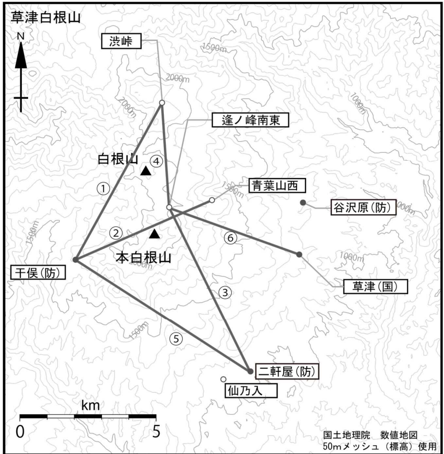
図9 草津白根山 GNSS 観測点配置図
