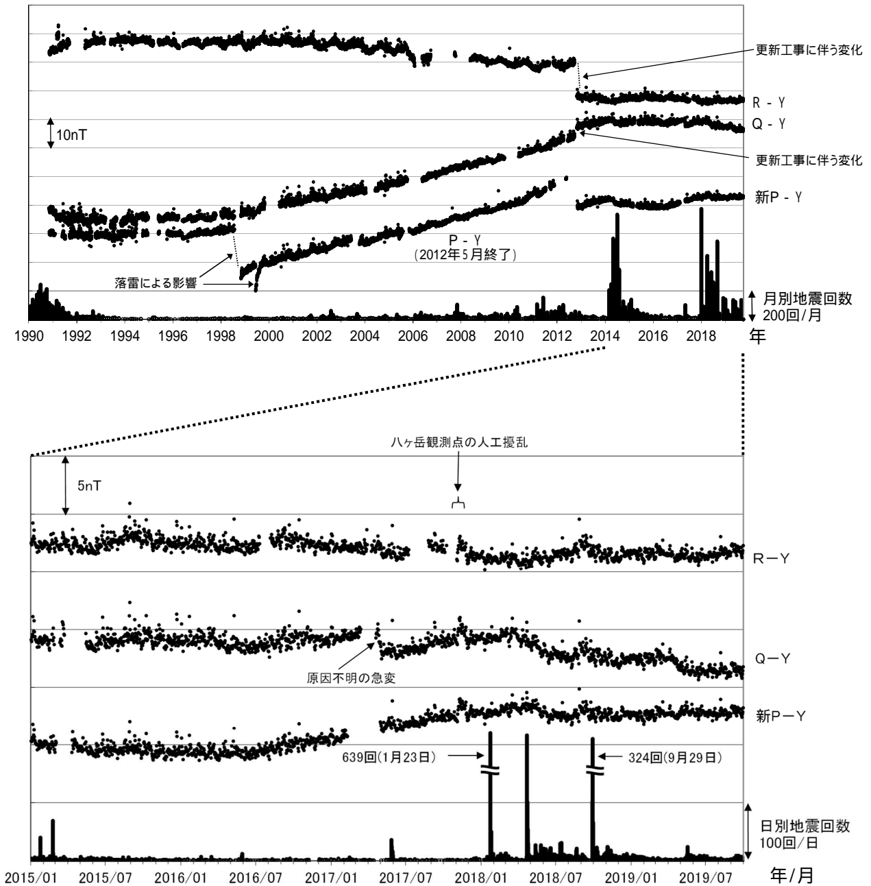
図 10 草津白根山（白根山（湯釜付近））全磁力連続観測による全磁力値の変化及び地震回数
