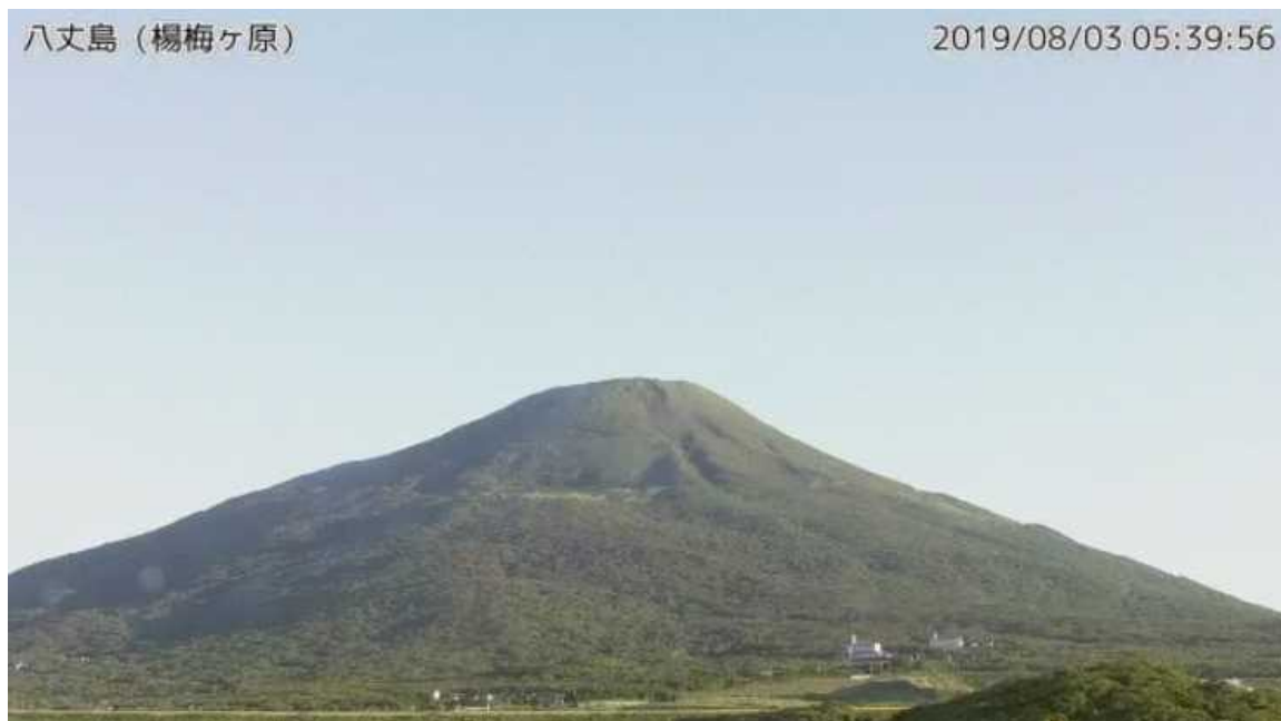
図1 八丈島 西山山頂部の状況 （8月3日、楊梅ヶ原 ようめがはら 監視カメラによる）
