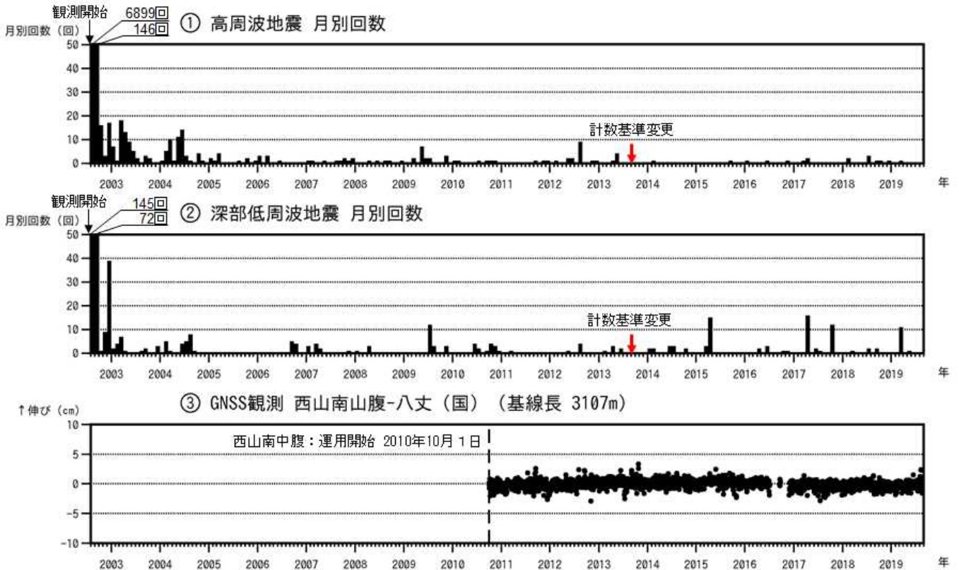
図2 八丈島 火山活動経過図（2002年8月13日～2019年8月31日）
