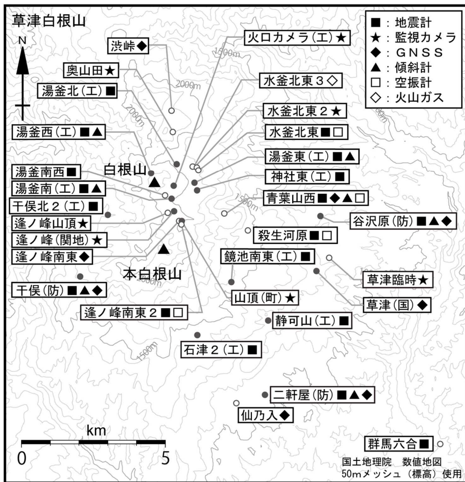
図 16 草津白根山 観測点配置図
