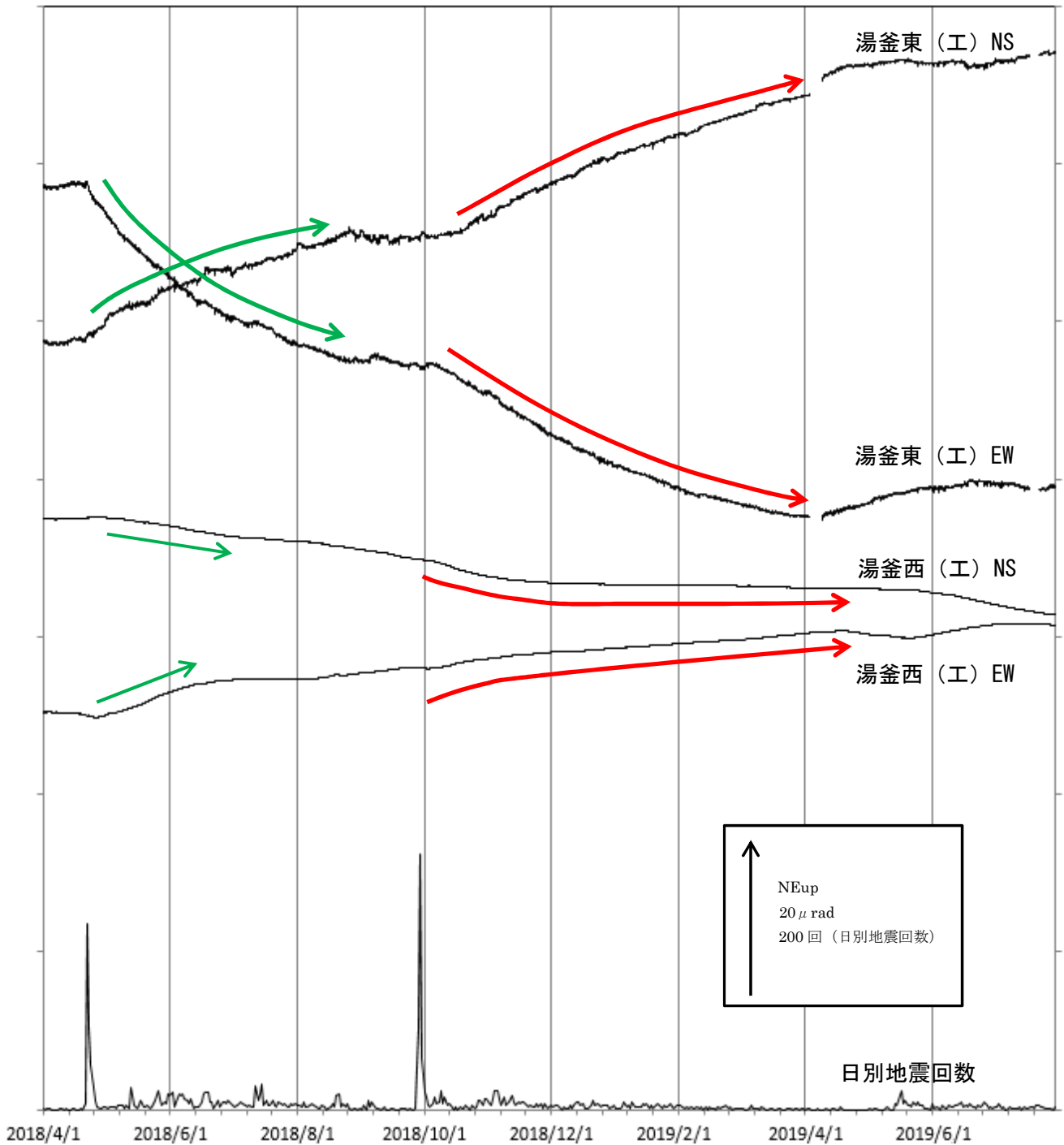
図 10 草津白根山（白根山（湯釜付近）） 傾斜変動（2018年4月1日～2019年7月31日） (工)：東京工業大学
