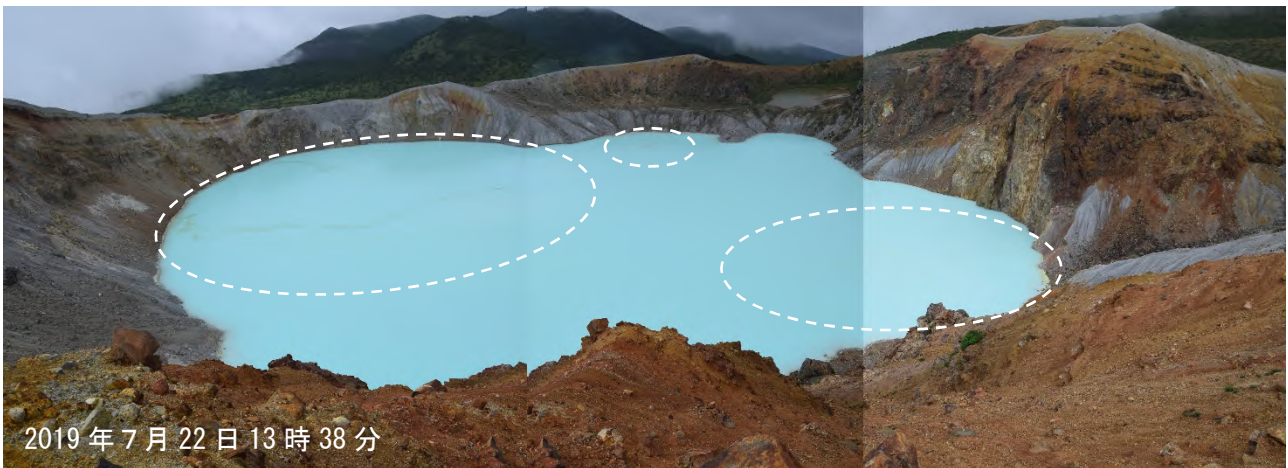
図3 草津白根山（白根山（湯釜付近）） 湯釜火口の状況 ・7月22日に実施した現地調査では、湯釜の湖面に変色域（白破線内）があることを確認しましたが、6月30日から7月1日にかけて観測された明瞭な変色域は認められませんでした。
