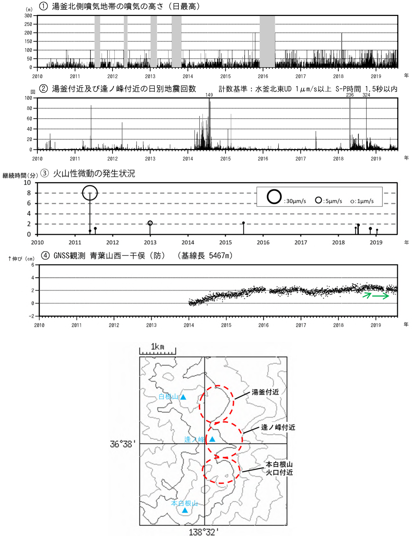
図8 草津白根山（白根山（湯釜付近））火山活動経過図（2010年1月1日～2019年7月31日）
