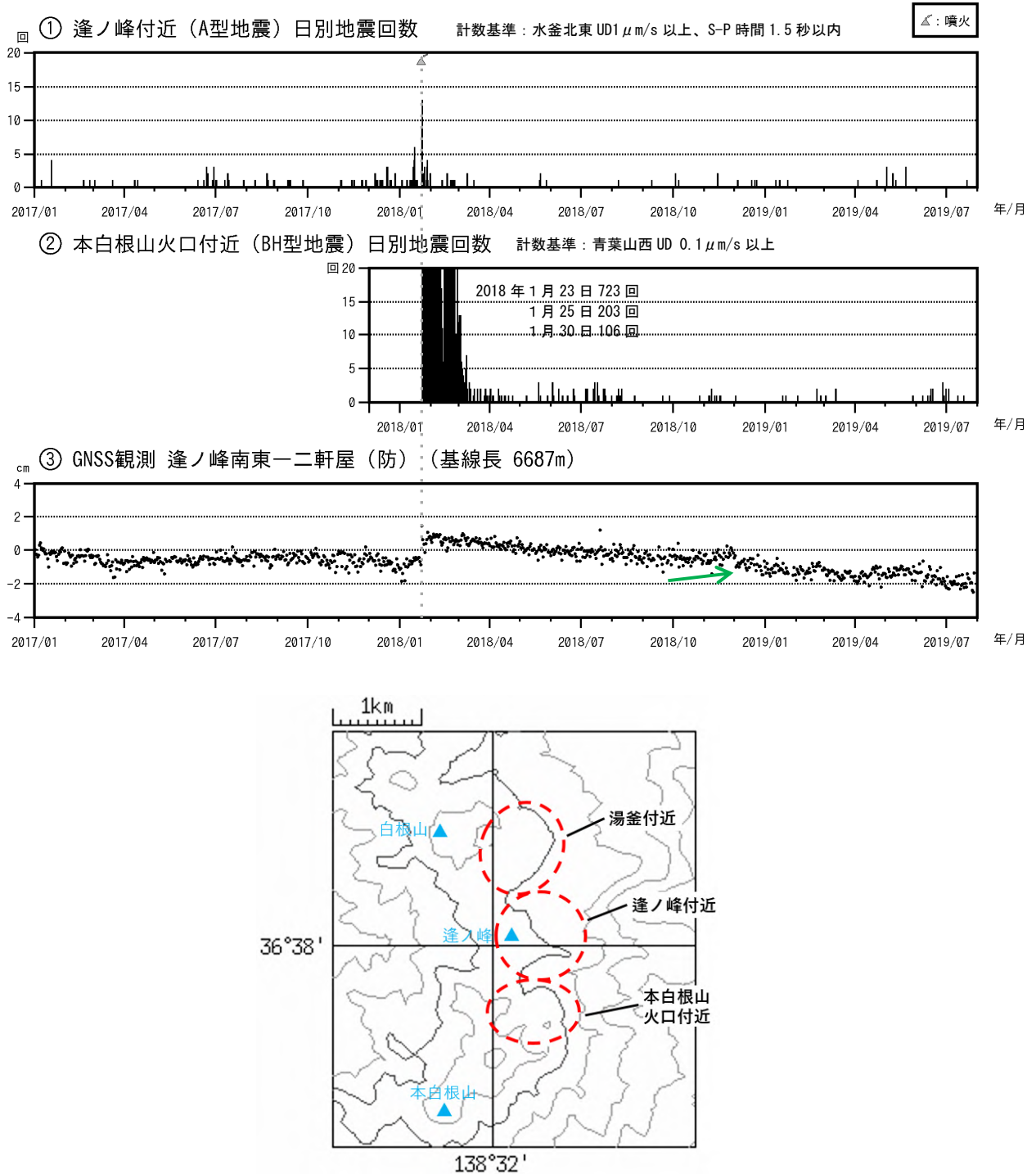
図 17 草津白根山（本白根山） 火山活動経過図（2017年1月1日～2019年7月31日）
