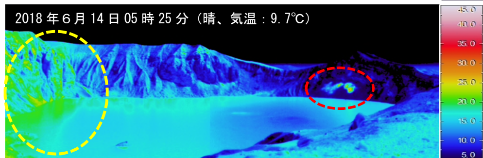
図4 草津白根山（白根山（湯釜付近）） 湯釜火口内壁の状況
