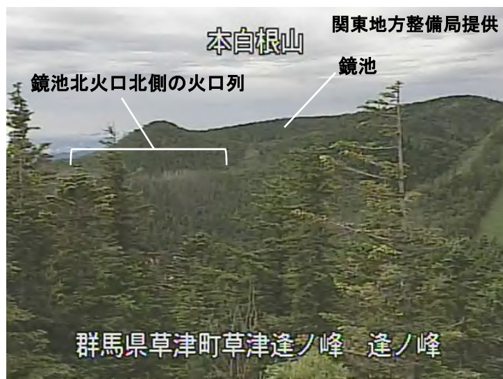
図16 草津白根山（本白根山） 本白根山付近の状況（7月20日、逢ノ峰監視カメラ）
