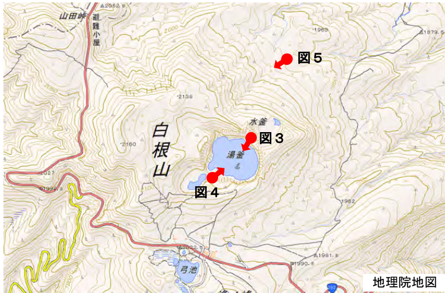
図2 草津白根山（白根山（湯釜付近）） 湯釜周辺図 ・赤丸及び赤矢印は、図3～5の撮影位置と撮影方向を示します。
