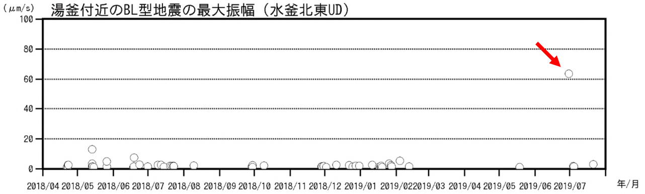
図6 草津白根山（湯釜付近） 湯釜付近で発生した低周波地震の振幅時系列図 （2018年4月1日～2019年7月31日） ・6月30日に湯釜付近が震源と推定される振幅の大きな低周波地震（赤矢印）が発生しました。その後も振幅の小さな低周波地震が時々発生しています。
