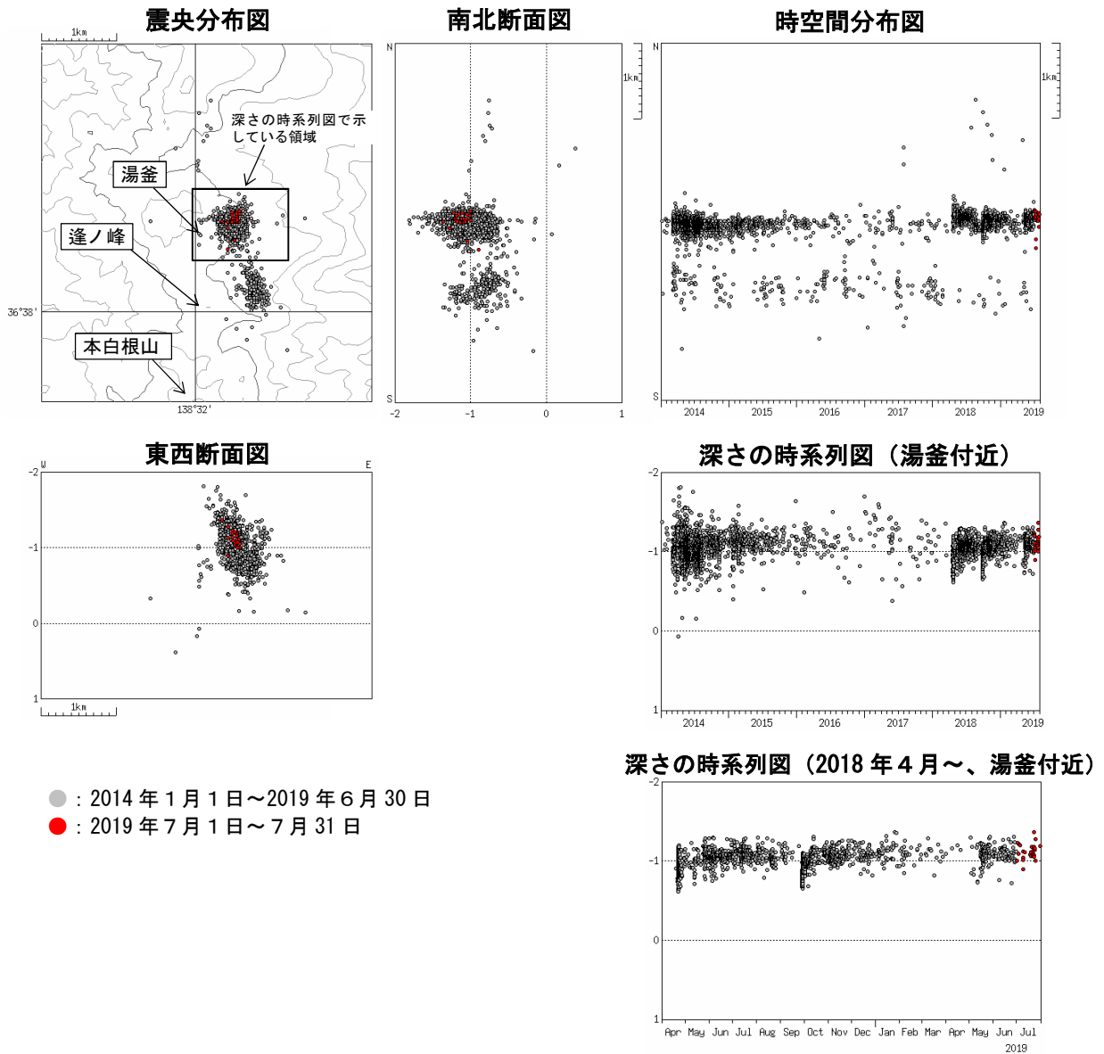
図9 草津白根山 震源分布図（2014年1月1日～2019年7月31日） 火山性地震の震源は、主に湯釜付近の海拔約1 kmに分布しました。
