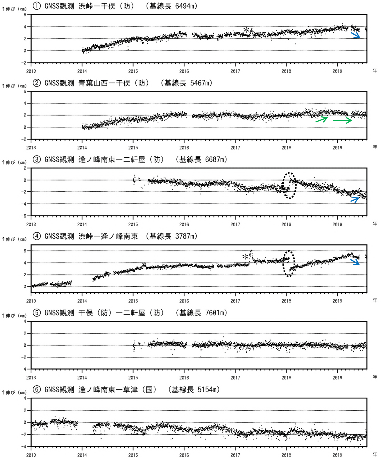
図 11 草津白根山 GNSS 連続観測の結果（2013 年 1 月 1 日～2019 年 7 月 31 日）
