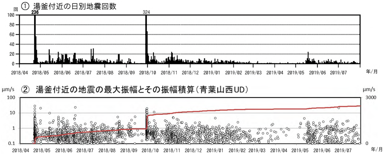
図7 草津白根山（白根山（湯釜付近）） 湯釜付近の地震活動（2018年4月1日～2019年7月31日） （○：最大振幅（左軸）、赤線：最大振幅の積算（右軸）） 湯釜付近を震源とする火山性地震は、5月中旬以降、増減を繰り返しながら推移しています。
