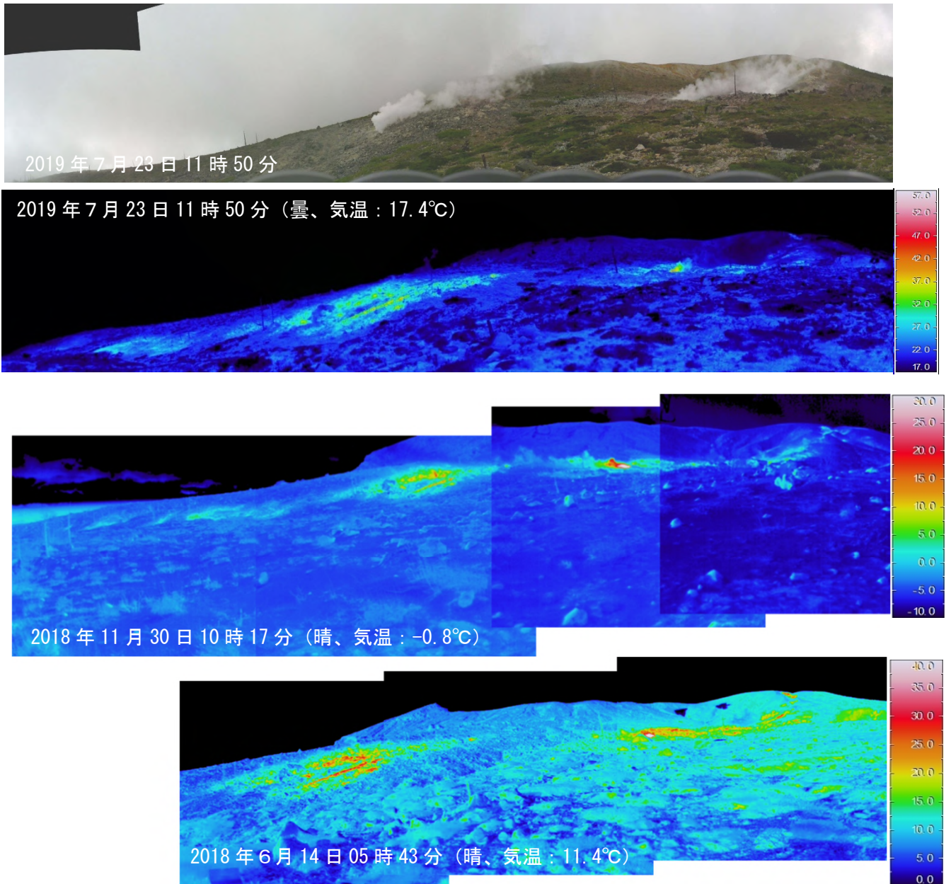
図5 草津白根山（白根山（湯釜付近）） 北側噴気地帯の状況
