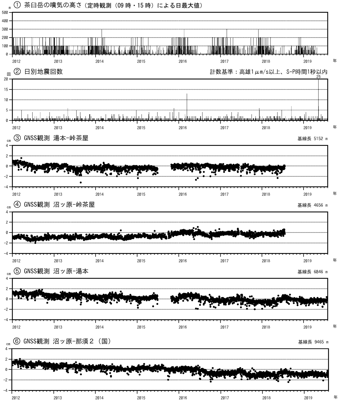
図4 那須岳 火山活動経過図（2012年1月1日～2019年7月31日）
