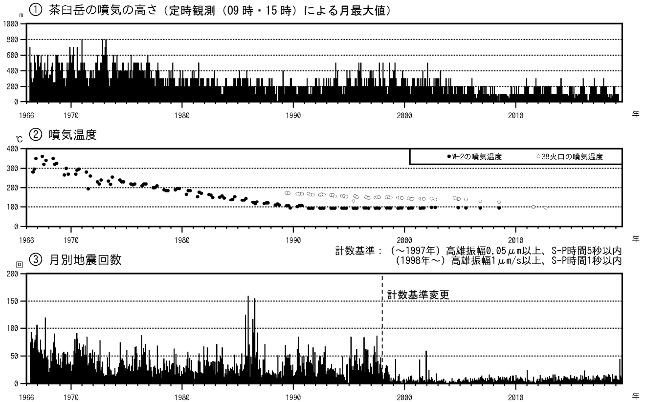
図3 那須岳 火山活動経過図（1966年1月～2019年7月）
