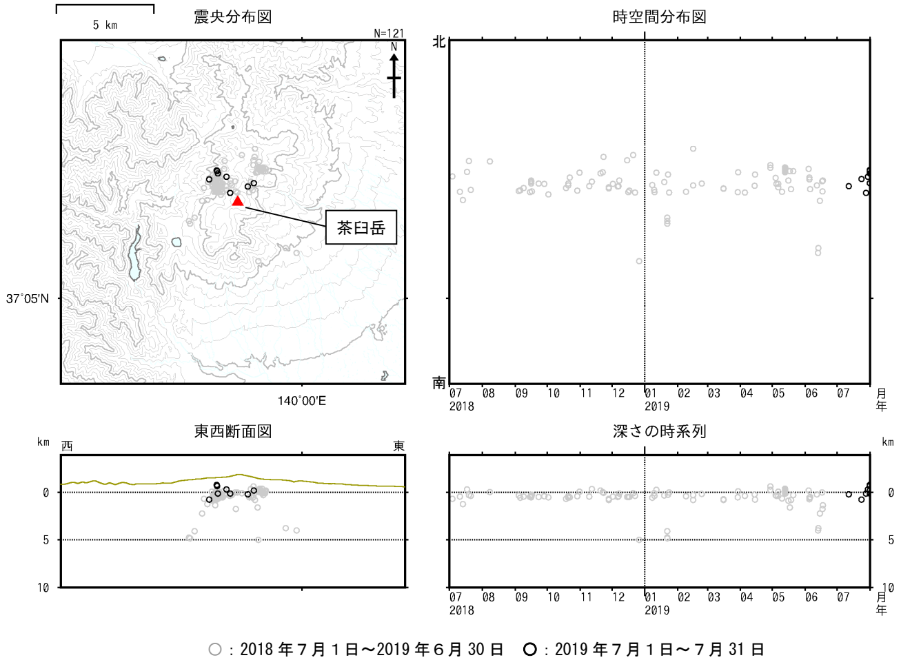
図5 那須岳 震源分布図（2018年7月1日～2019年7月31日）
