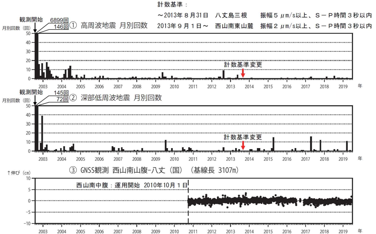
図2 八丈島 火山活動経過図（2002年8月13日～2019年6月30日）
