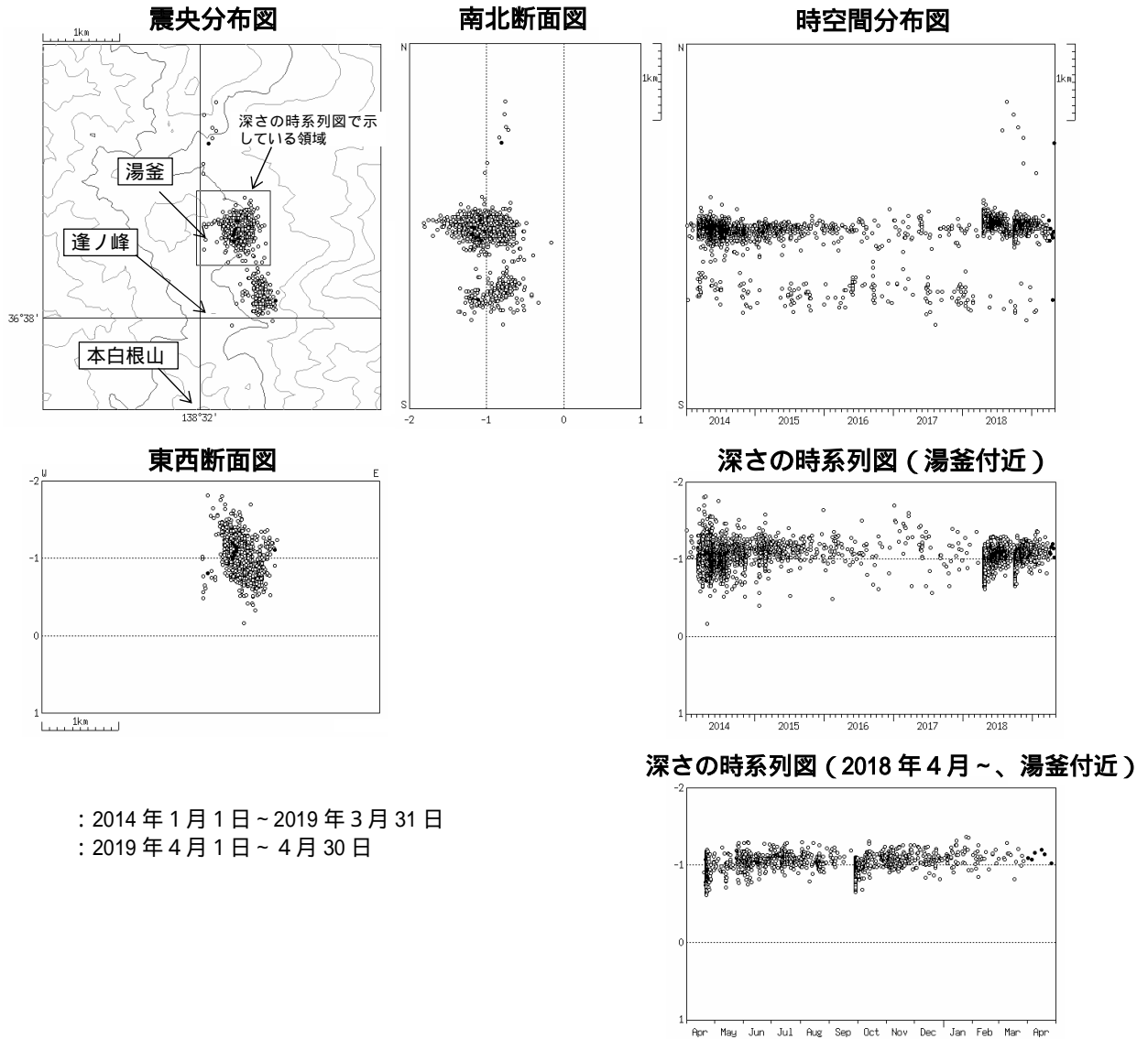
図5 草津白根山 震源分布図（2014年1月1日～2019年4月30日） 火山性地震の震源は、主に湯釜付近の海拔約1kmに分布しました。
