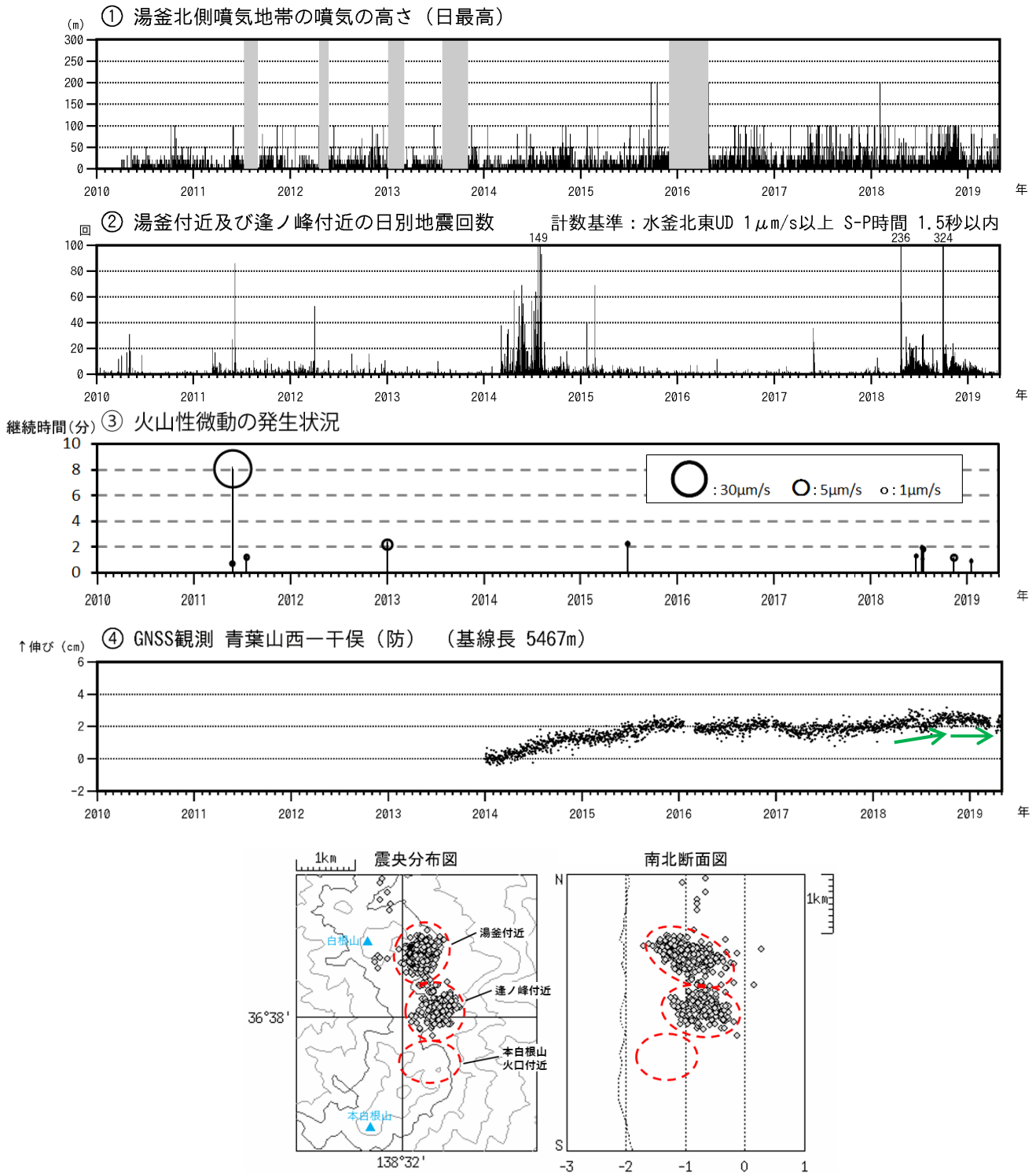
図4 草津白根山（白根山（湯釜付近））火山活動経過図（2010年1月1日～2019年4月30日）の灰色部分およびの空白部分は欠測を示します。
