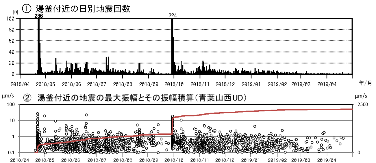
図2 草津白根山(白根山(湯釜付近)) 湯釜付近の地震活動(2018年4月1日~2019年4月30日) (○:最大振幅(左軸)、赤線:最大振幅の積算(右軸)) 湯釜付近を震源とする火山性地震は、2019年3月以降、概ね少ない状態で経過しています。
