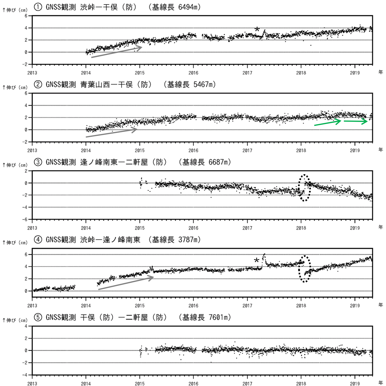
図7 草津白根山 GNSS連続観測の結果(2013年1月1日~2019年4月30日)
