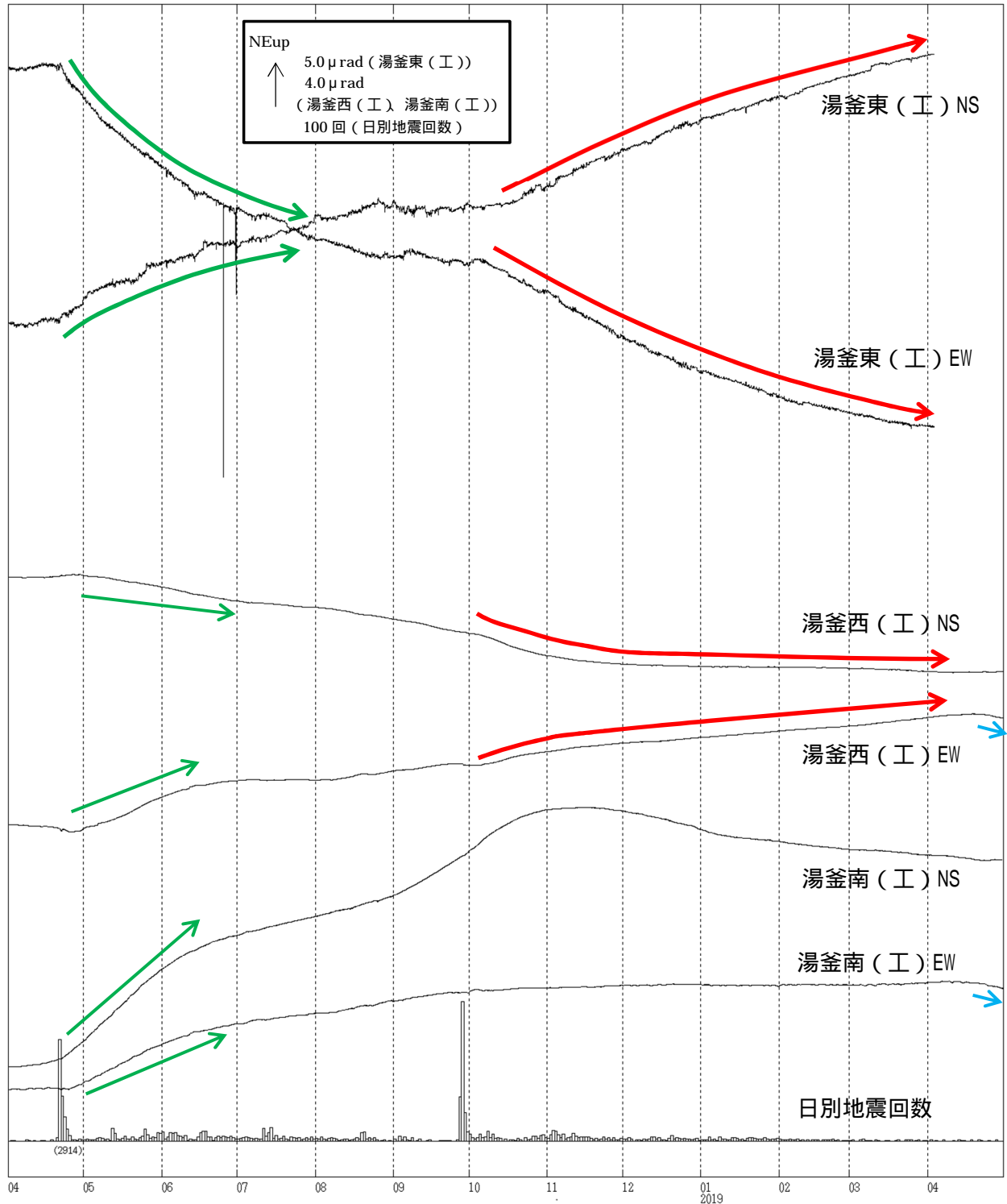
図3 草津白根山（白根山（湯釜付近）） 傾斜変動（2018年4月1日～2019年4月30日）
