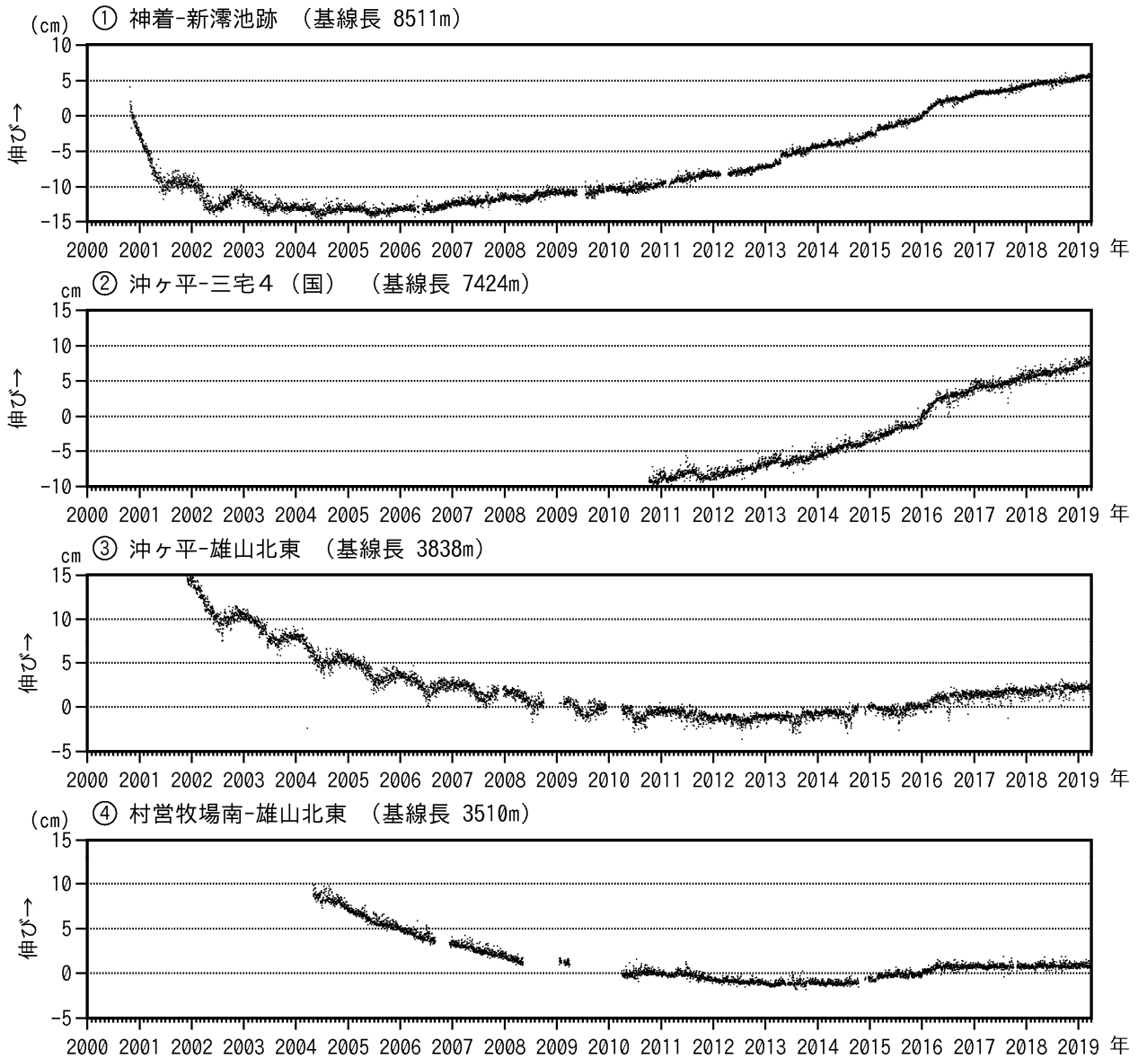
図9 三宅島 GNSS 連続観測結果（2000年10月26日～2019年3月31日）
