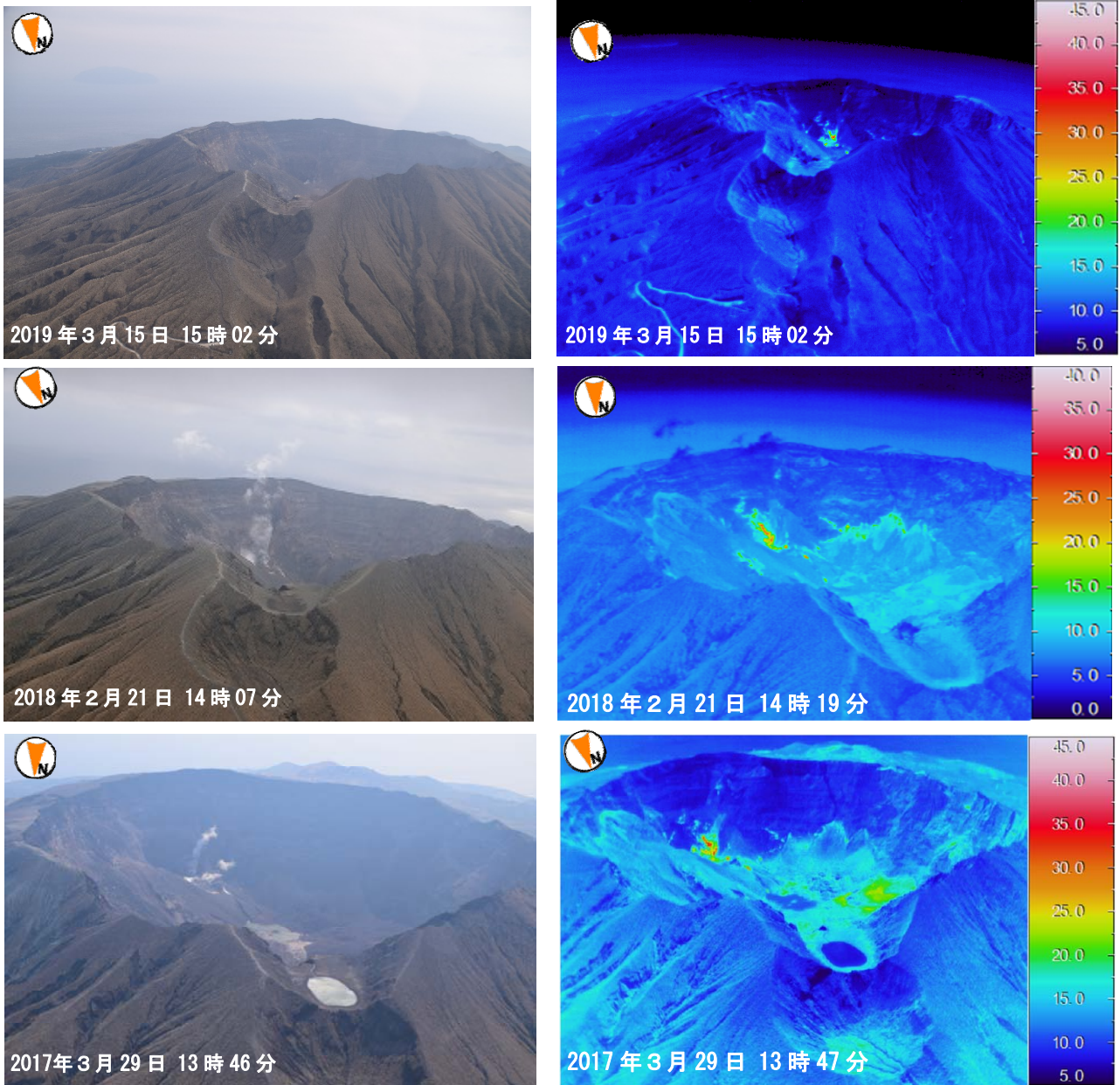
図4 三宅島 山頂火口の様子と赤外熱映像装置によるその地表面温度分布(陸上自衛隊の協力による) 上段: 天気: 薄曇り 気温: 8.7℃ (高度約1000mより撮影) 中段: 天気: 晴れ 気温: 2.4℃ (高度約1000mより撮影) 下段: 天気: 曇り 気温: 12.4℃ (高度約1200mより撮影) 火口の地形及び主火孔付近の地熱域の分布に特段の変化は認められません。
