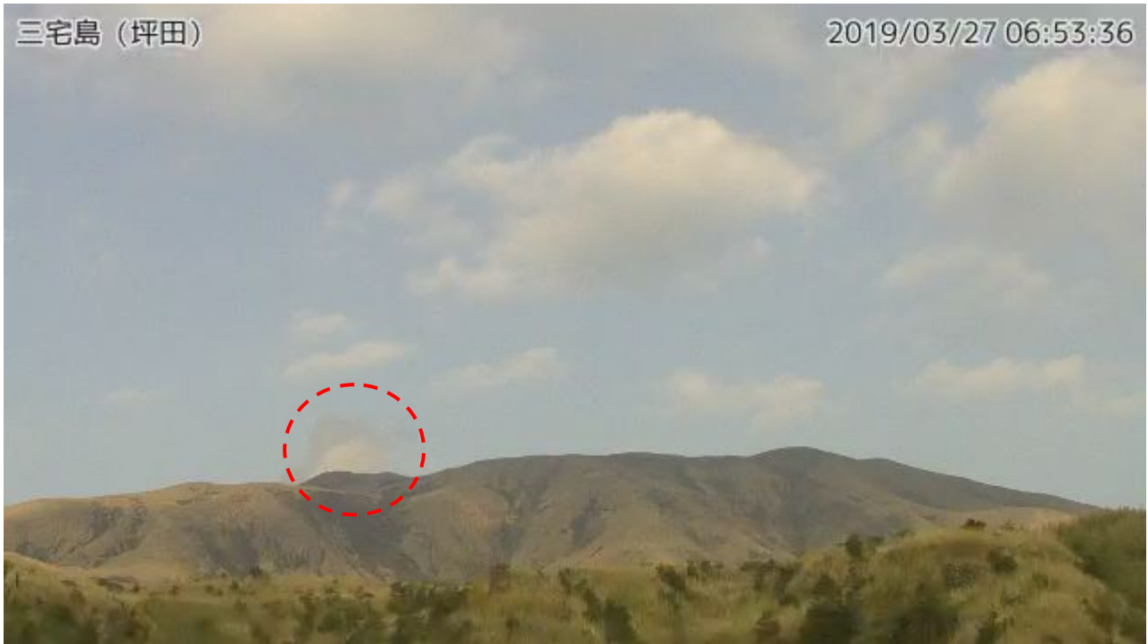
図1 三宅島 雄山山頂部の状況 坪田監視カメラ（3月27日）による。赤点線丸は噴気を示す。
