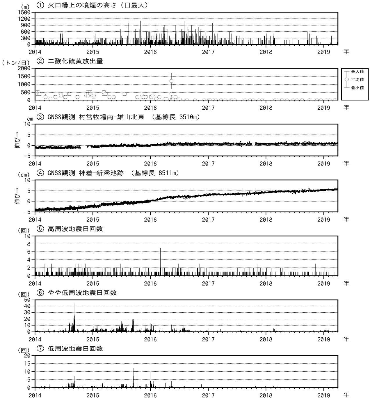
図 8 三宅島 火山活動短期経過図（2014 年 1 月 1 日～2019 年 3 月 31 日）
