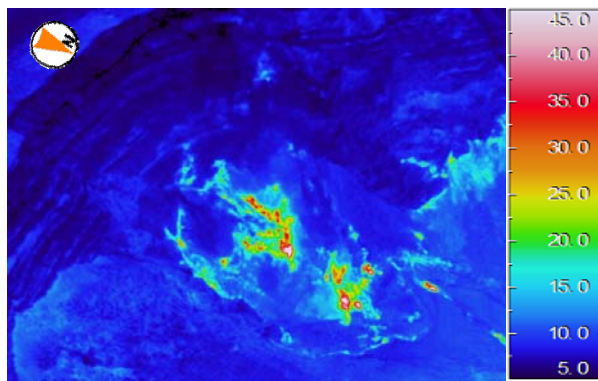
図6 三宅島 主火孔の状況 主火孔上空から撮影（陸上自衛隊の協力による）
