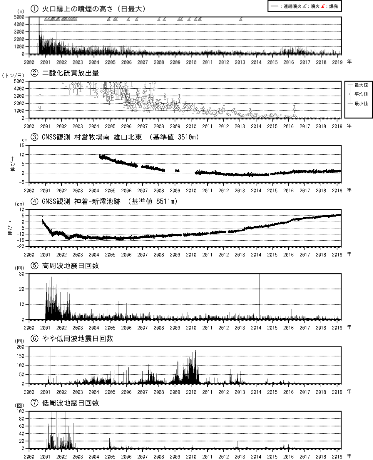
図7 三宅島 火山活動長期経過図（2000年1月1日～2019年3月31日）
