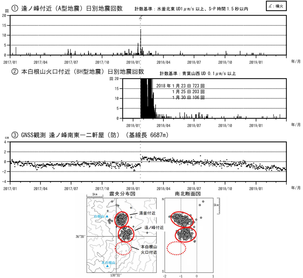
図 12 草津白根山（本白根山） 火山活動経過図（2017 年 1 月 1 日～2019 年 3 月 31 日）
