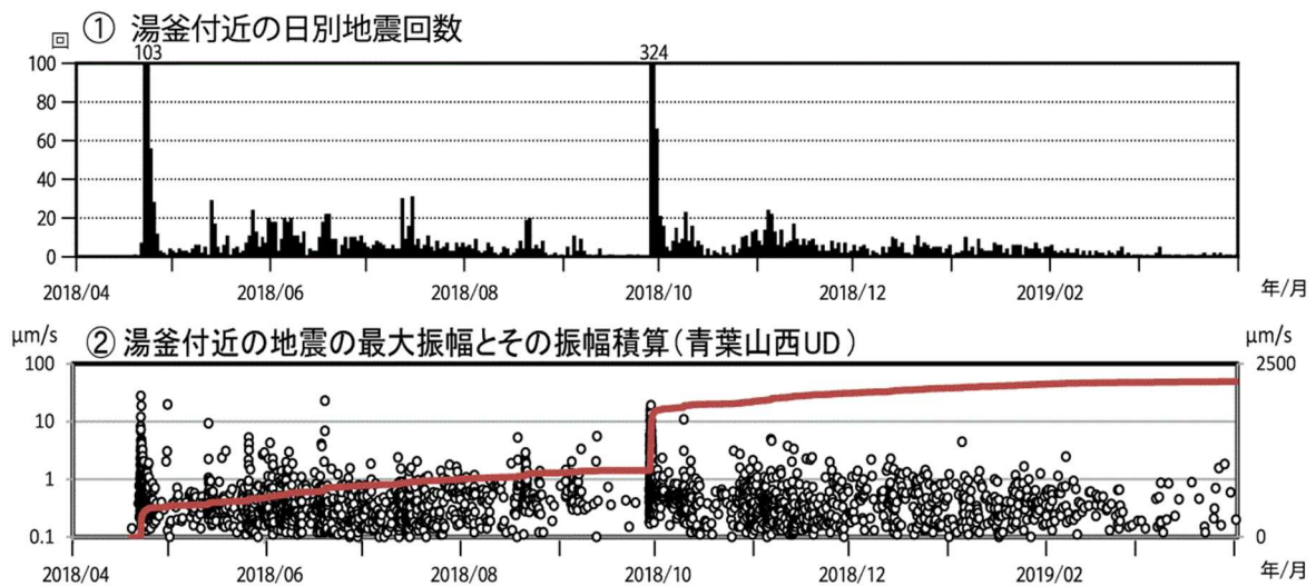
図2 草津白根山（白根山（湯釜付近）） 湯釜付近の地震活動（2018年4月1日～2019年3月31日） （○：最大振幅（左軸）、赤線：最大振幅の積算（右軸）） 湯釜付近を震源とする火山性地震は、2018年9月下旬に増加し、その後減少しましたが、増減を繰り返しており地震活動は継続しています。
