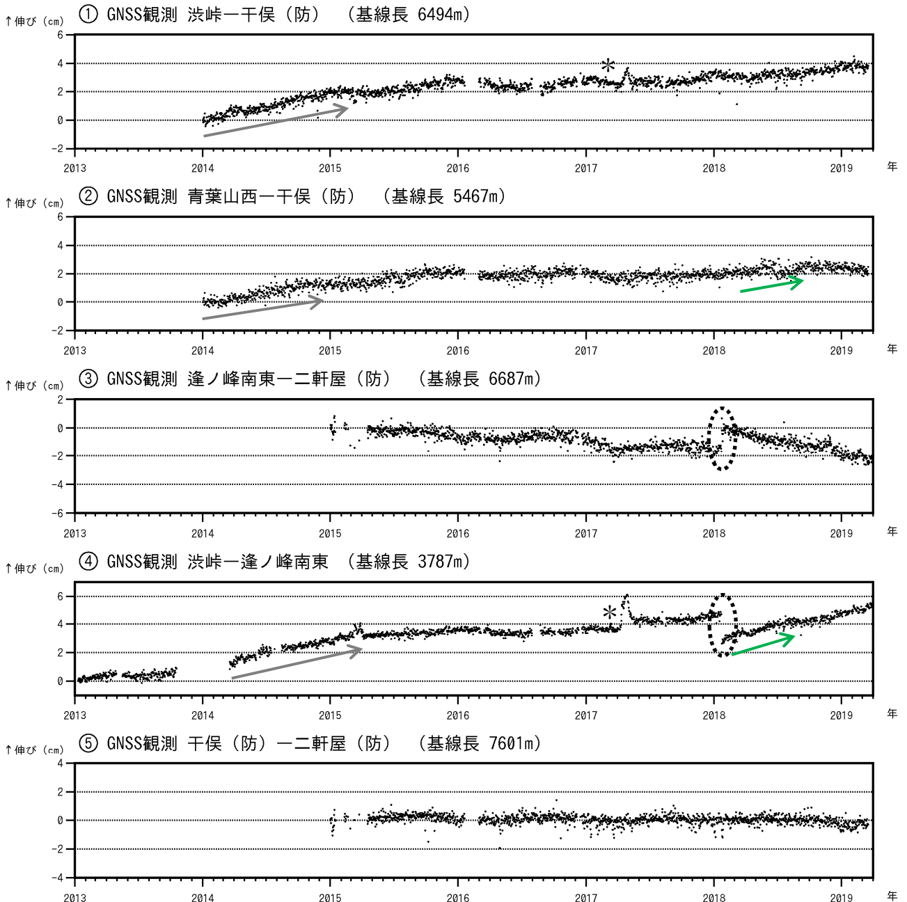
図7 草津白根山 GNSS連続観測の結果 (2013年1月1日～2019年3月31日)
