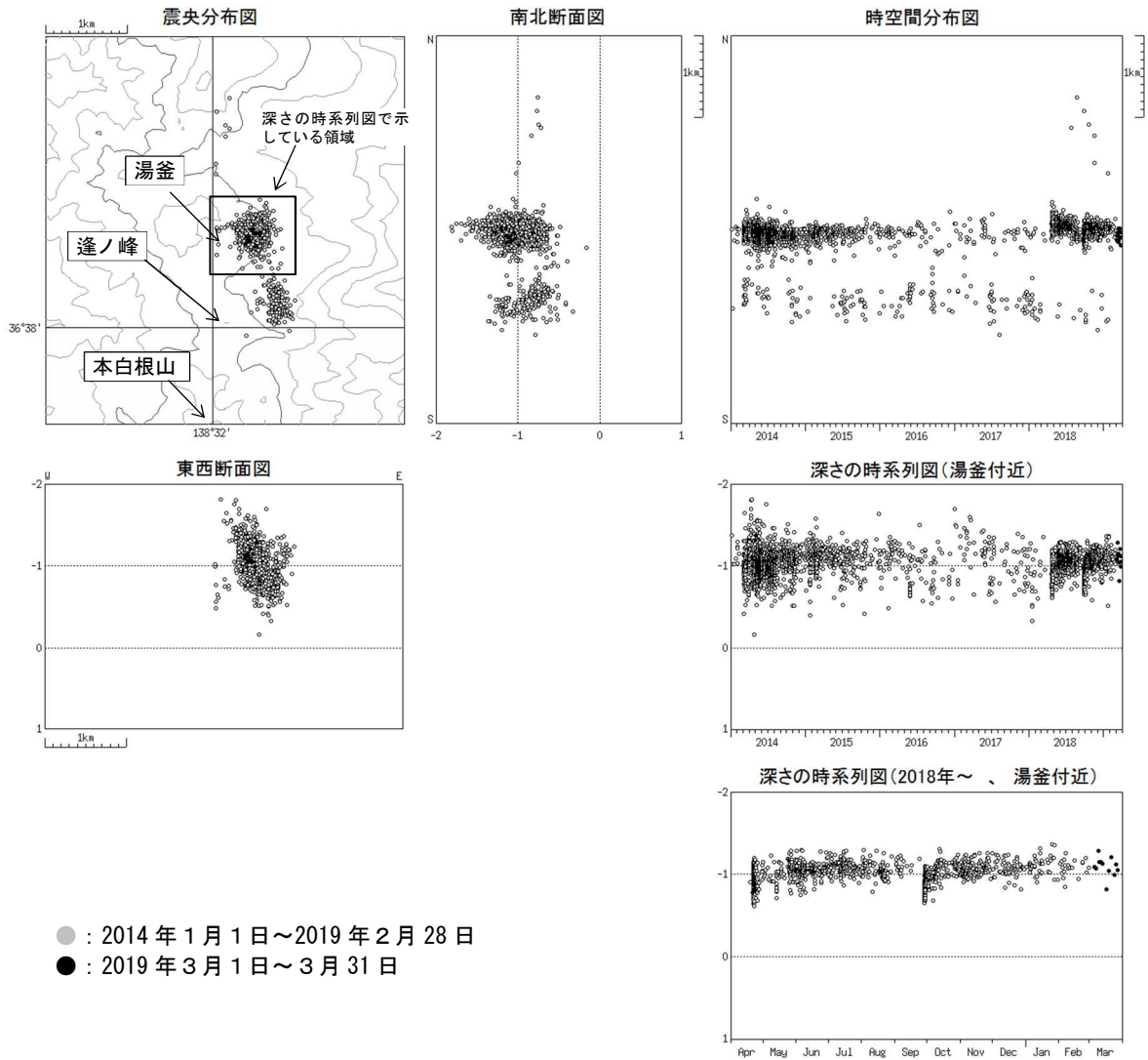
図5 草津白根山 震源分布図 (2014 年 1 月 1 日～2019 年 3 月 31 日) 火山性地震の震源は、湯釜付近の海拔約 1 km に分布しています。
