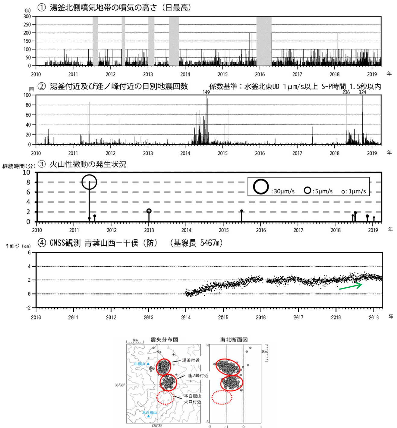
図4 草津白根山（白根山（湯釜付近）） 火山活動経過図（2010年1月1日～2019年3月31日）
