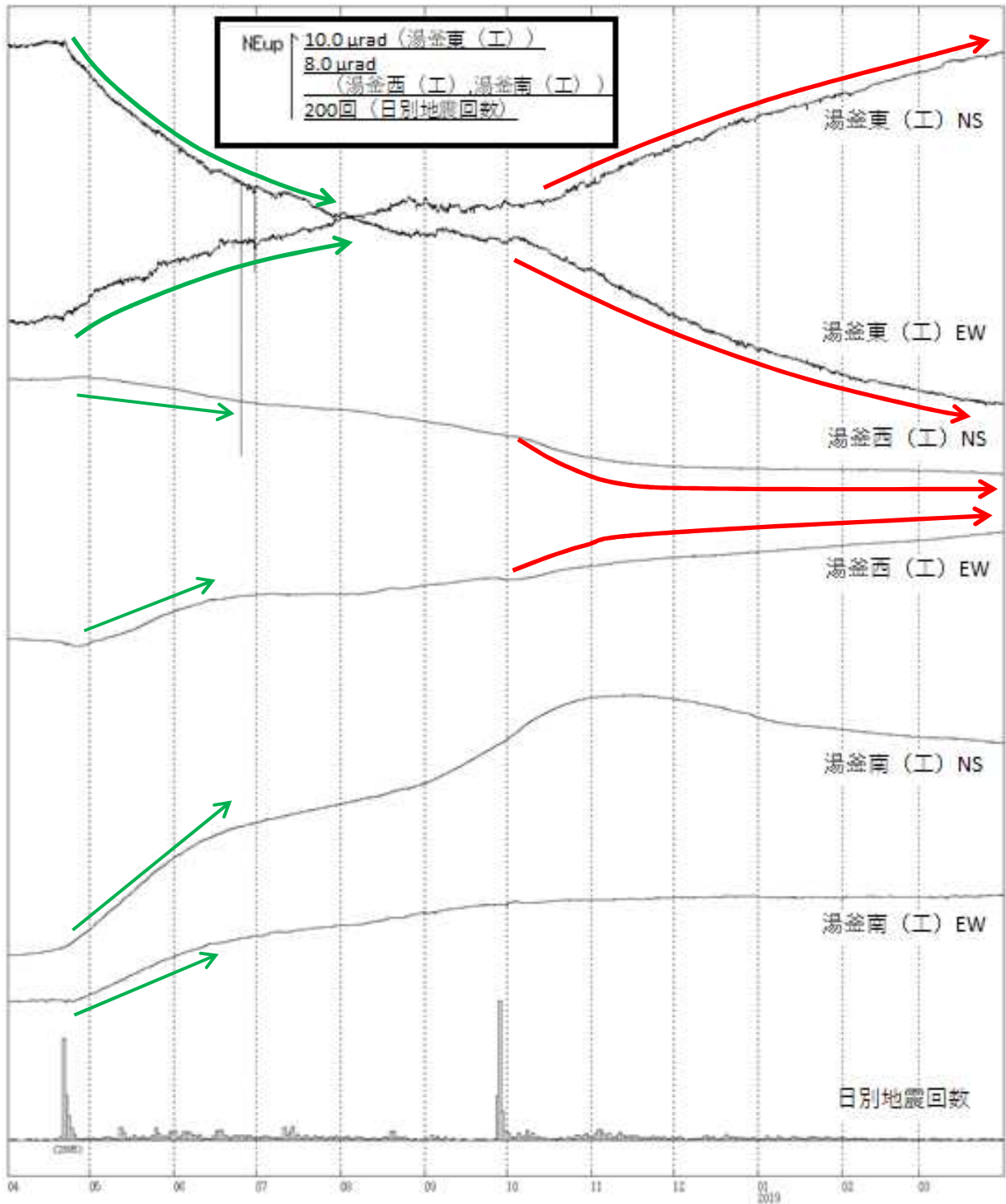
図3 草津白根山（白根山（湯釜付近）） 傾斜変動（2018年4月1日～2019年3月31日） （工）：東京工業大学
