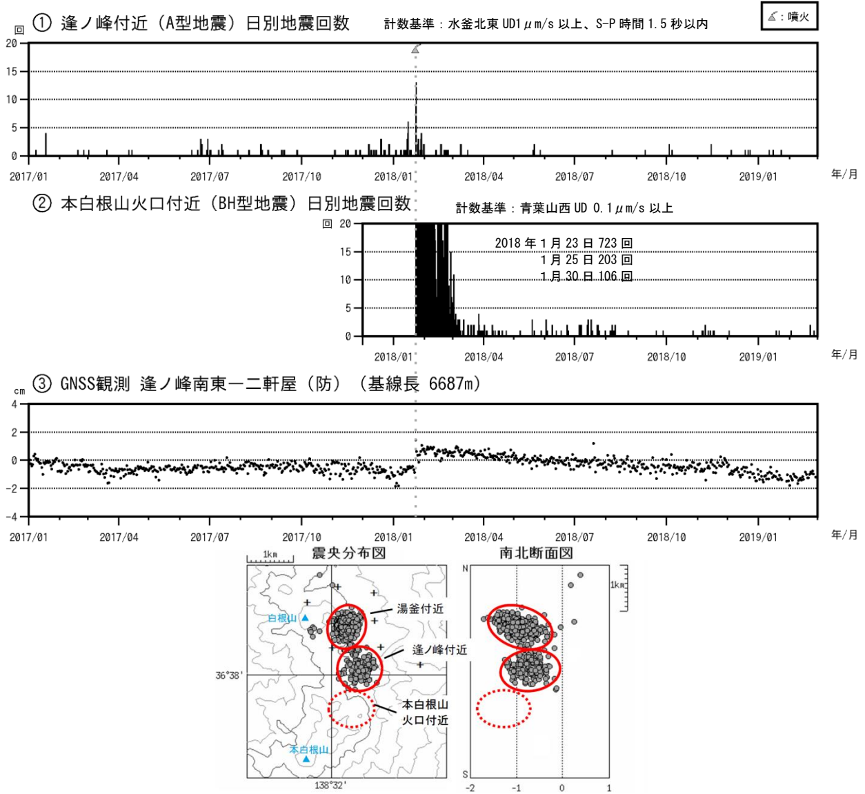
図 12 草津白根山（本白根山） 火山活動経過図（2017 年 1 月 1 日～2019 年 2 月 28 日）
