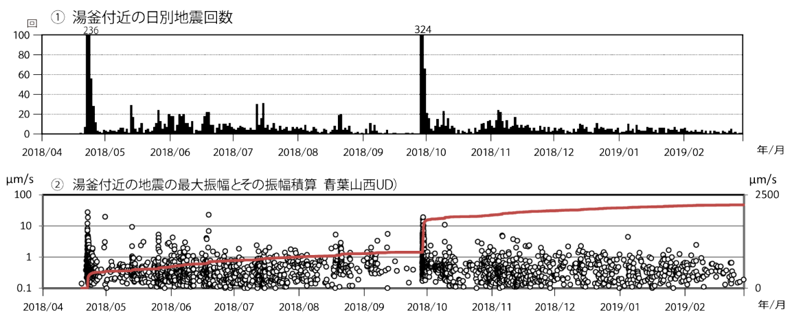
図 2 草津白根山（白根山（湯釜付近）） 湯釜付近の地震活動（2018年4月1日～2019年2月28日） （○：最大振幅（左軸）、赤線：最大振幅の積算（右軸）） 湯釜付近を震源とする火山性地震は、2018年9月下旬に増加し、その後減少しましたが、増減を繰り返しており地震活動は継続しています。
