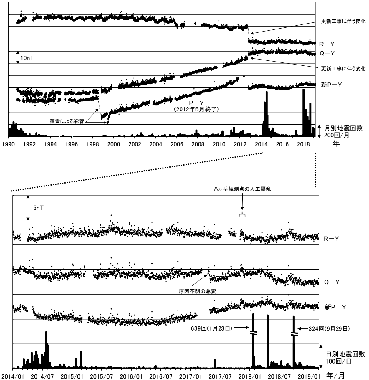
図 8 草津白根山（白根山（湯釜付近））全磁力連続観測による全磁力値の変化及び地震回数
