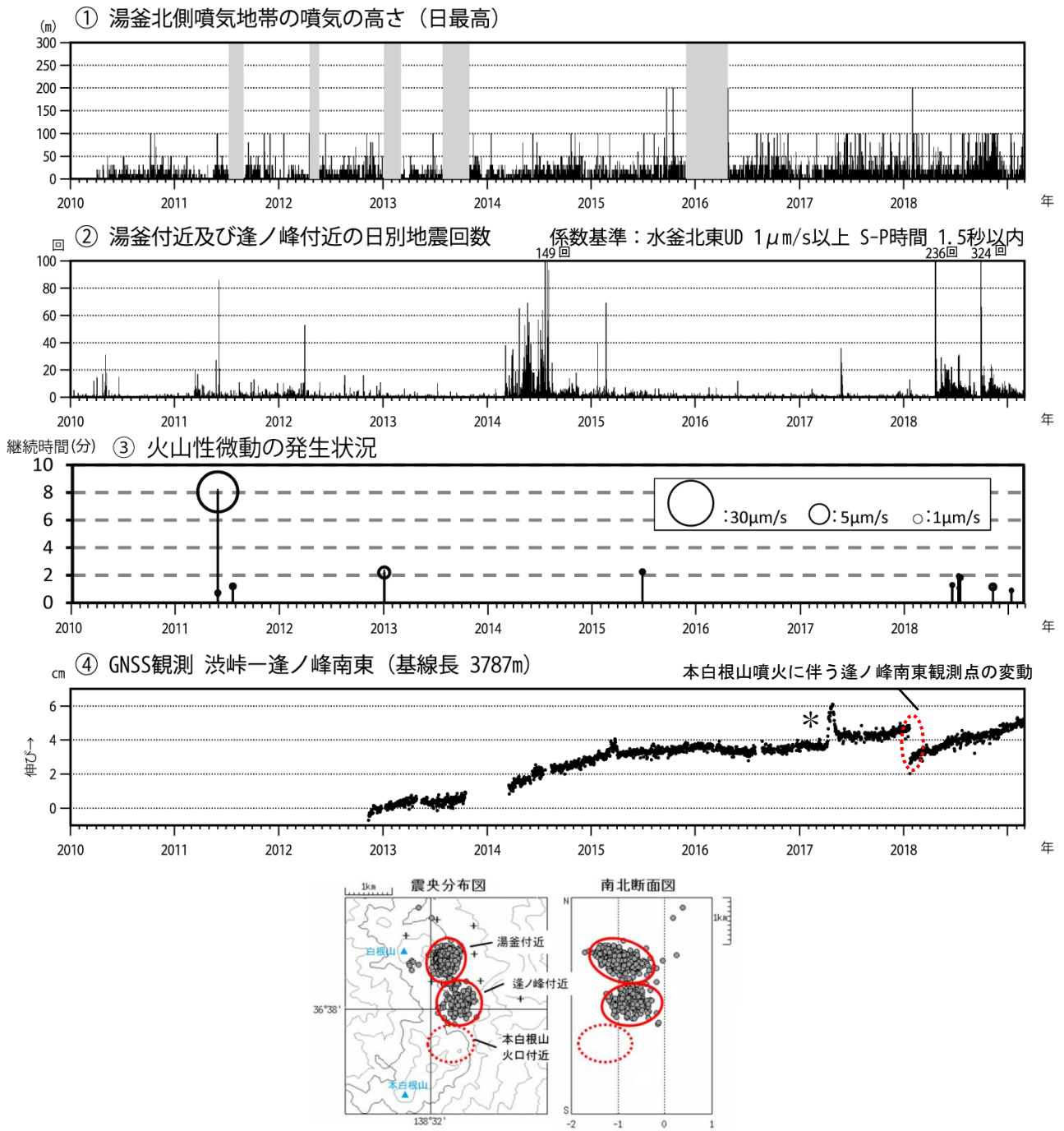
図 4 草津白根山（白根山（湯釜付近））火山活動経過図（2010 年 1 月 1 日～2019 年 2 月 28 日）
