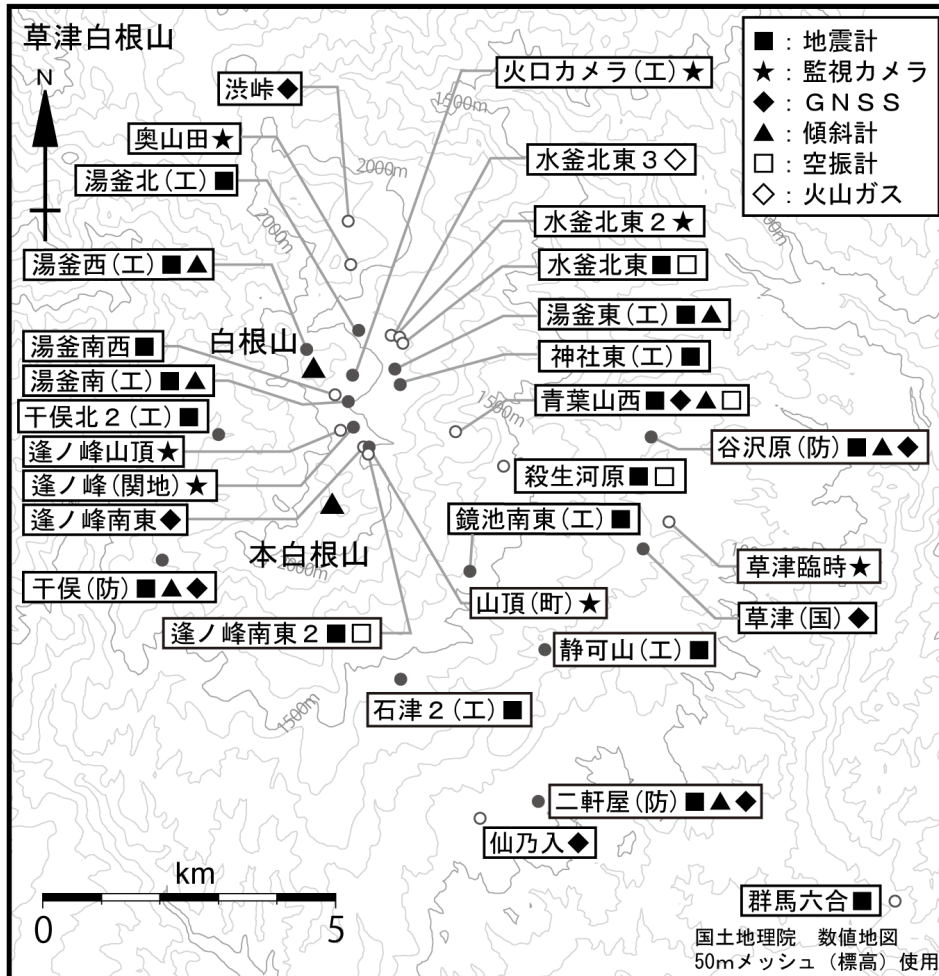
図 14 草津白根山 観測点配置図
