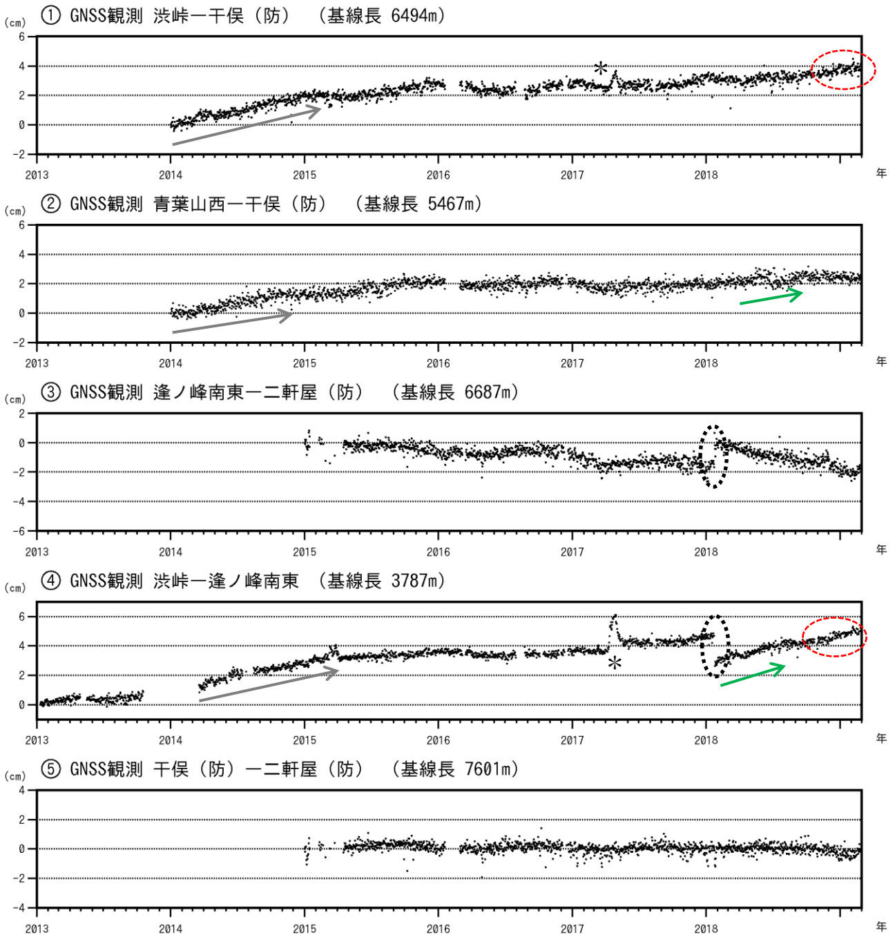
図7 草津白根山 GNSS連続観測の結果（2013年1月1日～2019年2月28日）
