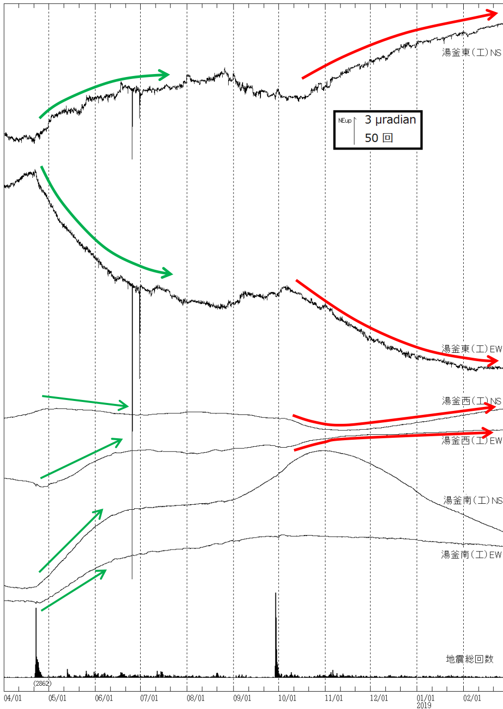
図3 草津白根山（白根山（湯釜付近）） 傾斜変動（2018年4月1日～2019年2月28日） (工)：東京工業大学
