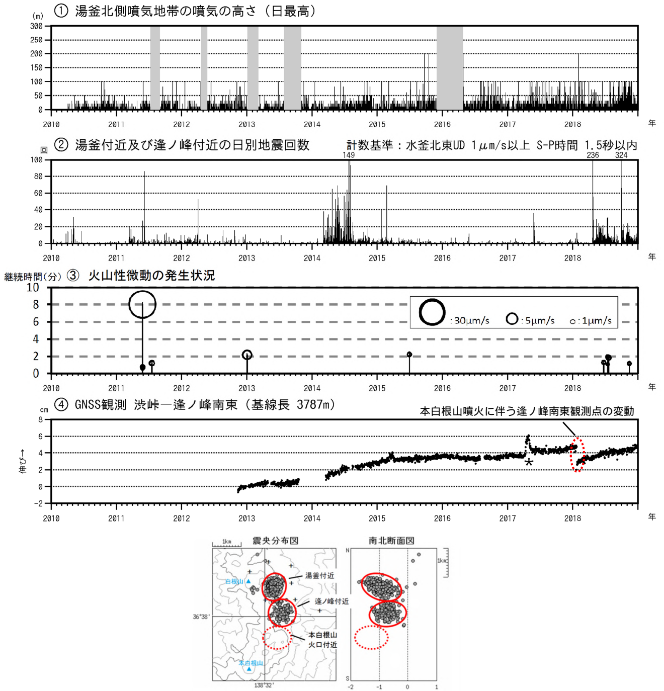
図4 草津白根山（白根山（湯釜付近））火山活動経過図（2010年1月1日～2018年12月31日）の灰色部分およびの空白部分は欠測を示します。 は図15のの基線に対応しています。 *の変動は、火山活動に起因するものではないと考えられます。 2013年1月に解析方法を変更しています。 最下段の震源分布図は、の地震の震源の概ねの位置を示しています。
