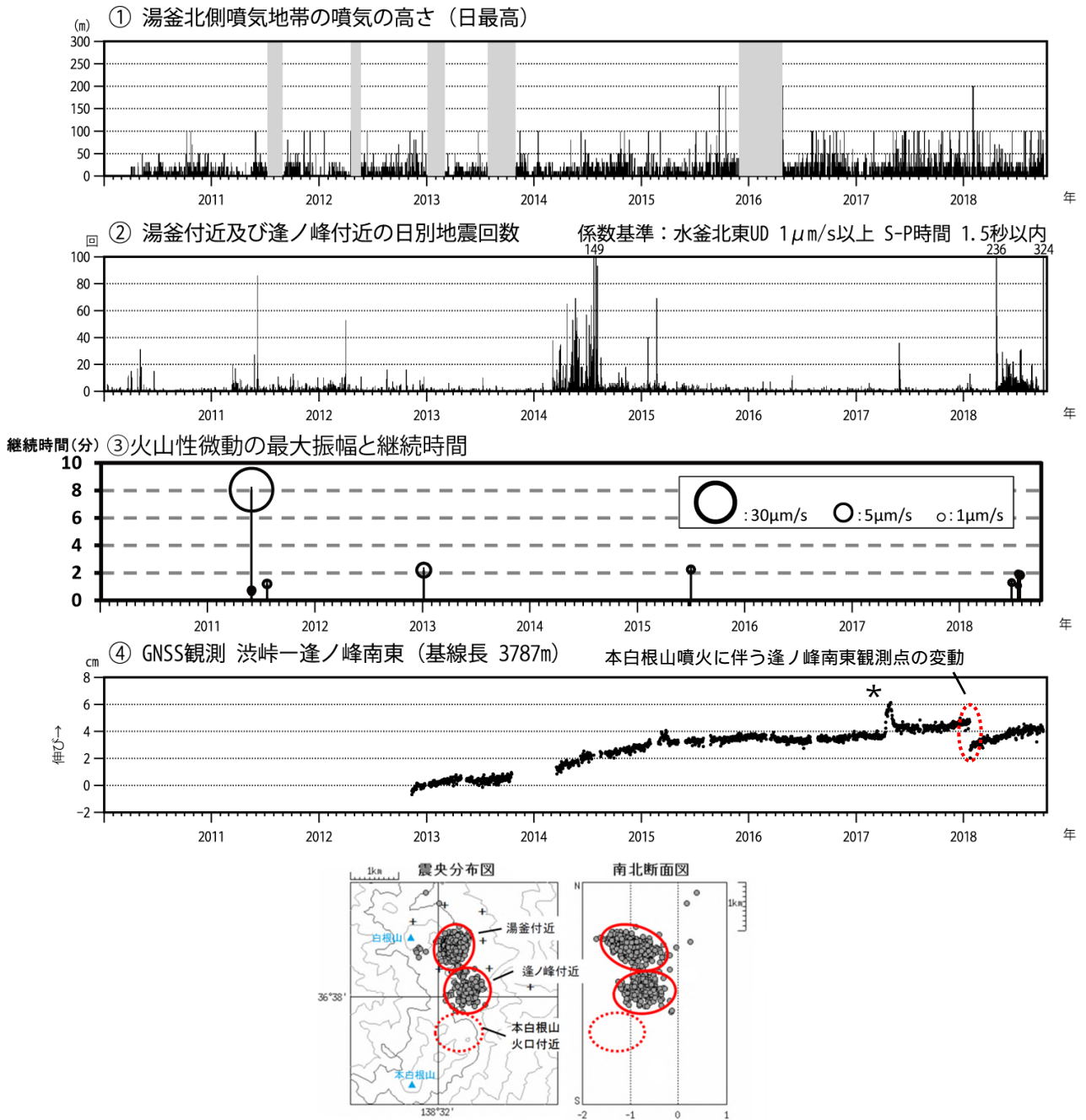
図4 草津白根山（白根山（湯釜付近））火山活動経過図（2010年1月1日～2018年9月30日）の灰色部分およびの空白部分は欠測を示します。は図17のの基線に対応しています。*の変動は、渋峠観測点の凍上による変動と考えられます。2013年1月に解析方法を変更しています。最下段の震源分布図は、の地震の震源の概ねの位置を示しています。
