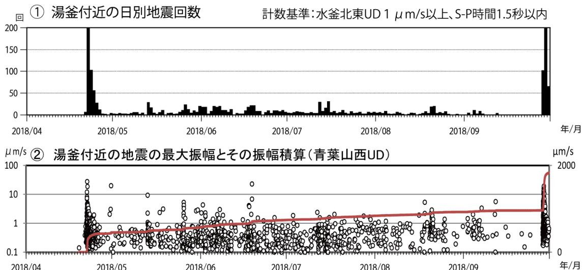
図2 草津白根山(白根山(湯釜付近)) 湯釜付近の地震活動(2018年4月1日~9月30日)
