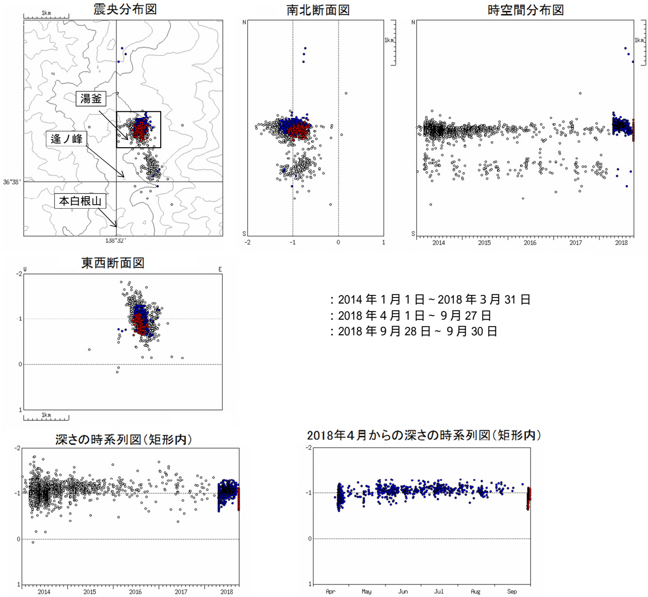
図5 草津白根山 震源分布図(2014年1月1日～2018年9月30日)
