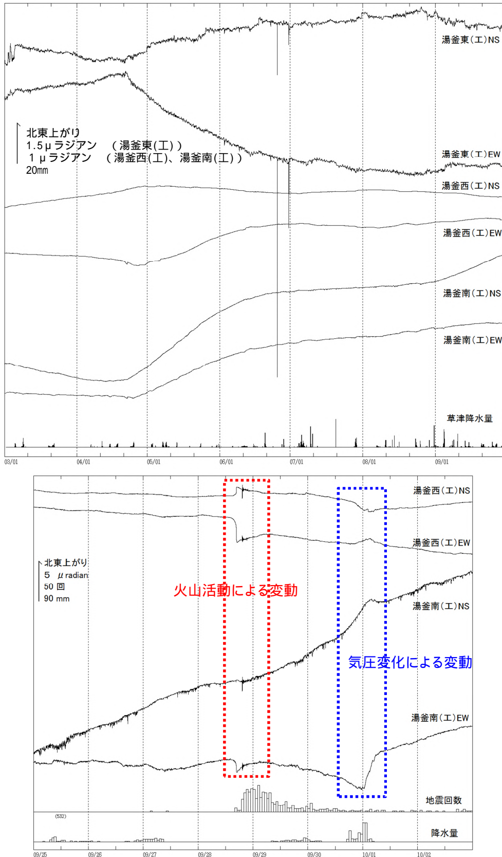
図3 草津白根山(白根山(湯釜付近)) 傾斜変動
