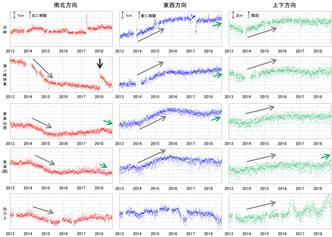
図9 草津白根山 GNSS観測による各観測点の変動(2013年1月1日~2018年9月29日) 地震等によるステップ、季節変動を除去しています。
