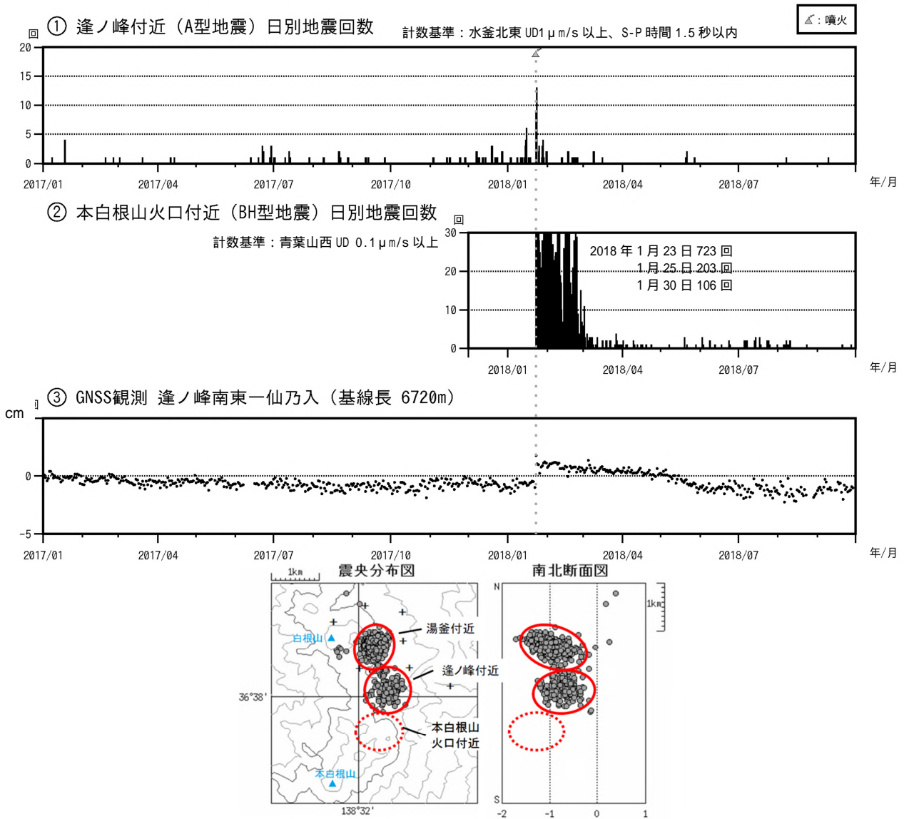
図15 草津白根山(本白根山) 火山活動経過図(2017年1月1日~2018年9月30日) 草津白根山では、火山性地震はその発生領域から、「湯釜付近」、「逢ノ峰付近」、「本白根山火口付近」に分けています。 本白根山の火山活動については、逢ノ峰付近と本白根山火口付近の地震活動に注目して監視しています。 火山性地震の種類については図16を参照してください。
