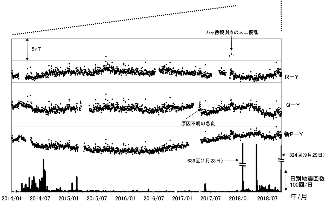
図 11 草津白根山（白根山（湯釜付近））全磁力連続観測による全磁力値の変化及び地震回数
