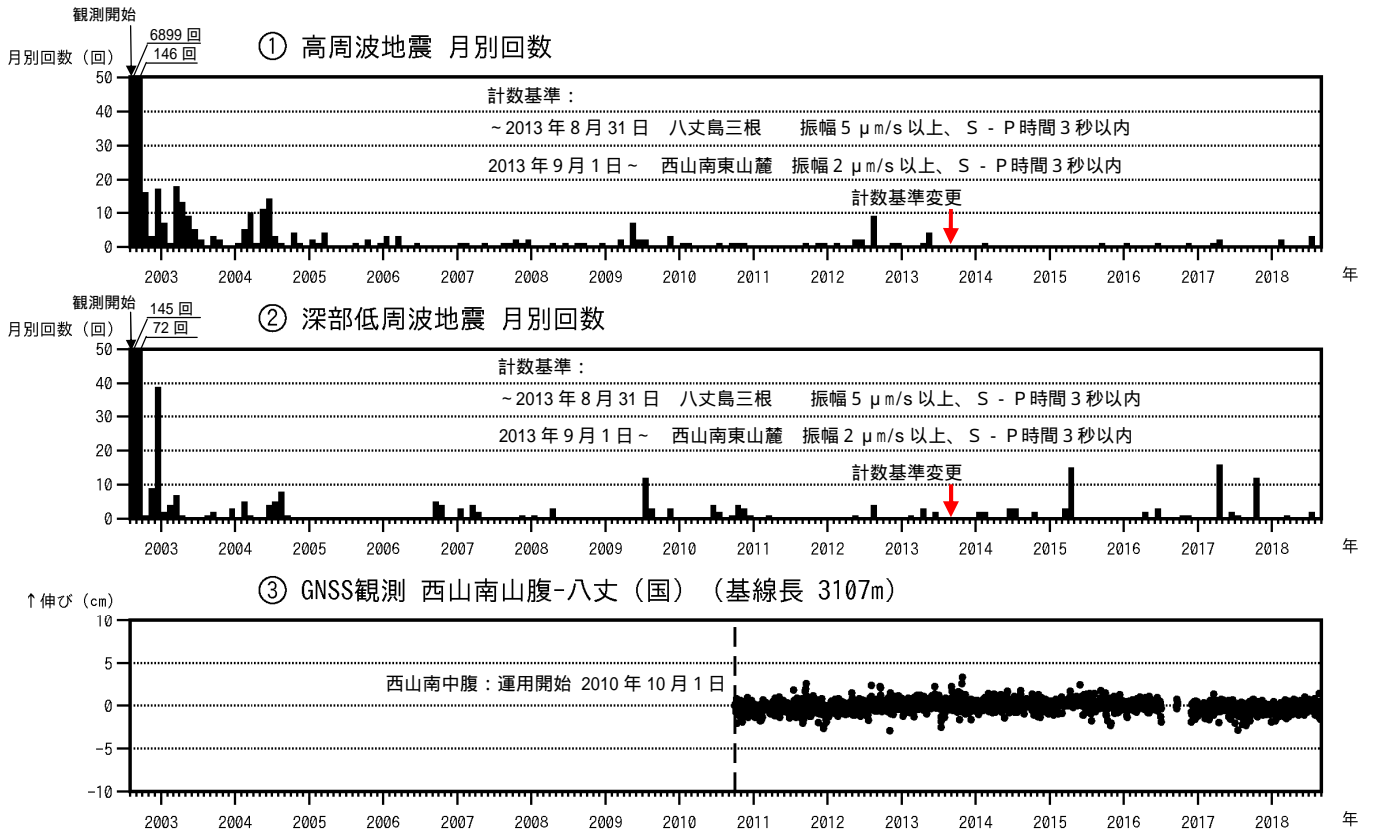
図2 八丈島 火山活動経過図(2002年8月13日~2018年8月31日)
