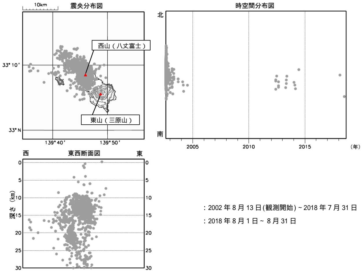
図3 八丈島 震源分布図(2002年8月13日～2018年8月31日) ・今期間、震源の求まる地震の発生はありません。
