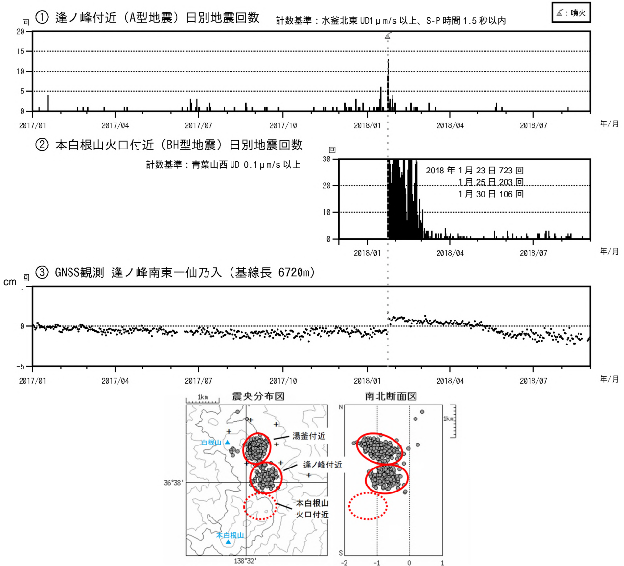
図12 草津白根山(本白根山) 火山活動経過図(2017年1月1日~2018年8月31日)
