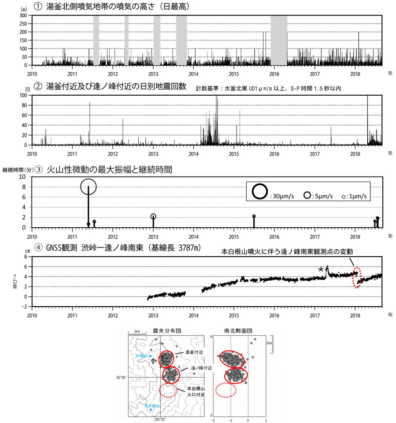
図3 草津白根山（白根山（湯釜付近））火山活動経過図（2010年1月1日～2018年8月31日）の灰色部分およびの空白部分は欠測を示します。は図14のの基線に対応しています。*の変動は、渋峠観測点の凍上による変動と考えられます。2013年1月に解析方法を変更しています。最下段の震源分布図は、の地震の震源の概ねの位置を示しています。
