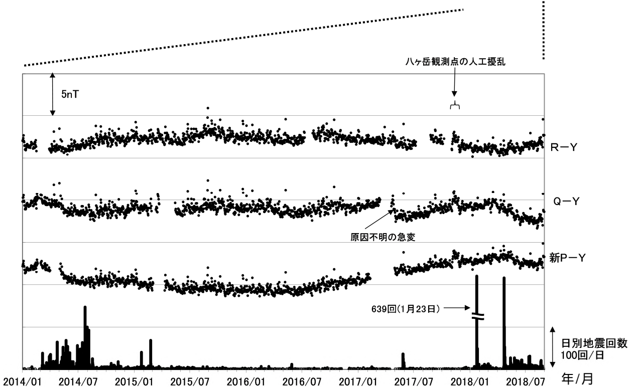
図8 草津白根山(白根山(湯釜付近))全磁力連続観測による全磁力値の変化及び地震回数
