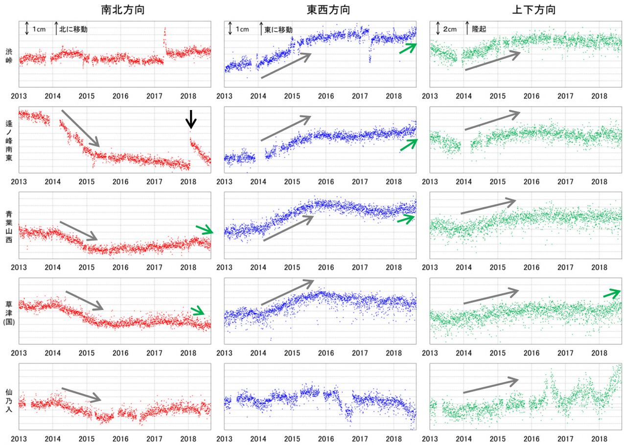
図6 草津白根山 GNSS観測による各観測点の変動(2013年1月1日~2018年8月31日) 地震等によるステップ、季節変動を除去しています。
