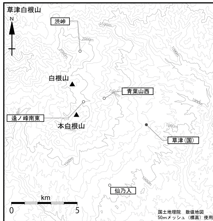
図7 草津白根山 GNSS観測点配置図 (国)国土地理院
