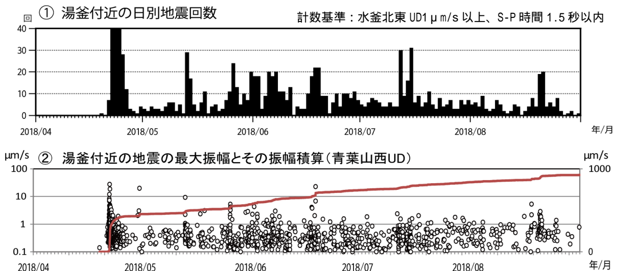
図2 草津白根山（白根山（湯釜付近）） 湯釜付近の地震活動（2018年4月1日～8月31日） (○：最大振幅(左軸)、赤線：最大振幅の積算(右軸)) 湯釜付近を震源とする火山性地震は、5月下旬以降増減を繰り返しています。
