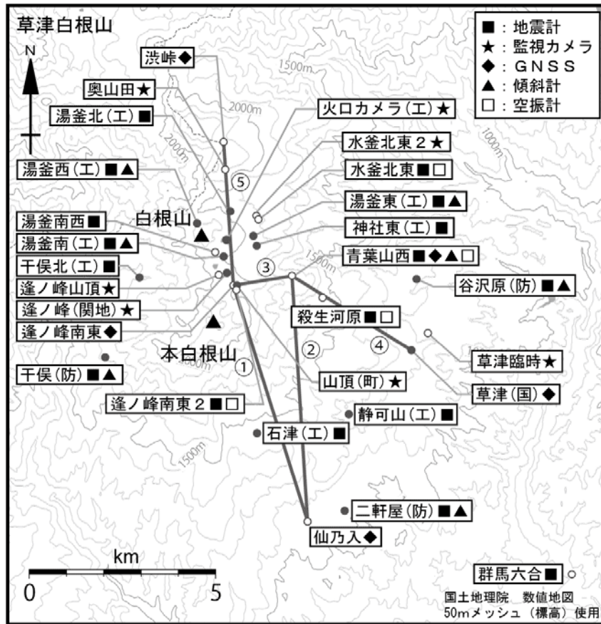
図 15 草津白根山 観測点配置図
