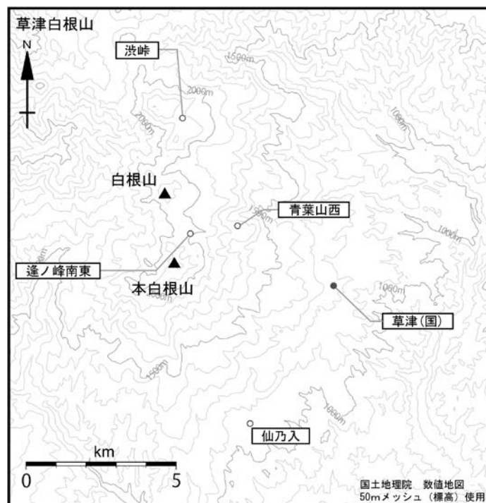
図7 草津白根山 GNSS 観測点配置図
