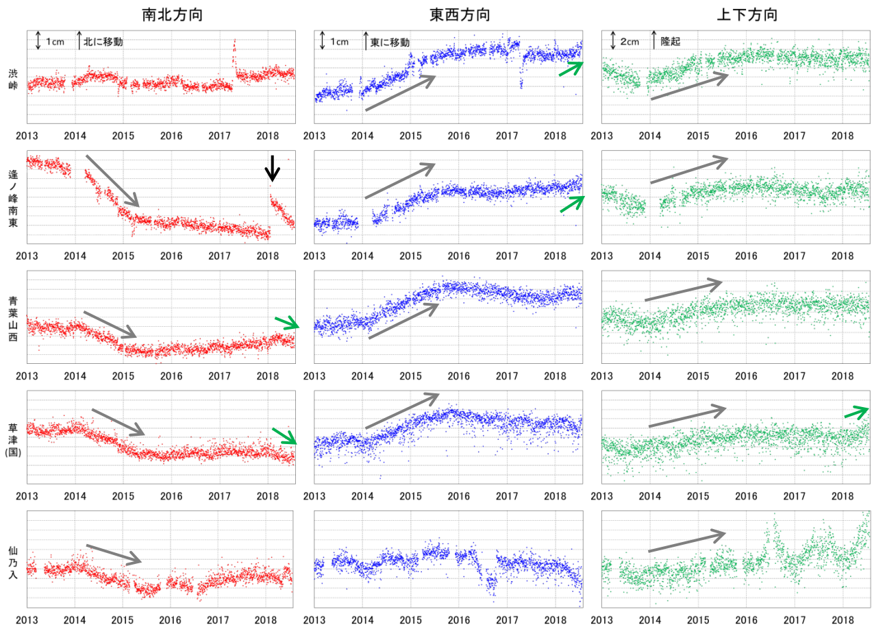
図6 草津白根山 GNSS 観測による各観測点の変動（2013 年 1 月 1 日～2018 年 7 月 31 日）
