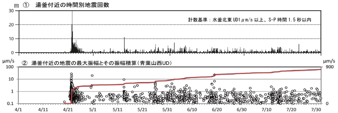
図3 草津白根山（白根山（湯釜付近）） 湯釜付近の地震活動（2018年4月1日～7月31日）
