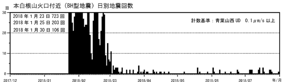
図 13 草津白根山 (本白根山) 本白根山火口付近の BH 型地震日回数
