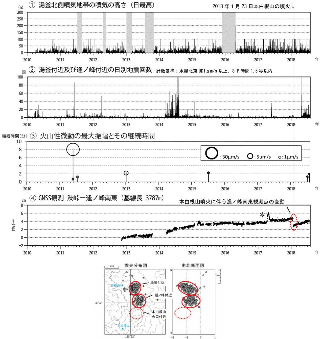
図2 草津白根山（白根山（湯釜付近））火山活動経過図（2010年1月1日～2018年7月31日）
