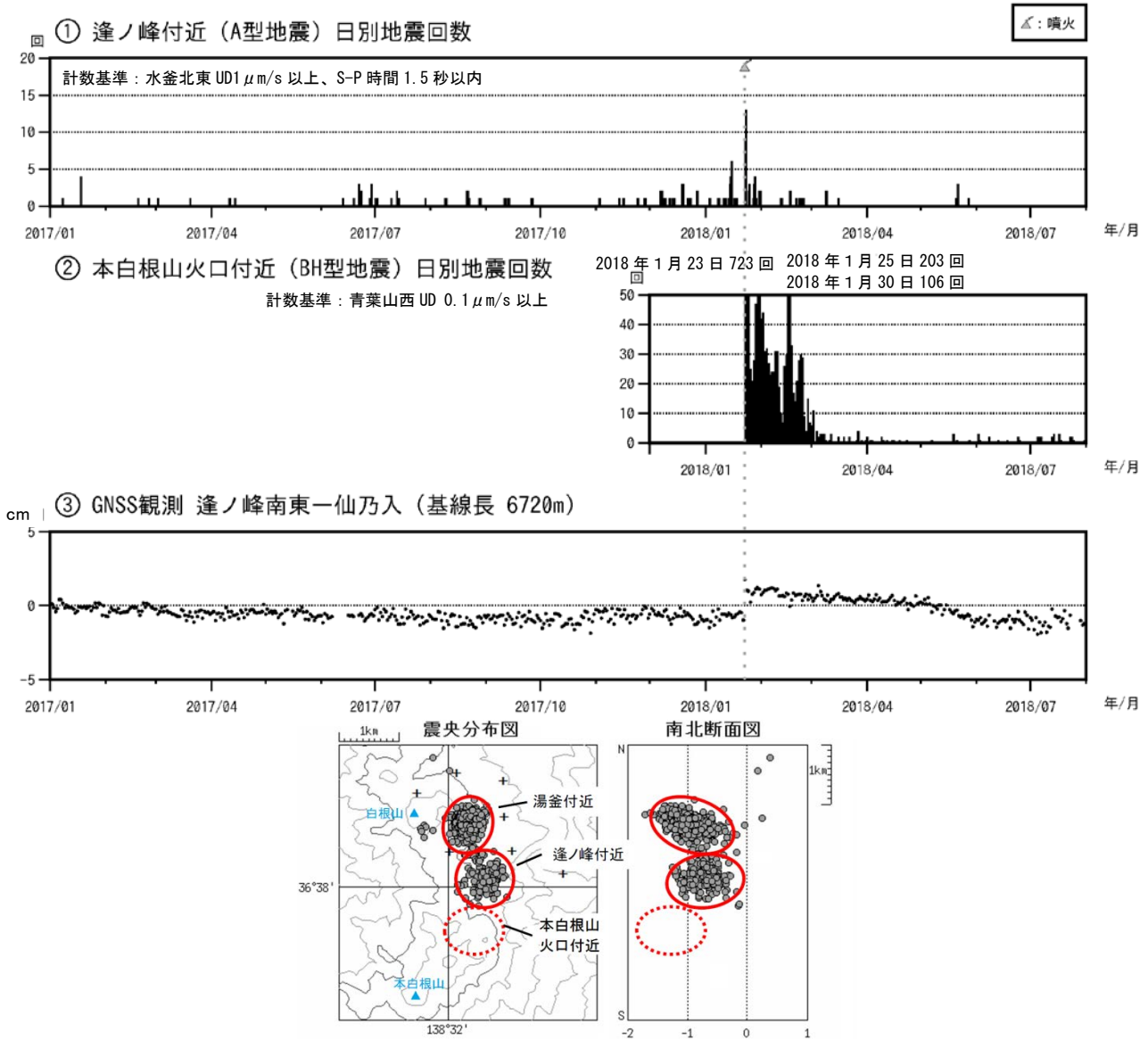
図 12 草津白根山 (本白根山) 火山活動経過図 (2017 年 1 月 1 日～2018 年 7 月 31 日)
