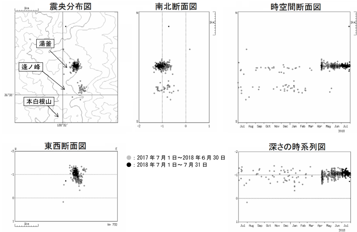
図4 草津白根山 震源分布図（2017年7月1日～2018年7月31日）
