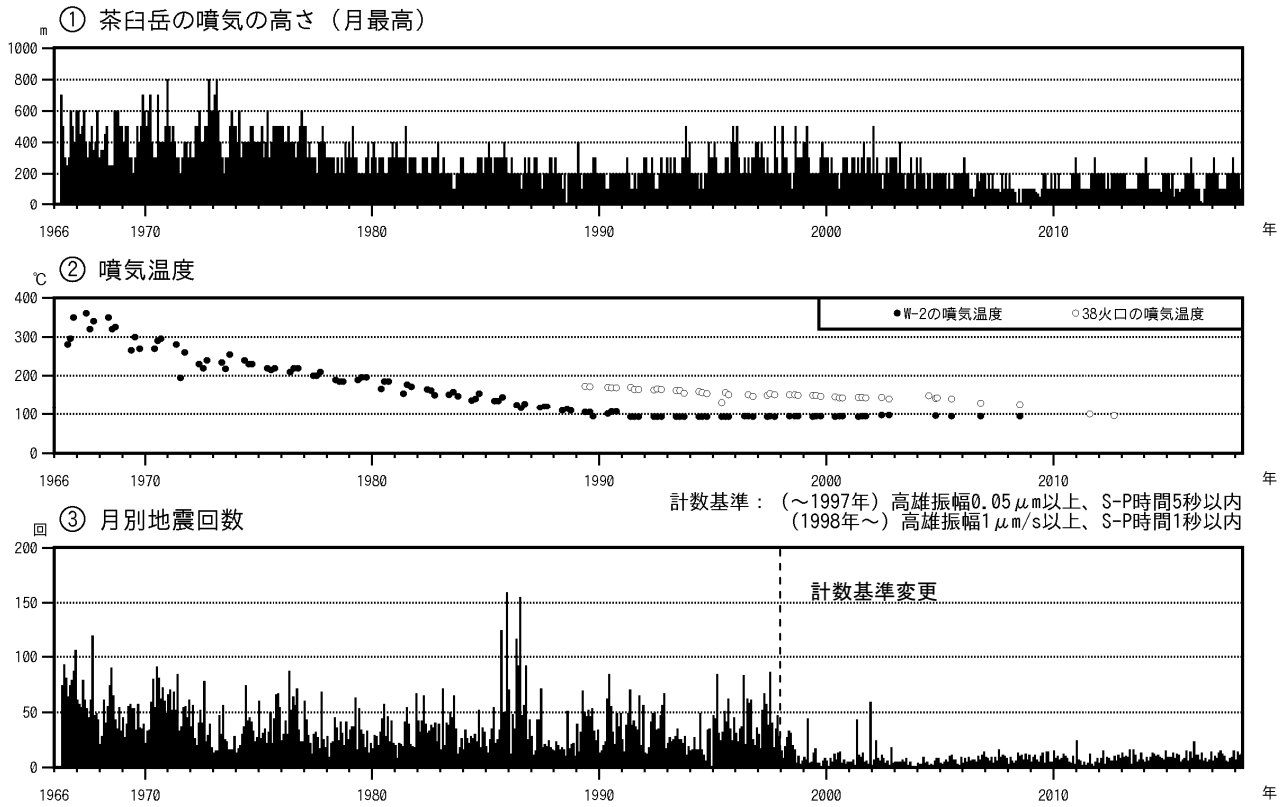
図2 那須岳 火山活動経過図（1966年1月～2018年7月）
