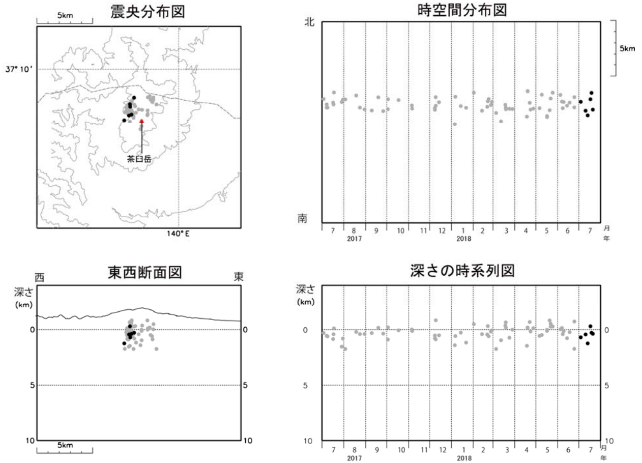
図 4 那須岳 震源分布図 (2017 年 7 月 1 日～2018 年 7 月 31 日)
