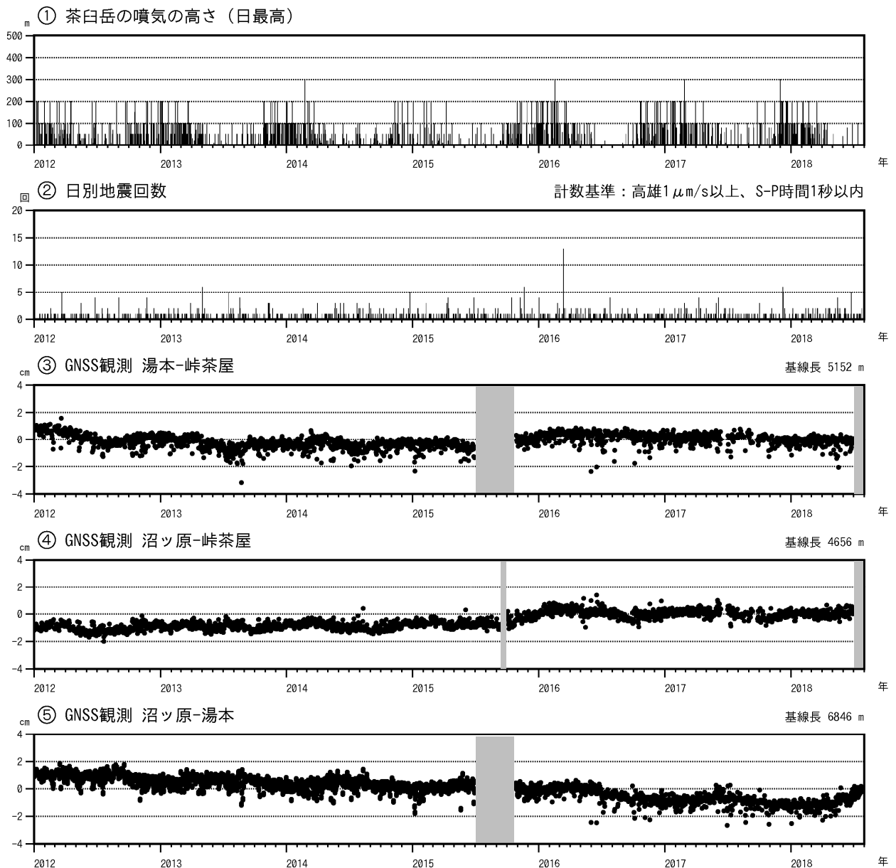
図3 那須岳 火山活動経過図（2012年1月1日～2018年7月31日）
