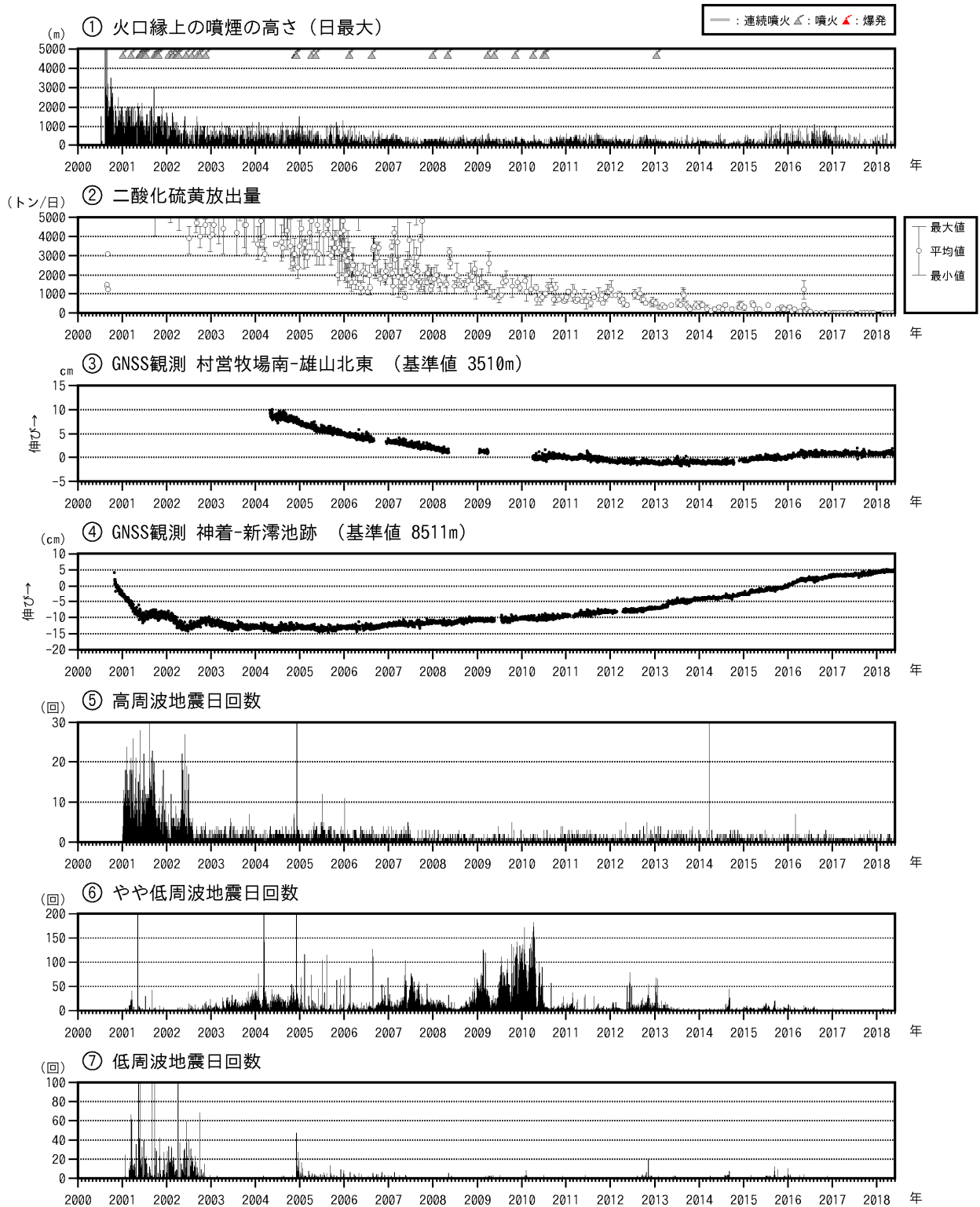
図5 三宅島 火山活動長期経過図（2000年1月1日～2018年5月31日）
