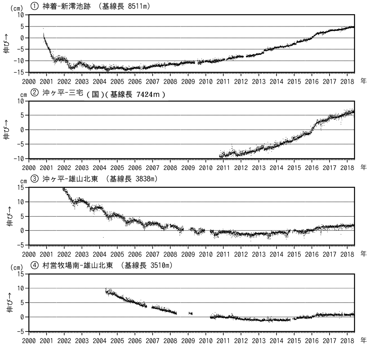
図7 三宅島 GNSS 連続観測結果(2000年10月26日~2018年5月31日)
