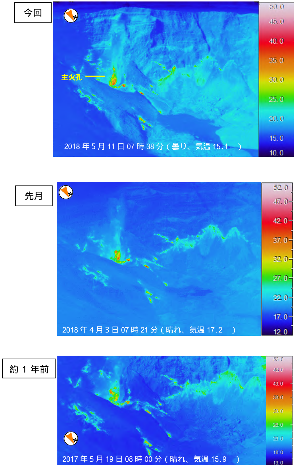
図 4 三宅島 赤外熱映像装置による山頂火口内の地表面温度分布
