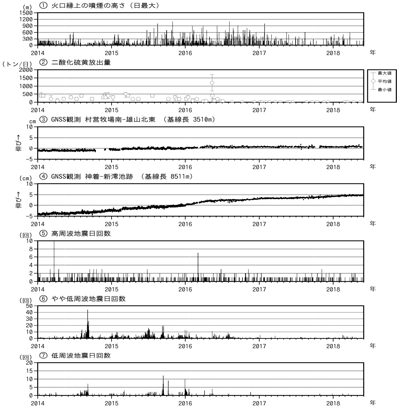
図6 三宅島 火山活動短期経過図(2014年1月1日~2018年5月31日)
