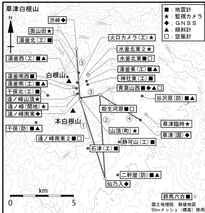
図17 草津白根山 観測点配置図
