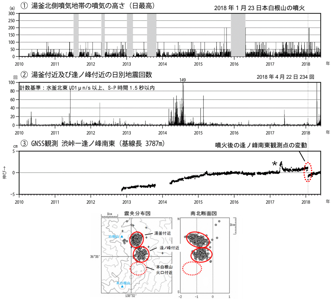
図2 草津白根山（白根山（湯釜付近）） 火山活動経過図（2010年1月1日～2018年5月31日）の灰色部分およびの空白部分は欠測を示します。
