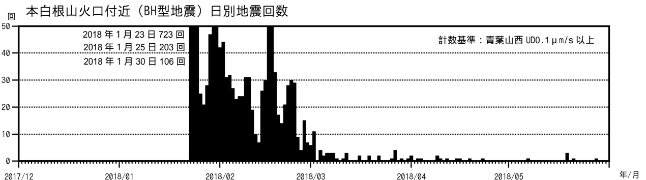
図 15 草津白根山(本白根山) 本白根山火口付近の BH 型地震日回数(2017年12月1日~5月31日) ・ 噴火発生後、本白根山火口付近で BH 型の火山性地震が多発し、その後も少ないながらも継続しています。
