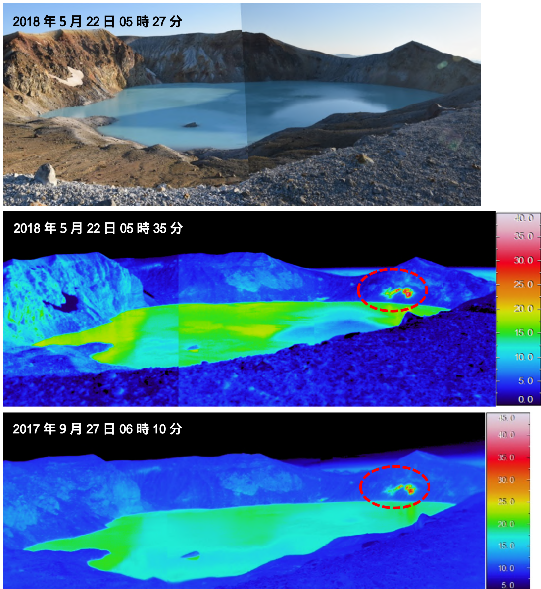
図6 草津白根山（白根山（湯釜付近））湯釜火口内壁の赤外熱映像 ・湯釜火口内にみられている地熱域（図中赤破線）について、前回（2017年9月27日）の調査結果と比較して、地熱域の広がりや温度に顕著な変化は認められませんでした。
