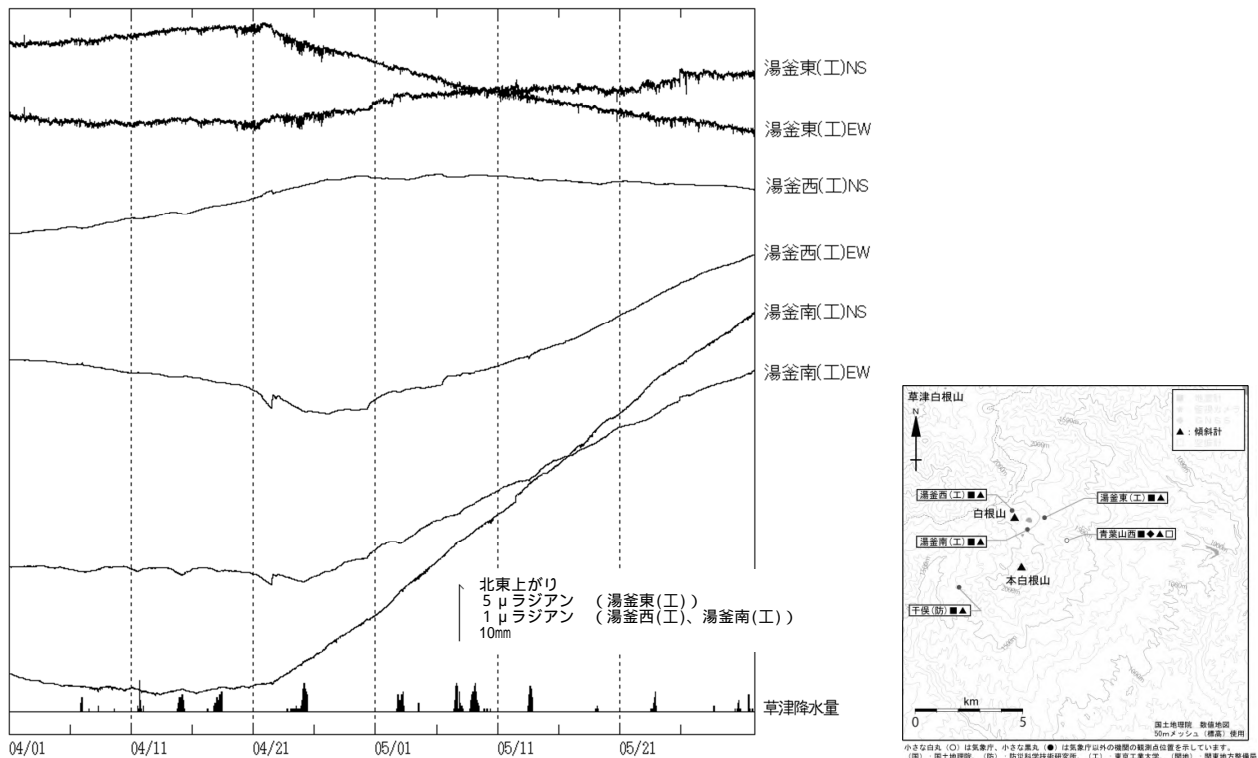
図5 草津白根山（白根山（湯釜付近）） 傾斜変動（2018年4月1日～5月31日）
