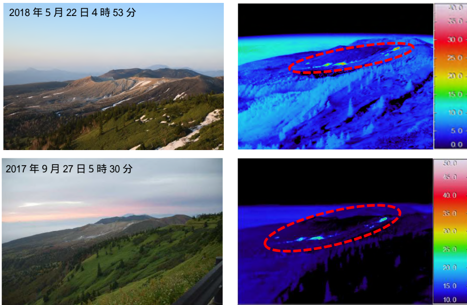
図 8 草津白根山（白根山（湯釜付近））湯釜の北側の赤外熱映像
