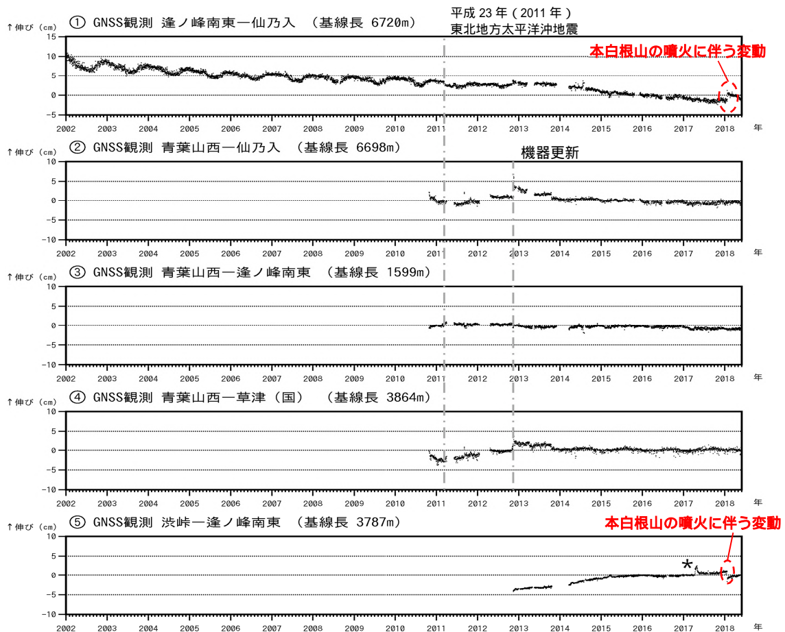
図 9 草津白根山 GNSS 連続観測による基線長変化（2002 年 1 月 1 日～2018 年 5 月 31 日）
