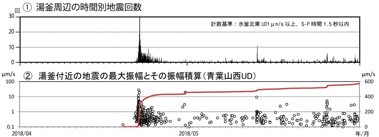
図3 草津白根山（白根山（湯釜付近）） 湯釜付近の地震活動（2018年4月1日～5月31日）（○：最大振幅（左軸）、赤線：最大振幅の積算（右軸））
