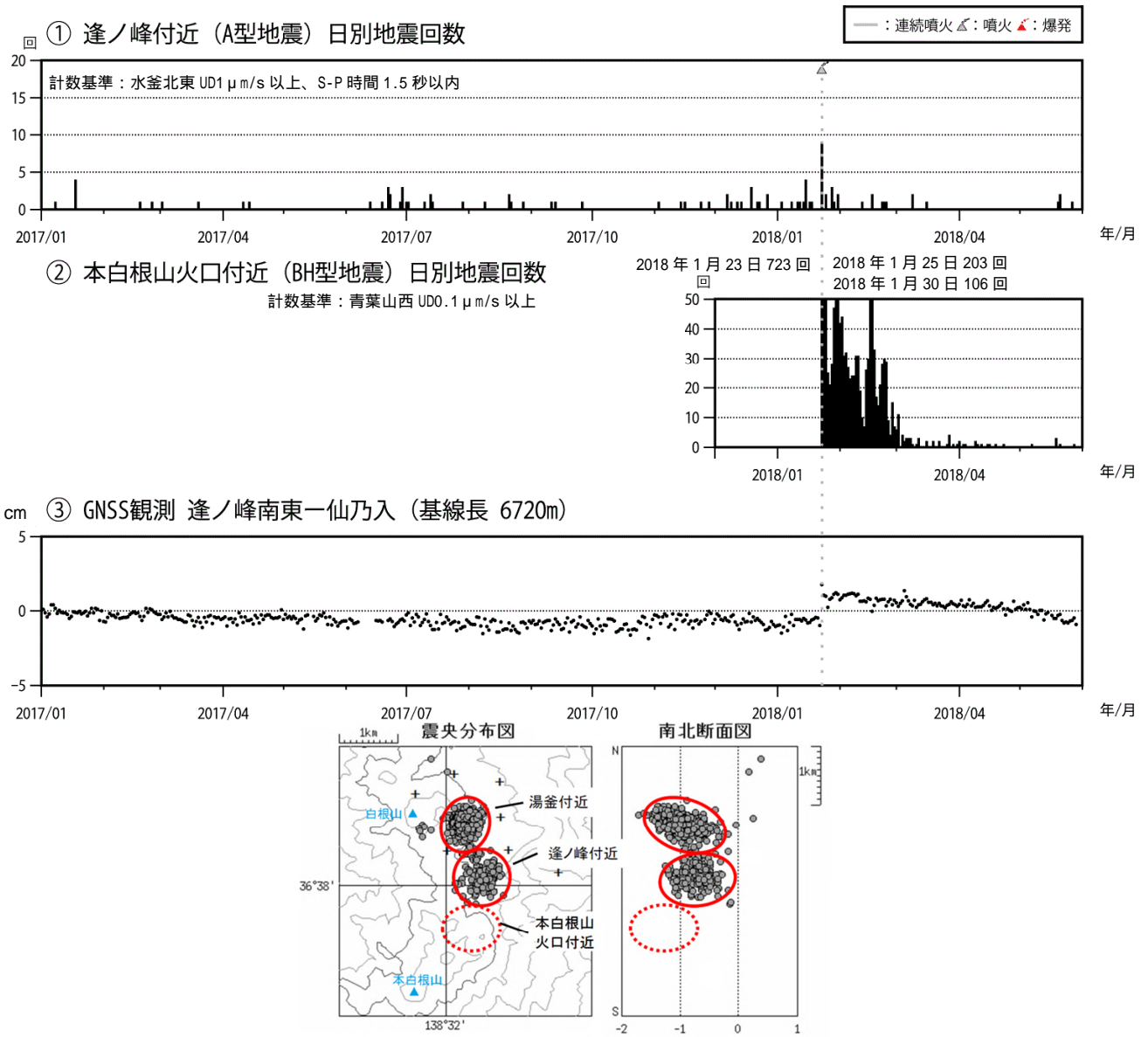
図 14 草津白根山(本白根山) 火山活動経過図(2017年1月1日~2018年5月31日) 草津白根山では、火山性地震はその発生領域から、「湯釜付近」、「逢ノ峰付近」、「本白根山火口付近」に分けています。本白根山の火山活動については、逢ノ峰付近と本白根山火口付近の地震活動に注目して監視しています。火山性地震の種類については図 16 を参照してください。
