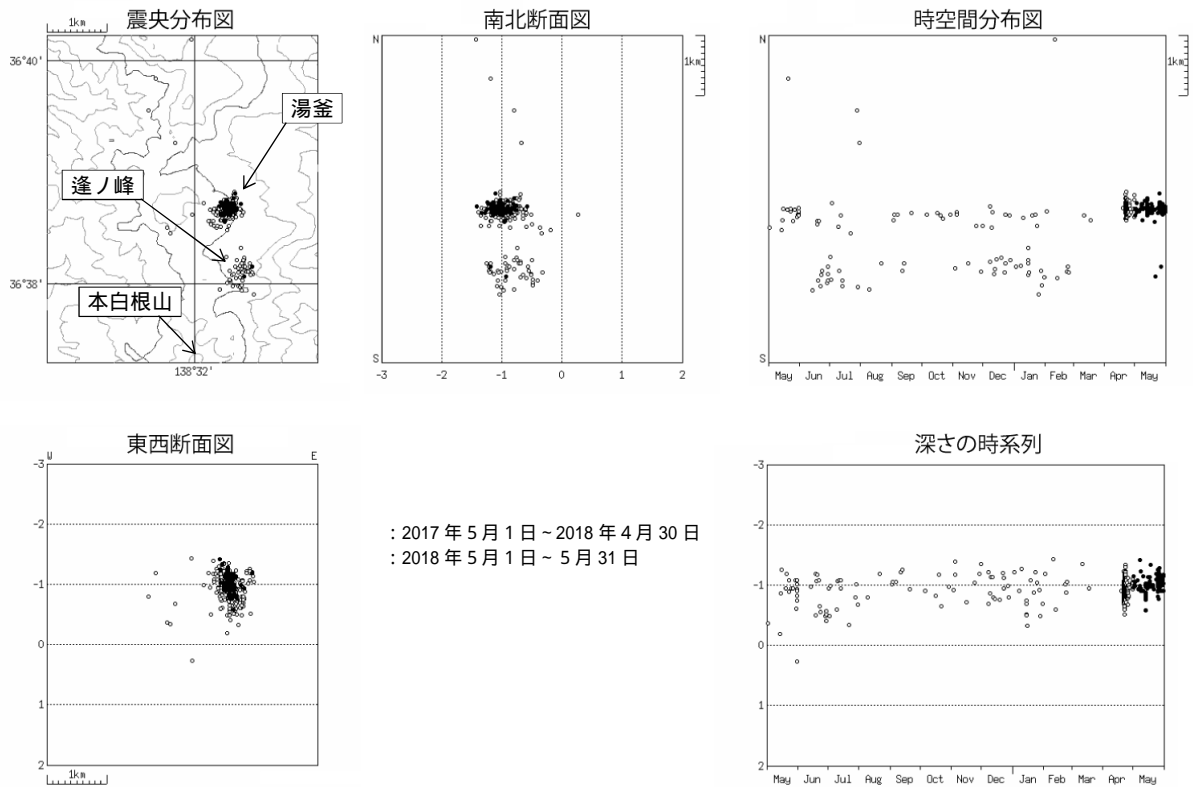
図4 草津白根山 震源分布図（2017年5月1日～2018年5月31日）
