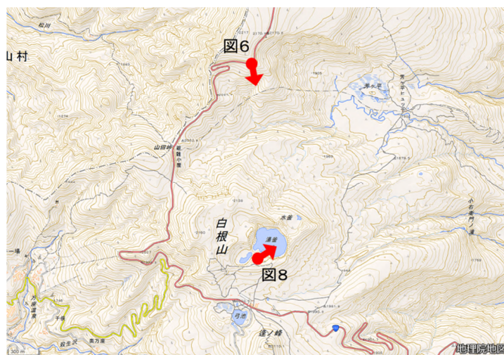
図7 草津白根山（白根山（湯釜付近）） 図6、図8の撮影場所
