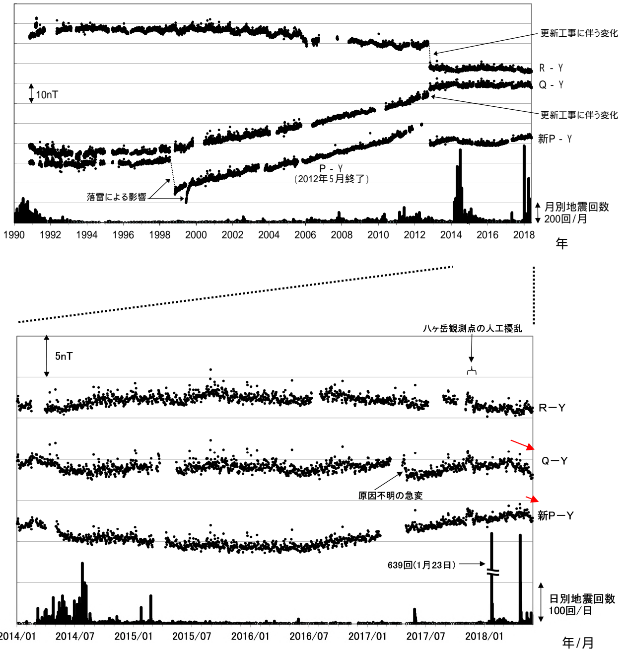
図 10 草津白根山(白根山(湯釜付近))全磁力連続観測による全磁力値の変化及び地震回数
