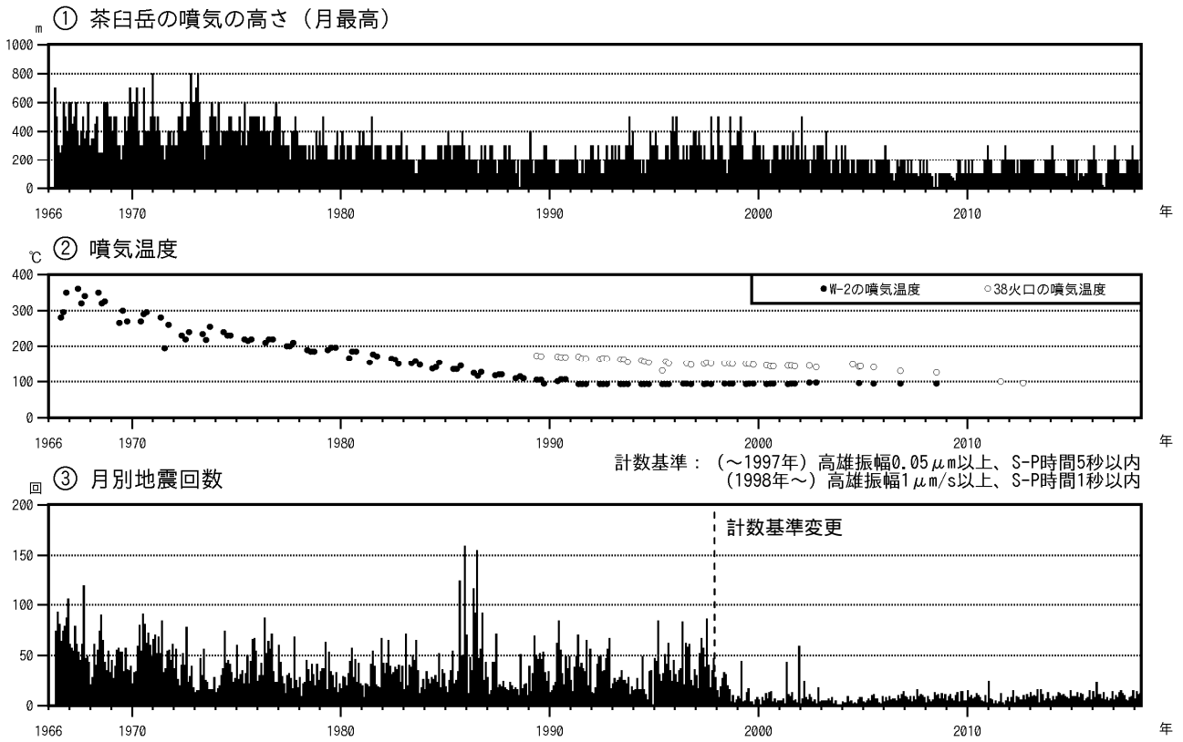
図2 那須岳 火山活動経過図(1966年1月~2018年4月)
