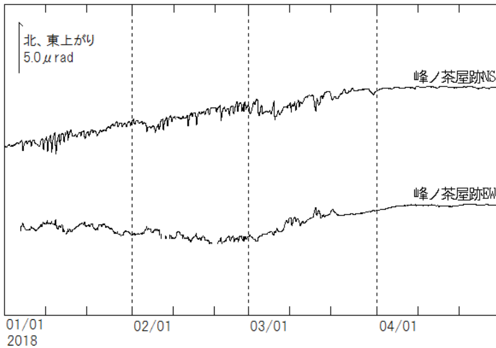
図5 那須岳 峰ノ茶屋跡観測点における傾斜データ(2018年1月1日～4月30日)
