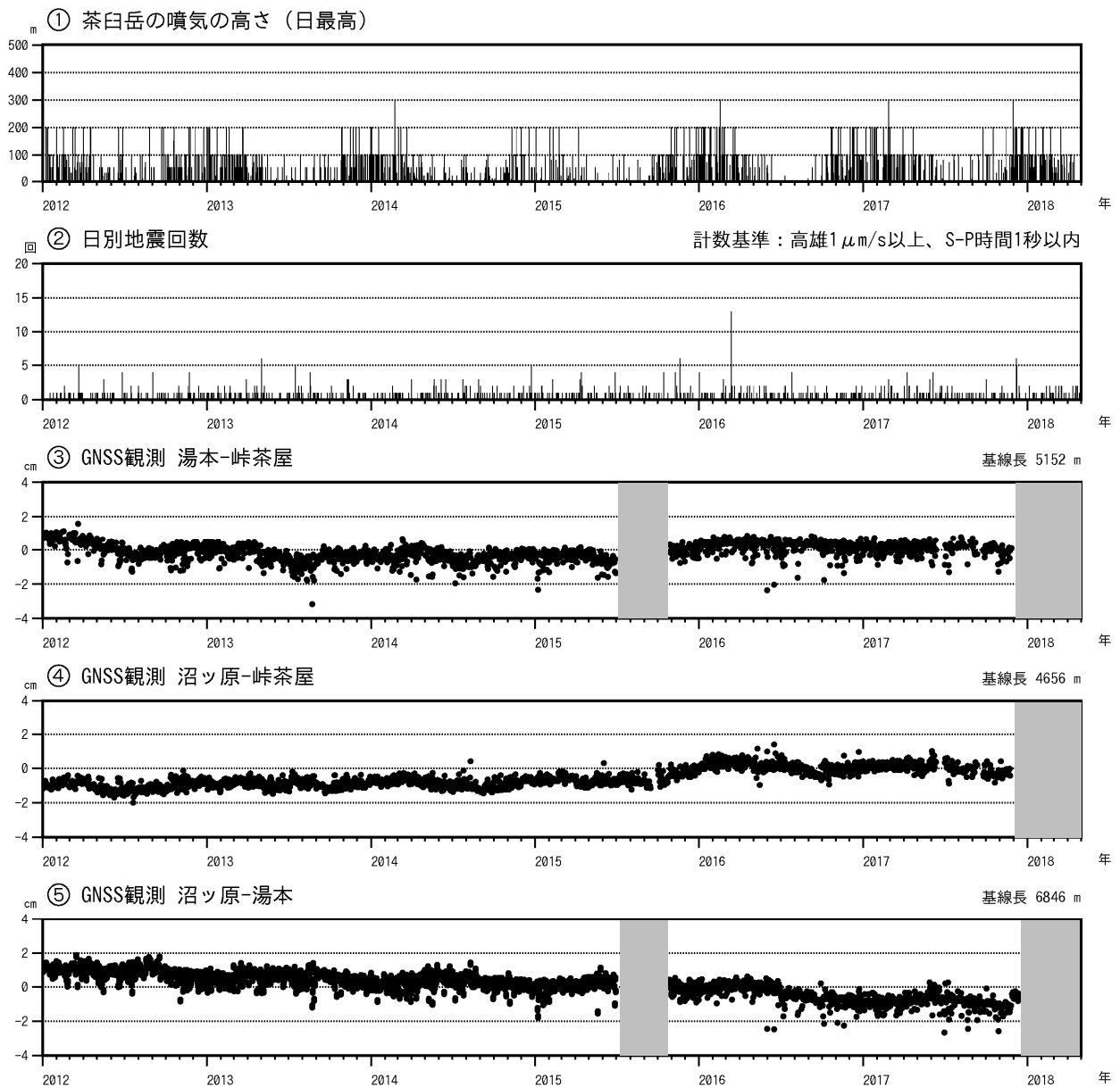
図3 那須岳 火山活動経過図（2012年1月1日～2018年4月30日）
