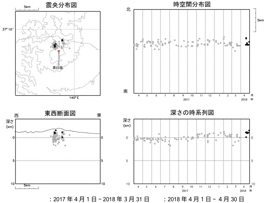
図4 那須岳 震源分布図(2017年4月1日～2018年4月30日)
